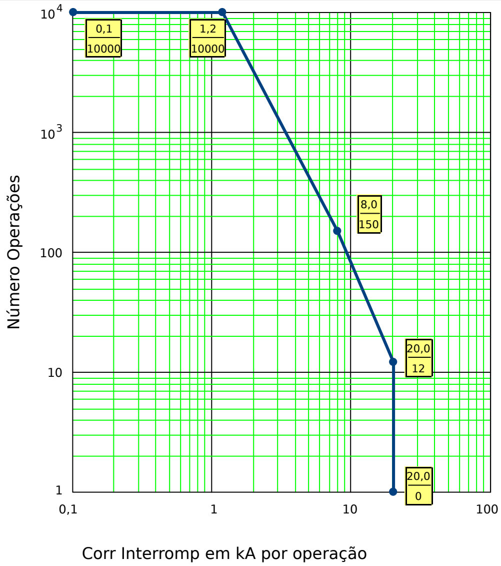
Fig. 169: Curva Manutenção de Disjuntor para Disjuntor normal 25kV
