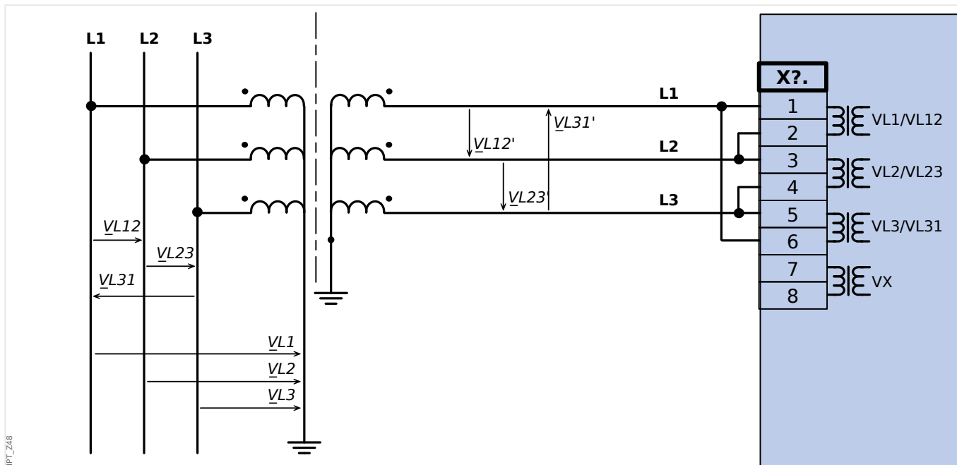
Fig. 40: Medição de tensão trifásica - fiação das entradas de medição: "conexão-delta"
