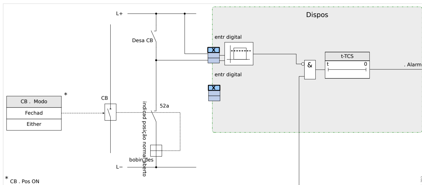
Fig. 161: Exemplo de conexão: Supervisão do circuito de disparo com apenas um contato CB auxiliar »Aux ON« (52a).
