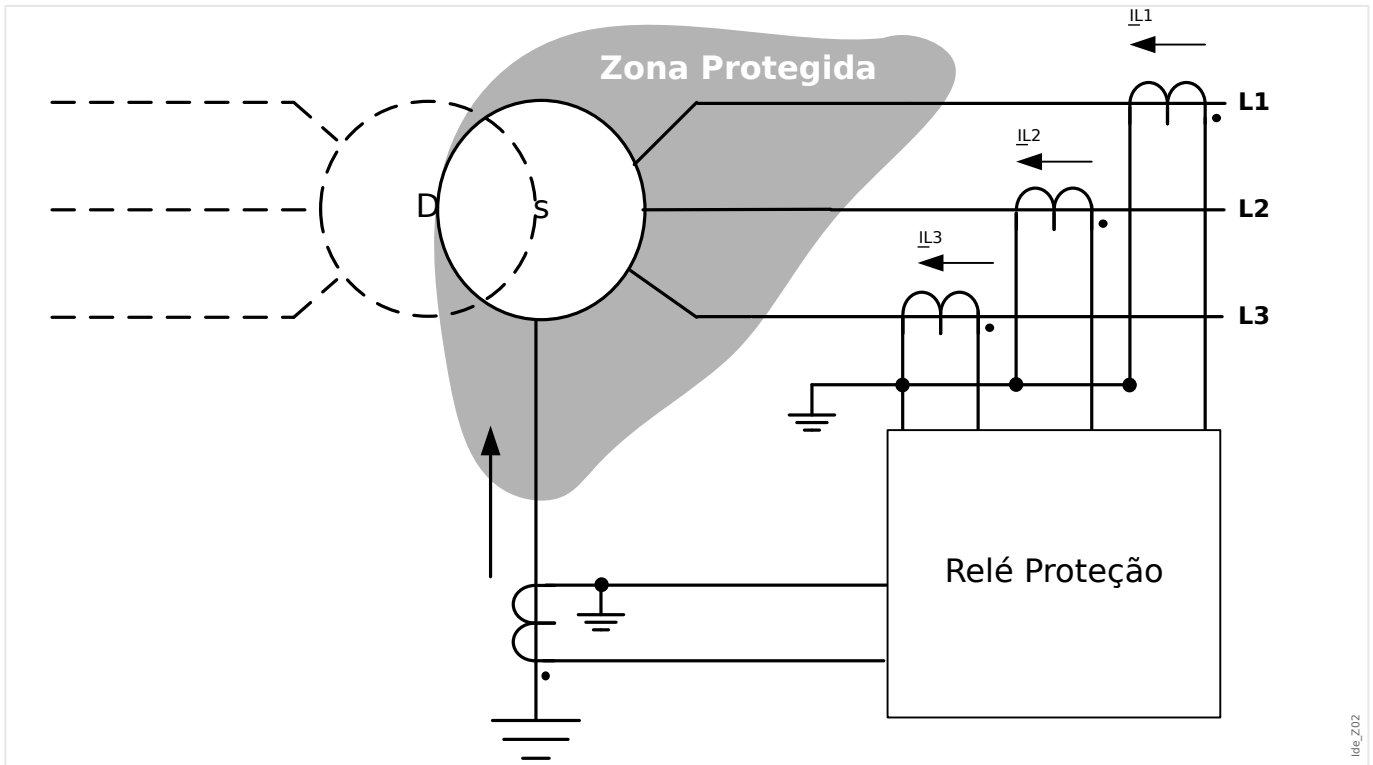
Fig. 89: Princípio de Proteção da Proteção Diferencial de Corrente de Aterramento no enrolamento lateral wye do transformador.
