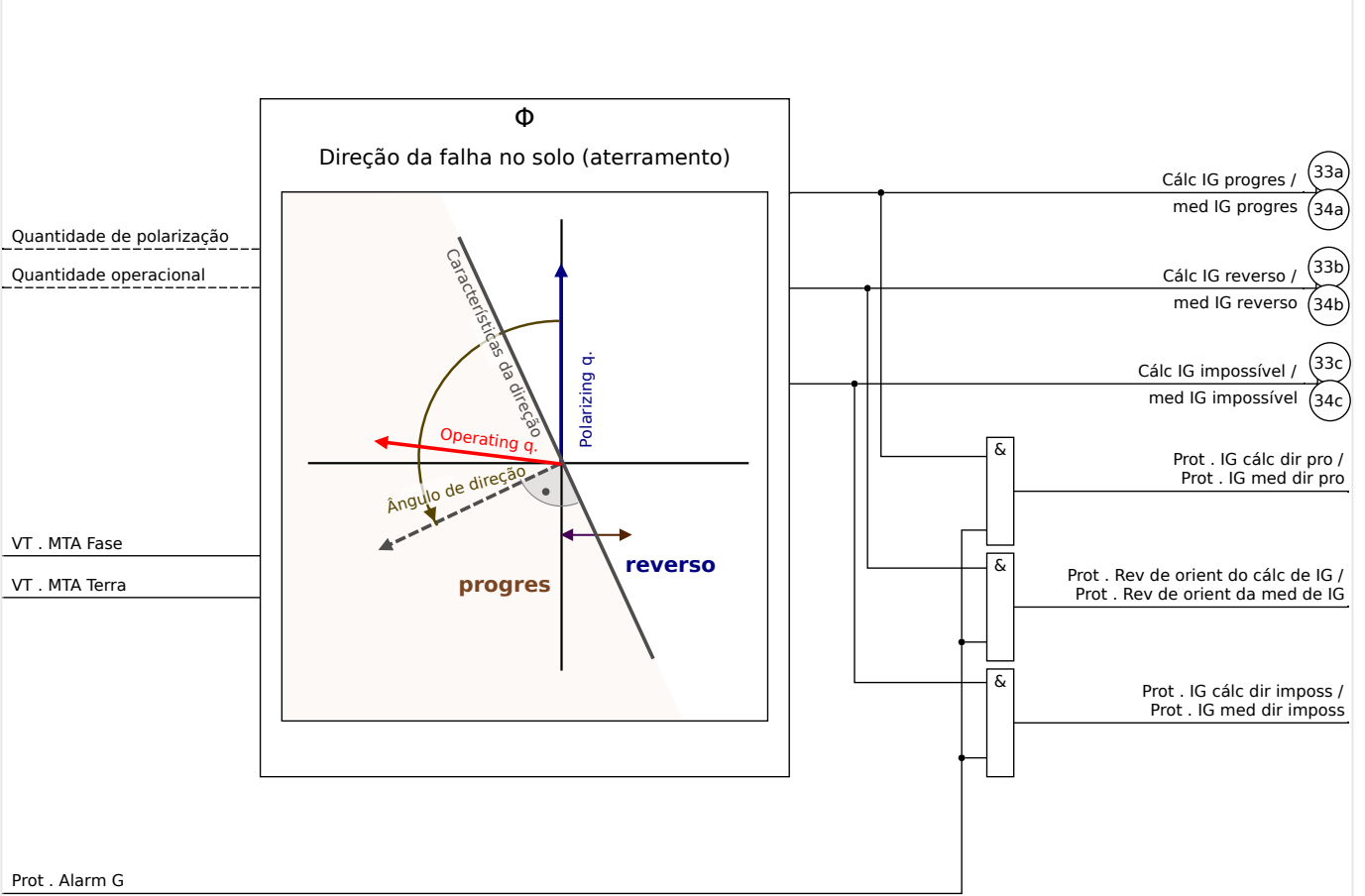
Fig. 76: Determinação da direção para todos os métodos, exceto "cos( \phi )", "sin( \phi )".
