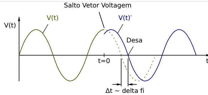
Fig. 143: Aumento de vetor de tensão.
