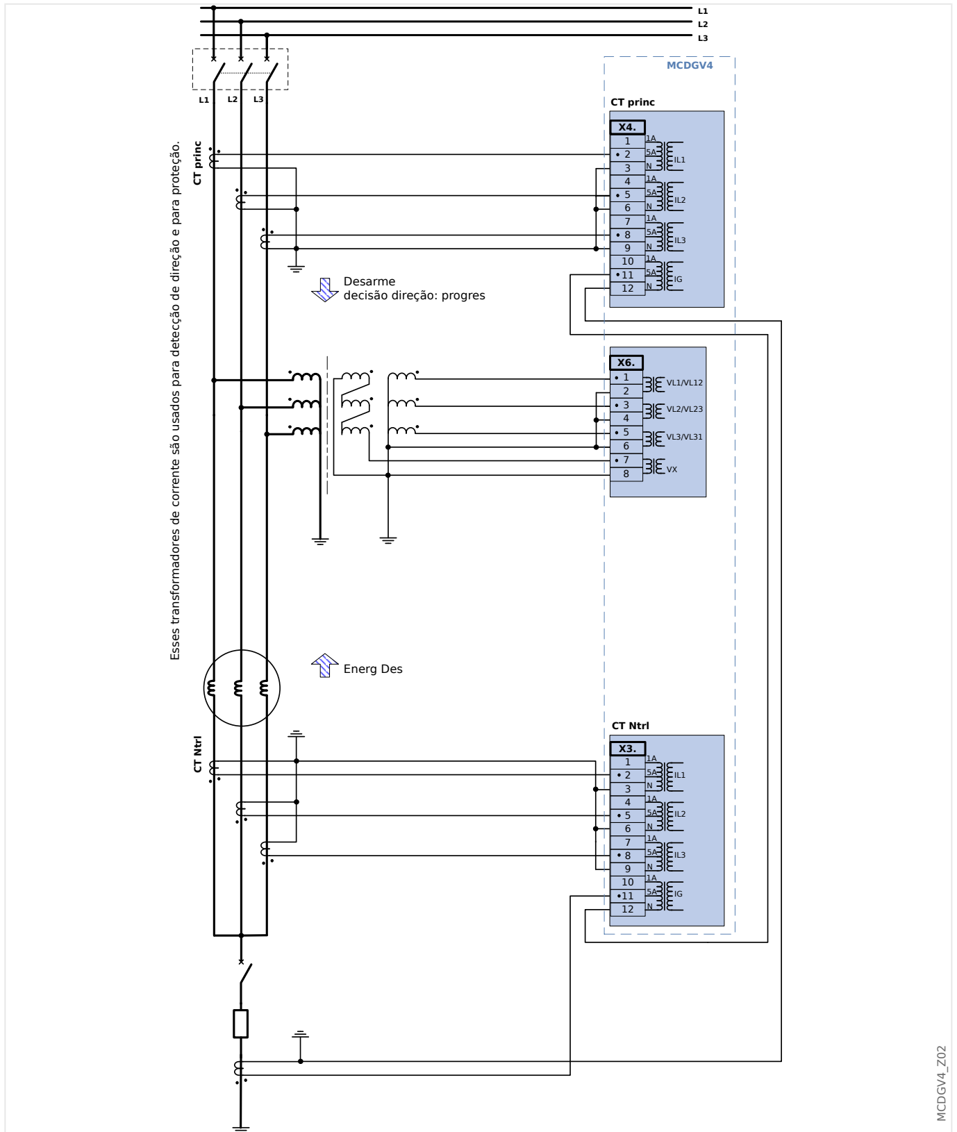
Fig. 43: Gerador Aterrado de Baixa Resistência com Proteção Diferencial de Fase e de Terra
