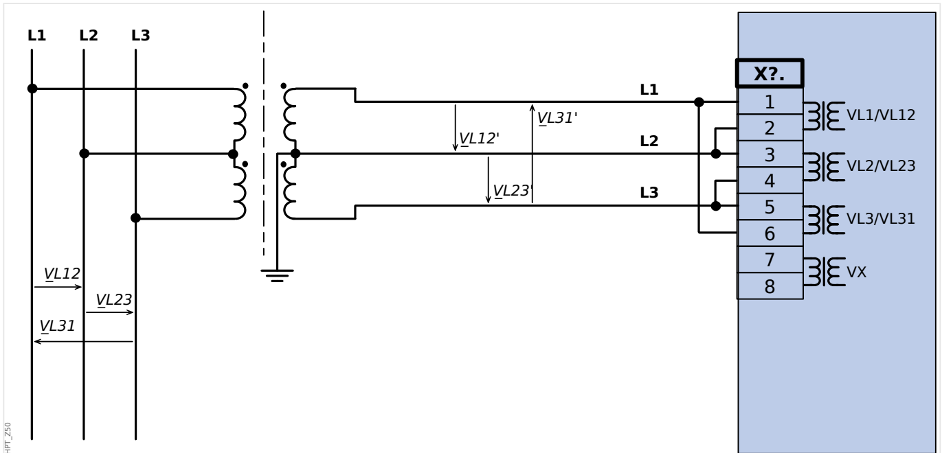
Fig. 42: Medição de voltagem bifásica - fiação das entradas de medição: "Delta Aber"
