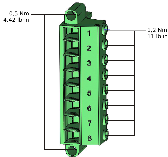
Fig. 183: Terminais de medição de tensão da placa de medição "TU" (↳ "3.8.1 TU - Entradas de Medição de Tensão").
