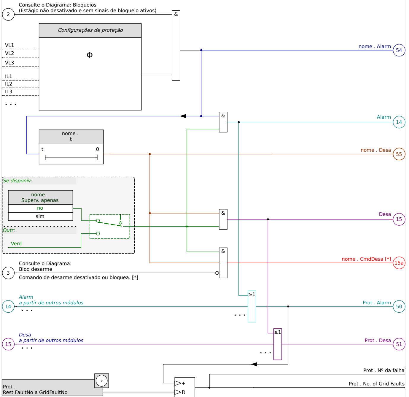
Fig. 72: Esboço rápido da funcionalidade de qualquer HighPROTEC elemento de proteção.
