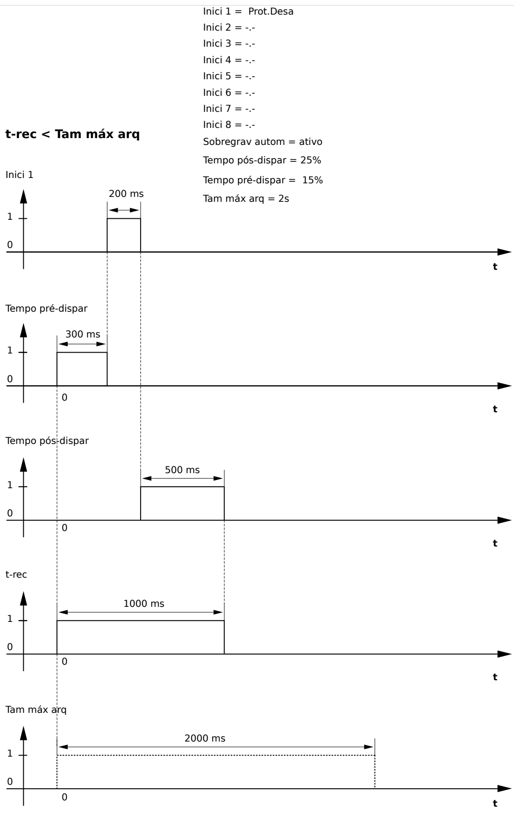
Fig. 173: Exemplo de Gráfico de Prazo do Gravador de Perturbação II
