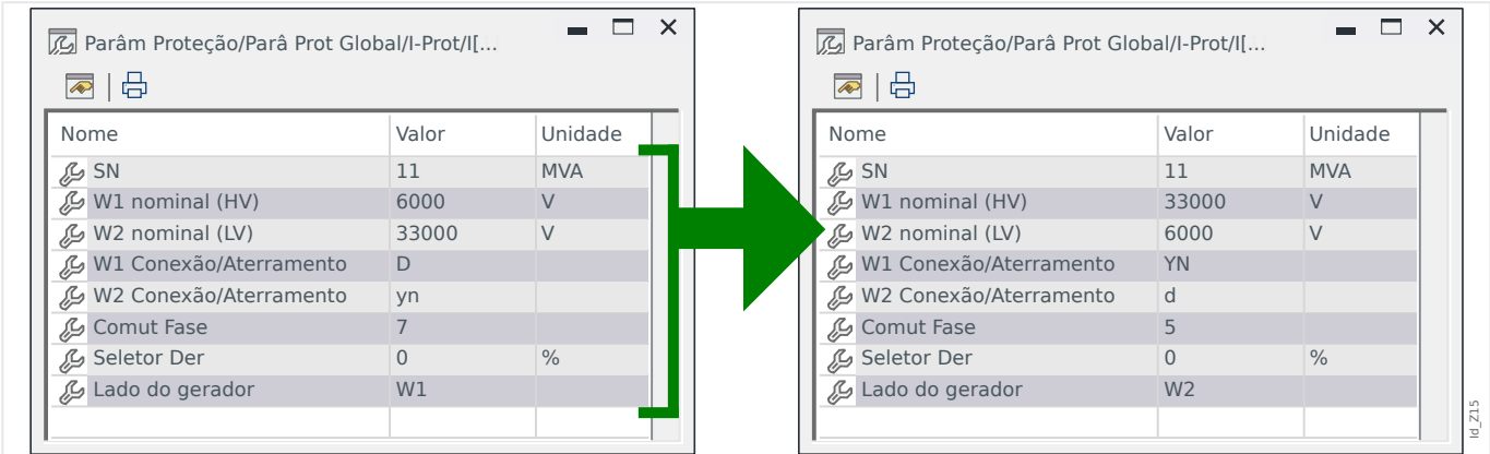
Fig. 87: Esquerda: Dados do transformador „inverso“ até a versão 3.4. Direita: Dados adaptados manualmente para versões a partir da 3.6.
