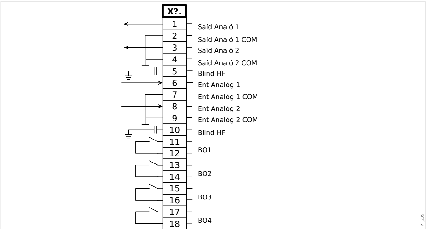
Fig. 29: Marcação de Terminal.
