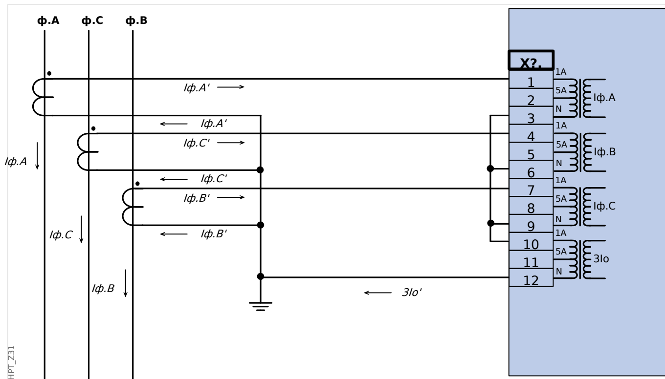
Рис. 25: Измерение фазных токов по схеме «полной» звезды; I_n вторичн. = 1 А. Ток на землю, измеряемый через соединение по схеме Холмгрена 3I_o .ном.втор. = 1 А.
