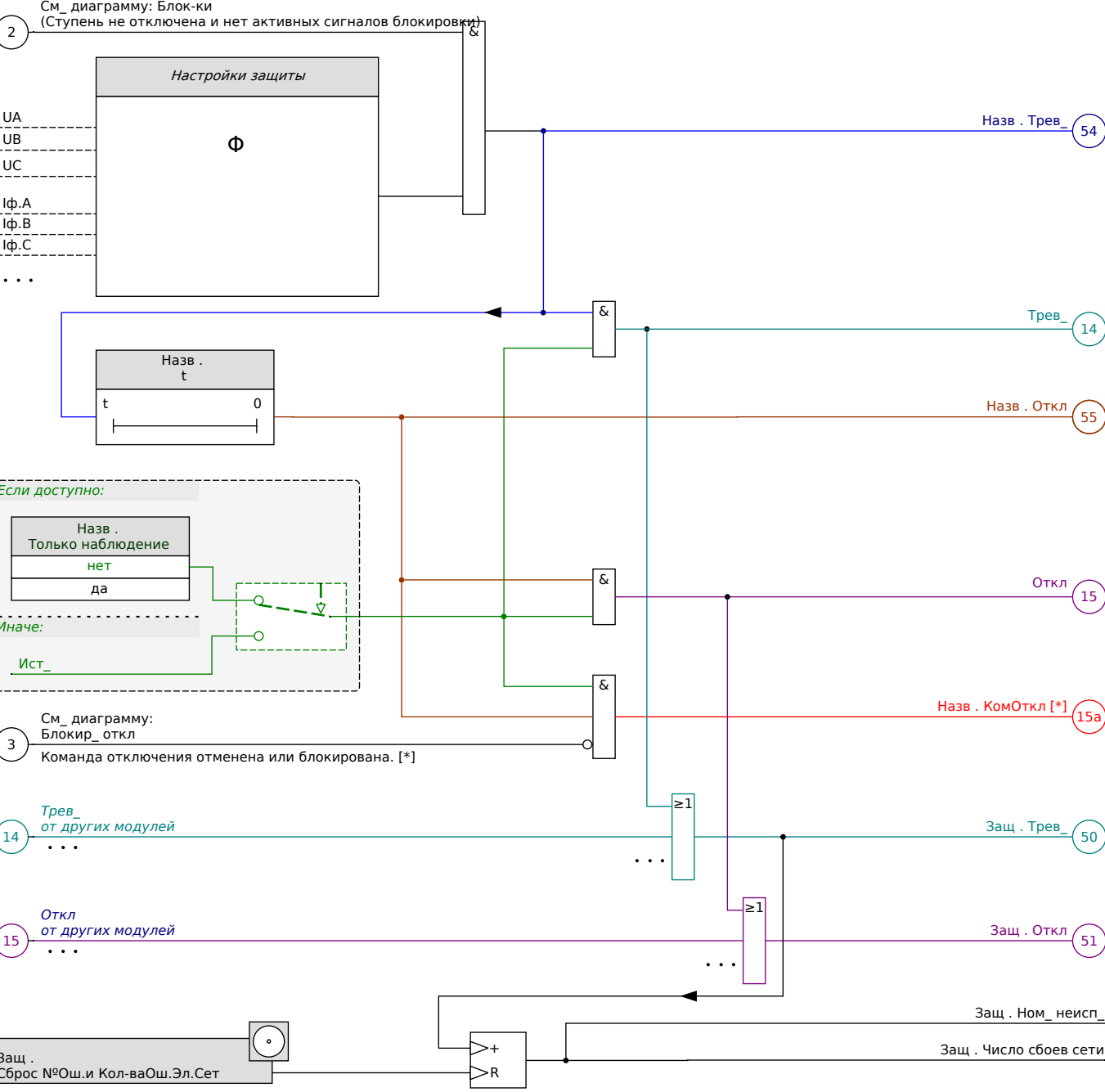
Рис. 71: Примерная схема функций любого элемента защиты HighPROTEC.
