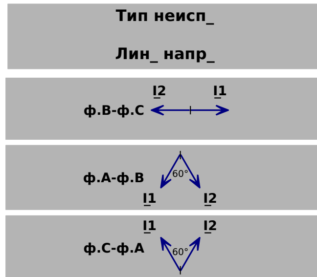
Рис. 90: Фазовые векторы токов прямой и обратной последовательности при различных типах сбоя
