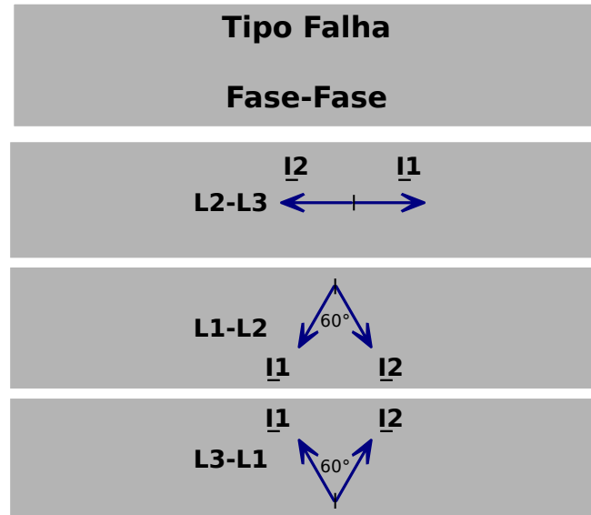
Fig. 90: Vetores de fase da corrente de sequência de fase positiva e negativa para diferentes tipos de falha.
