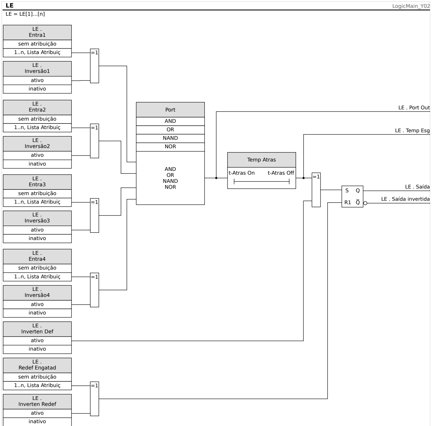
Fig. 166: Visão Geral Detalhada - Diagrama Lógico Geral.
