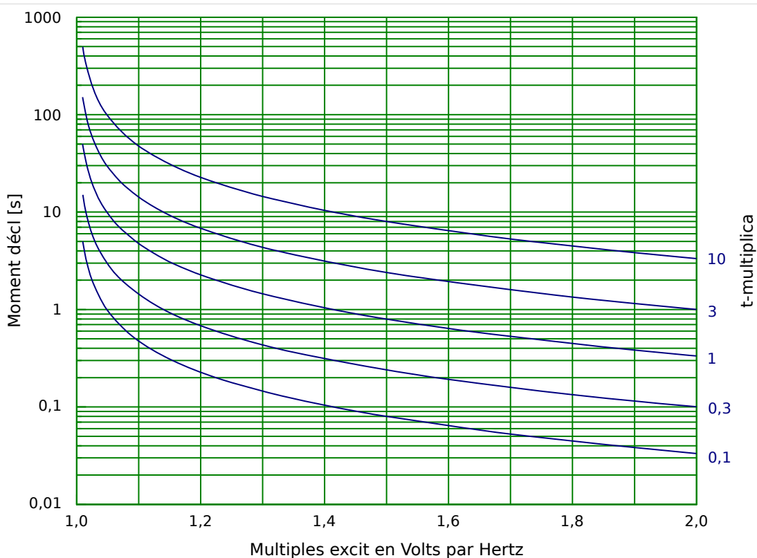
Fig. 116: Caractéristiques / forme de la courbe : INV A
