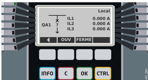
Fig. 155: Exemple de page de contrôle, avec le « disjoncteur » en position de dysfonctionnement (ou invraisemblable).
