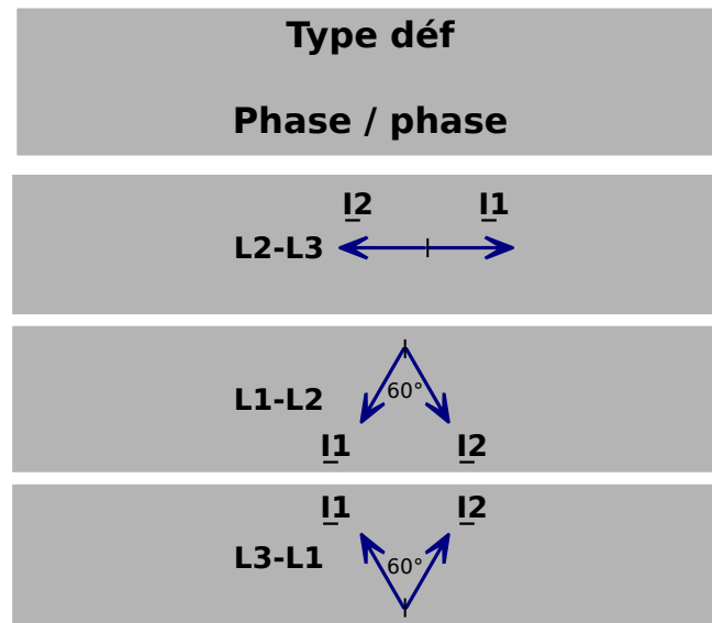
Fig. 90: Phaseurs de courant de séquence de phase positive et négative pour les différents types de défaut.
