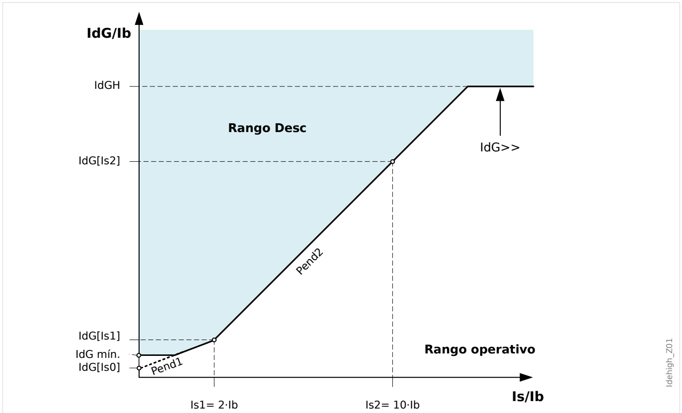
Fig. 88: Valor de selección I_dG >> de la corriente de diferencial de tierra basada en la corriente nominal I_b del objeto de protección relacionado.
