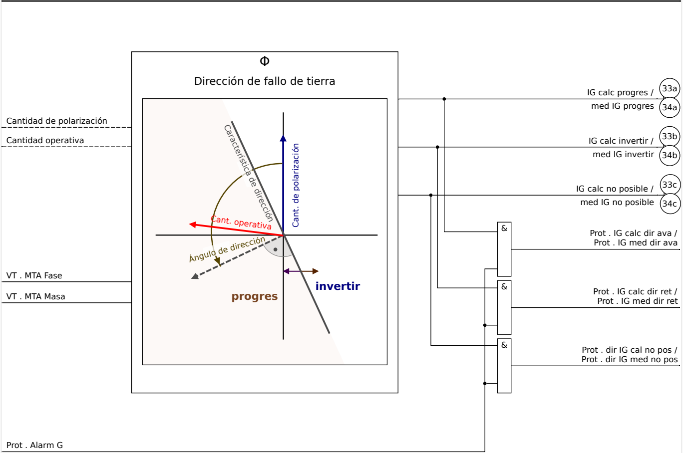
Fig. 75: Detección de dirección en todos los métodos, excepto "cos( \phi )", "sin( \phi )".
