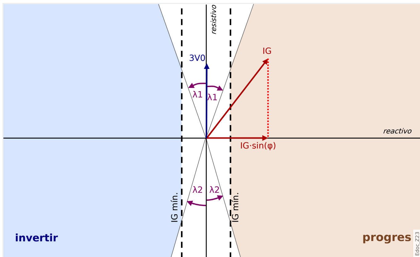
Fig. 77: Principio para determinar la dirección en el método "sin(φ)".
