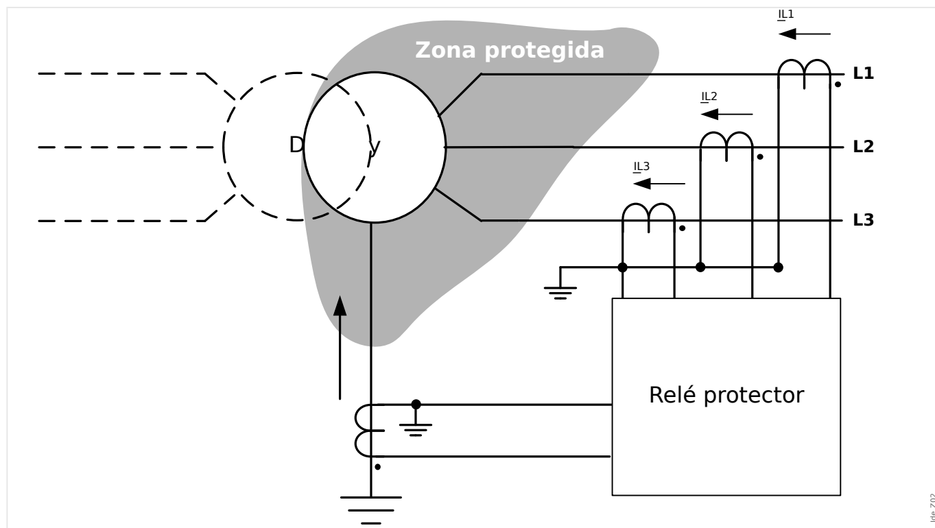
Fig. 87: Principio de protección de la protección de diferencial de corriente de tierra conectada al bobinado del lado wye del transformador
