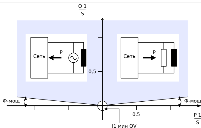
Рис. 140: Метод 1: контроль угла мощности.
