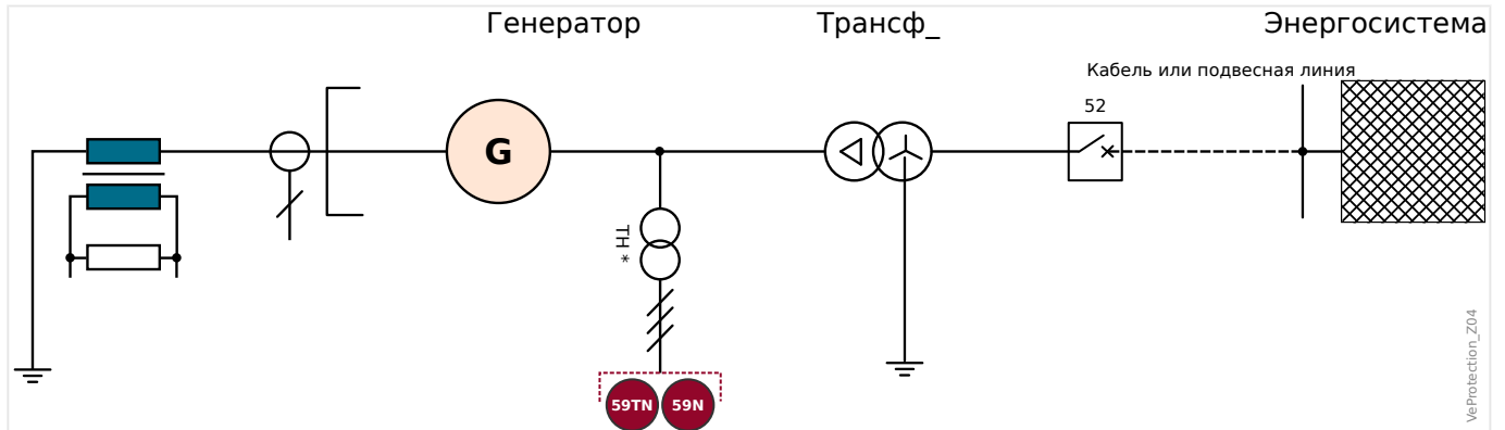
Рис. 128: Абсолютная защита статора от замыкания на землю, обеспеченная сочетанием функций ANSI 59TN/59N.
