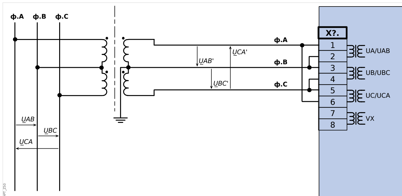
Рис. 42: Измерение двухфазного напряжения - электрическая схема измерительных входов: «соединение открытым треугольником»
