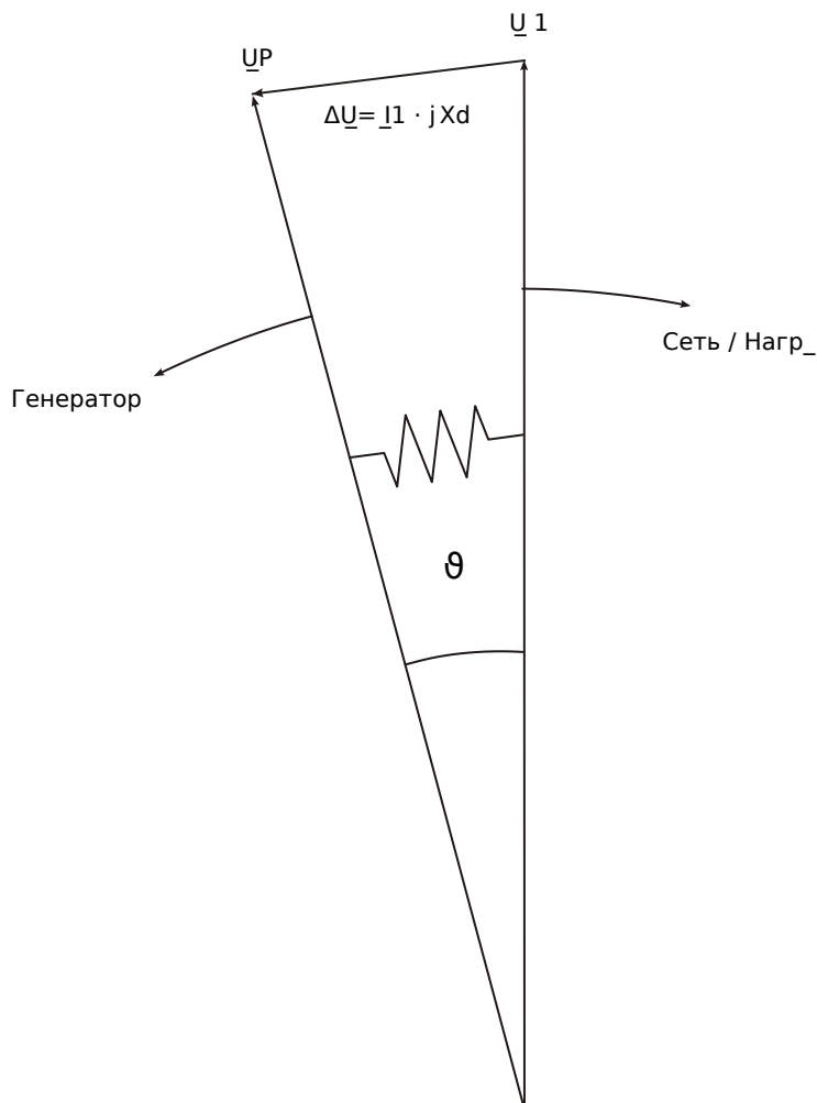
Рис. 130: Векторы напряжения в параллельной работе с электросетью.
