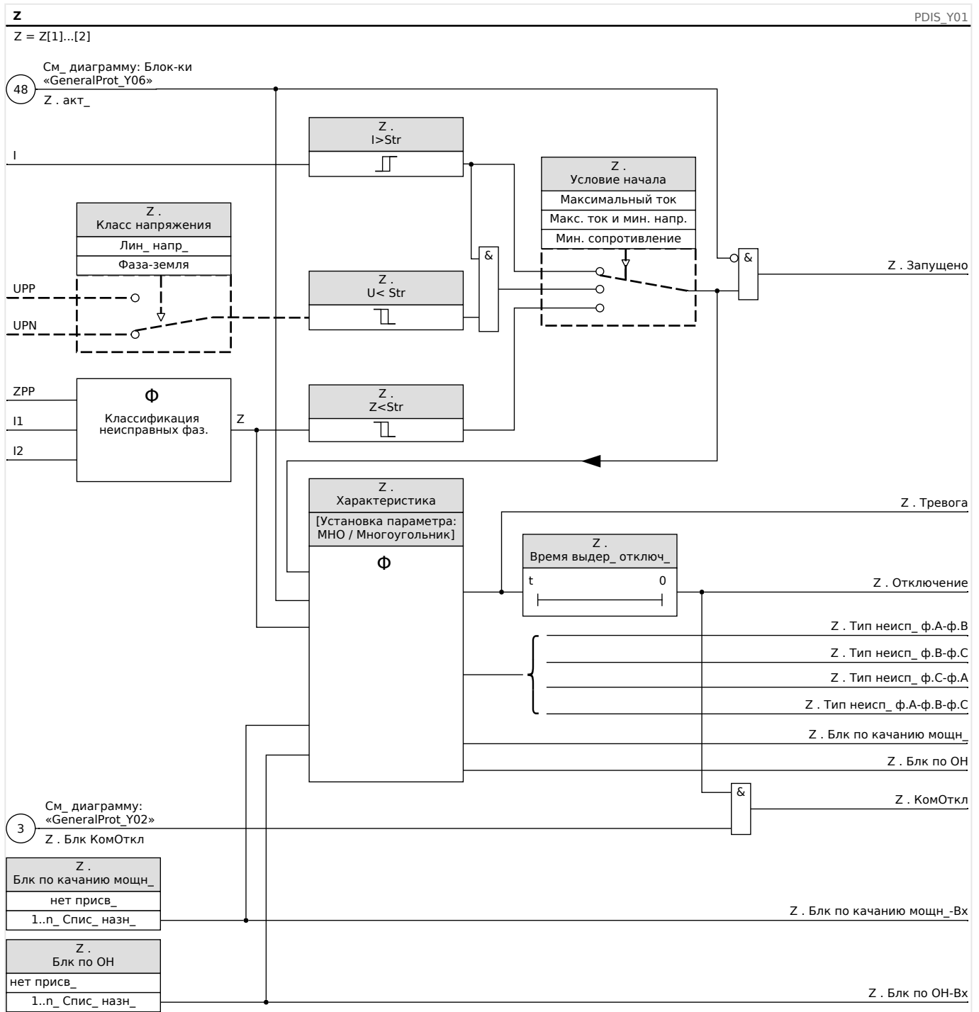
Рис. 97: Принцип работы модуля Z.
