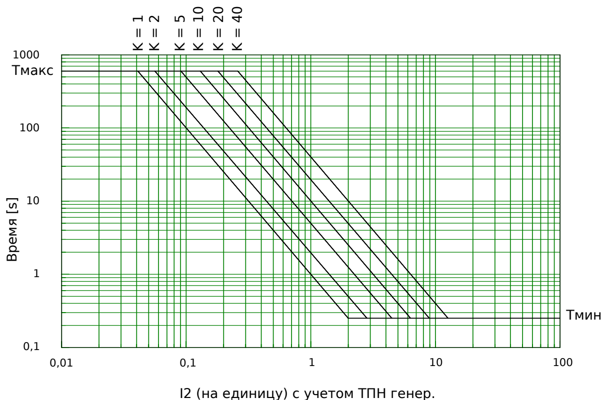
Рис. 113: Кривые отключения вследствие несимметрии генератора.
