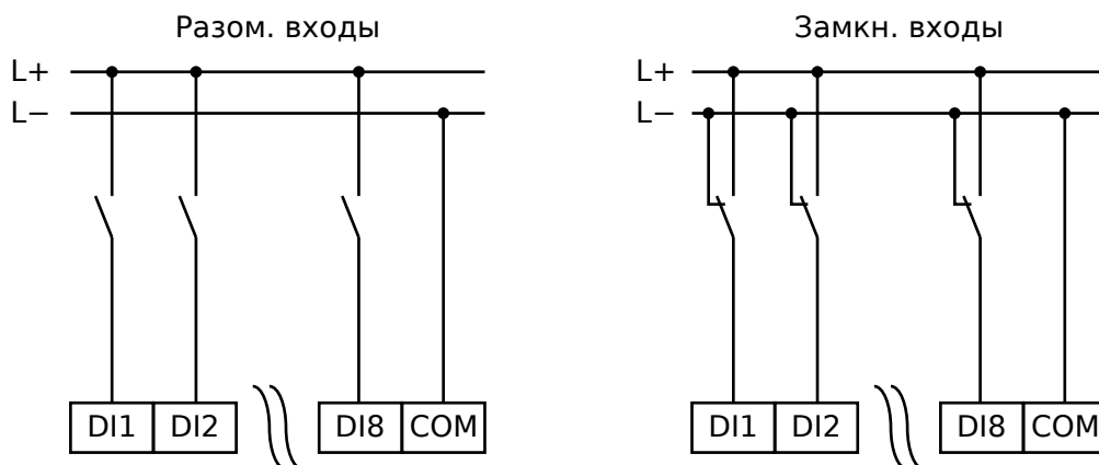
Рис. 177: Безопасное состояние цифровых входов
