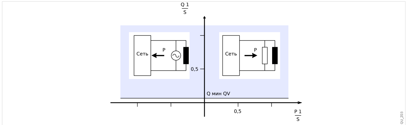
Рис. 141: Метод 2: контроль чистой реактивной мощности.
