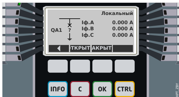
Рис. 155: Пример страницы управления, выключатель в аварийном (недопустимое состояние) положении.
