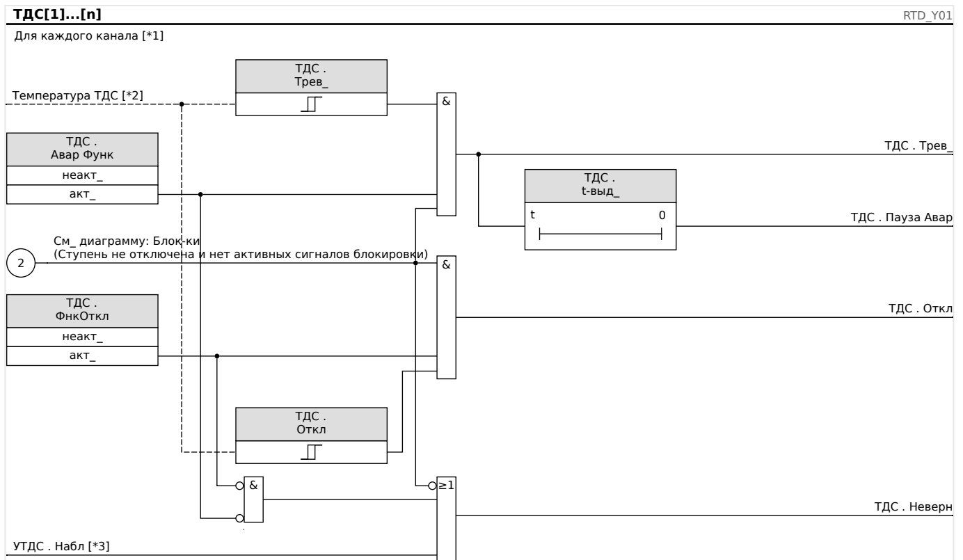
Рис. 148: Общий принцип работы (аварийный сигнал с задержкой, отключение без задержки).
