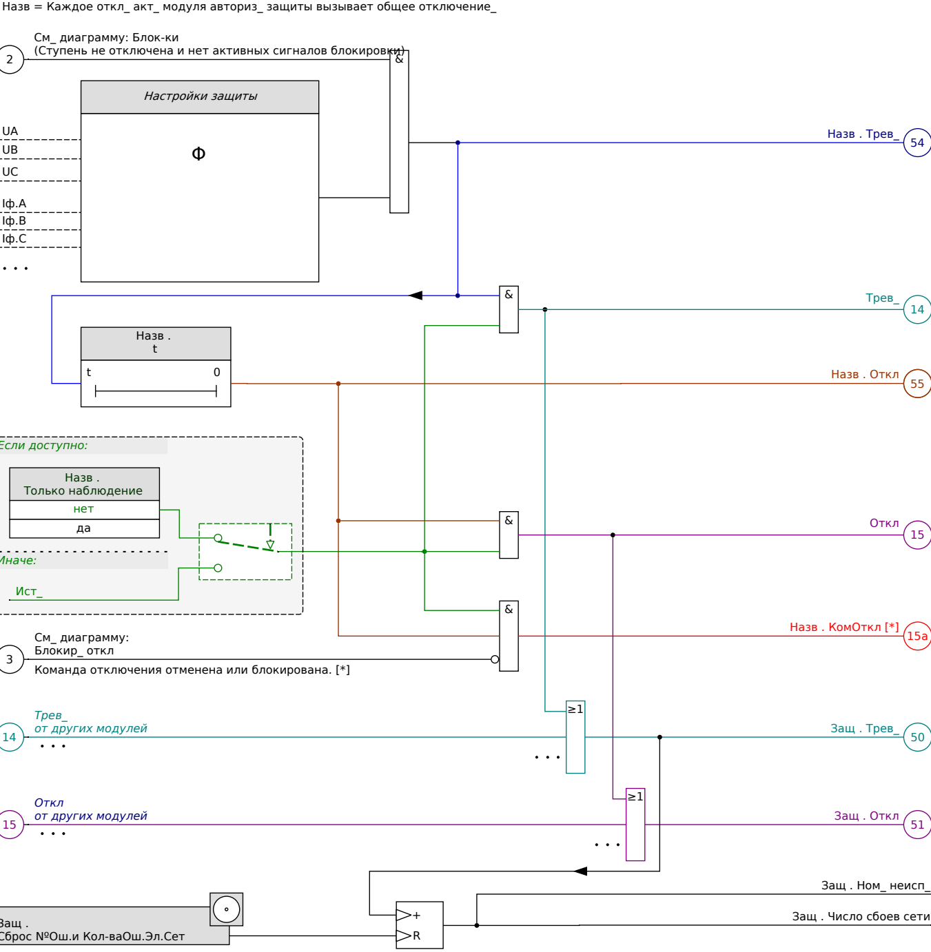
Рис. 71: Примерная схема функций любого элемента защиты HighPROTEC.
