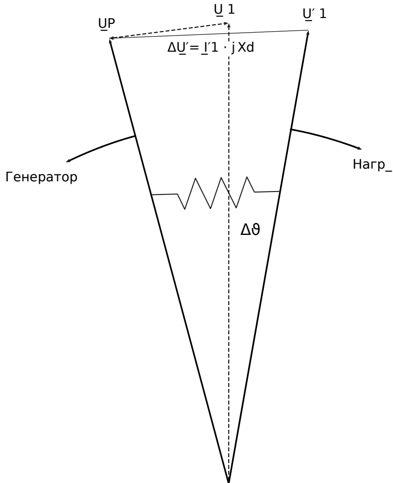
Рис. 132: Векторы напряжения при сбое электросети.
