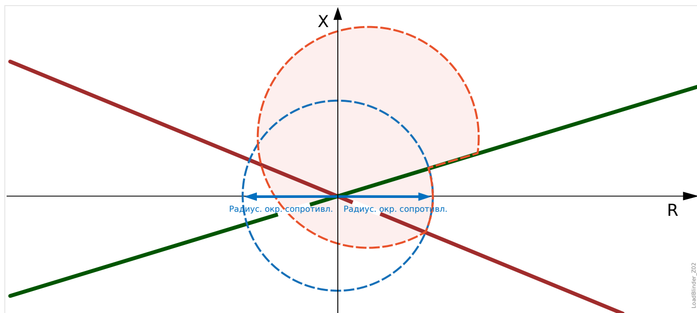
Рис. 109: Зона отключения дистанционной защиты (область, выделенная красным) с активным ограничителем нагрузки.
