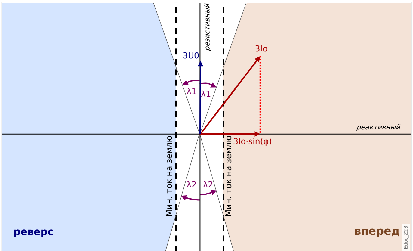
Рис. 77: Принцип определения направления для метода « \sin(\phi) ».
