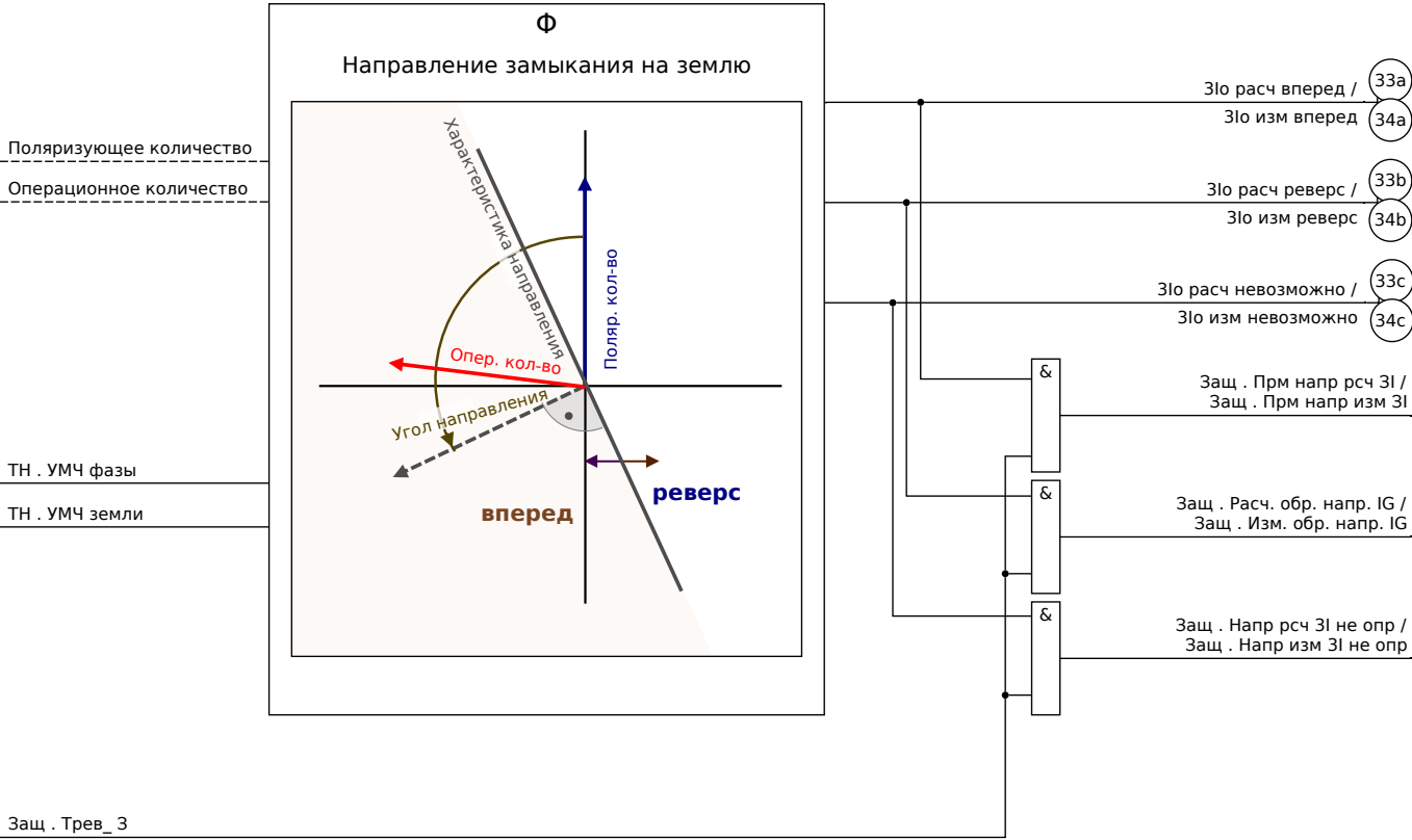
Рис. 75: Определение направления для всех методов, кроме « \cos(\phi) » и « \sin(\phi) ».
