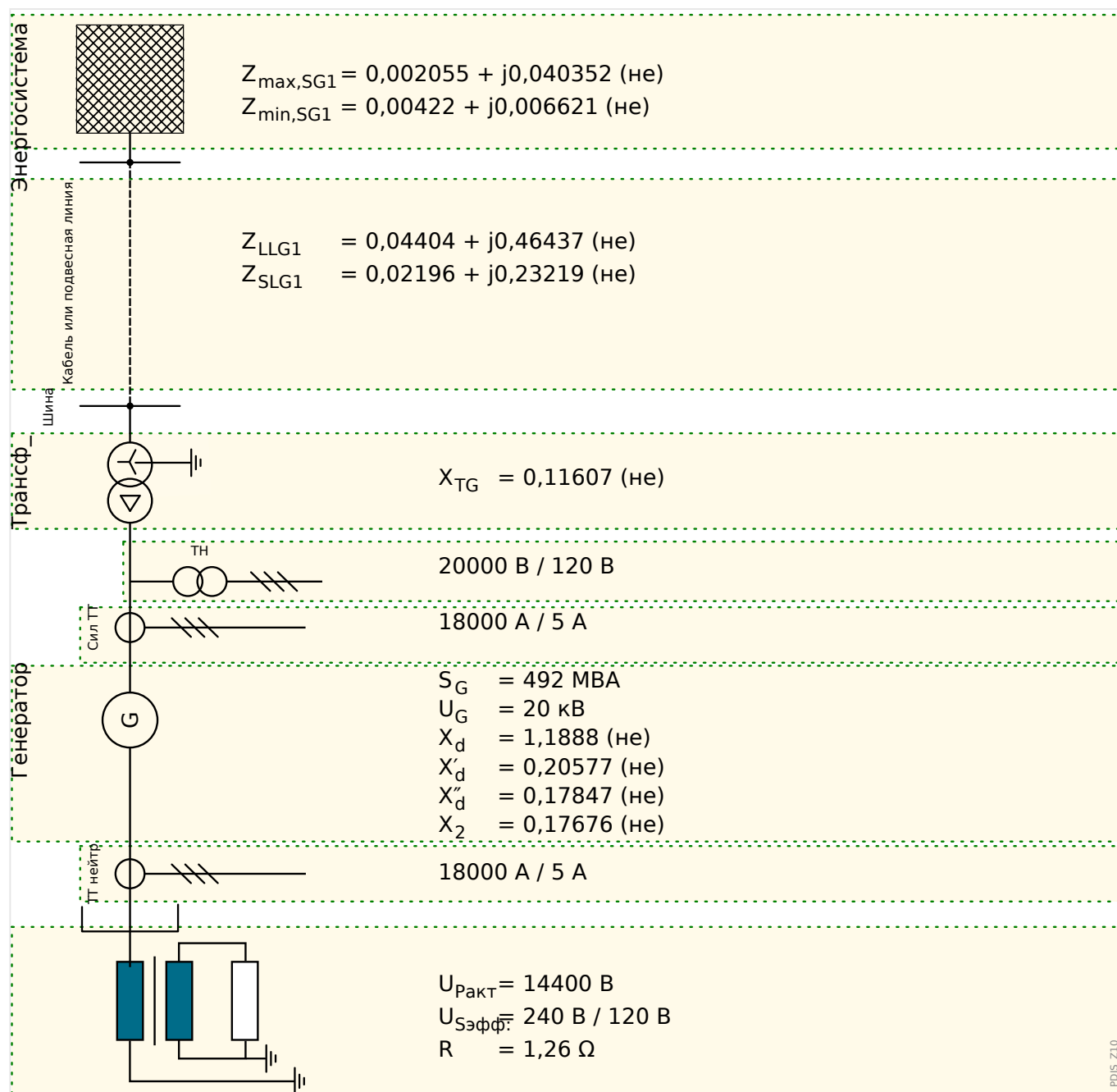
Рис. 99: Однолинейная схема с данными генератора
