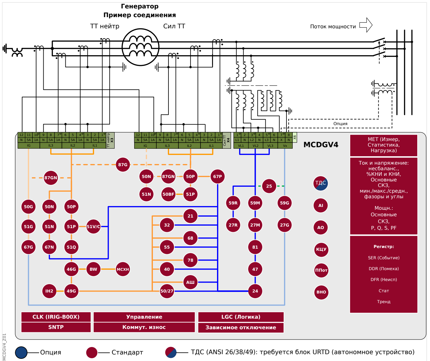
Рис. 1: Обзор функций MCDGV4.
