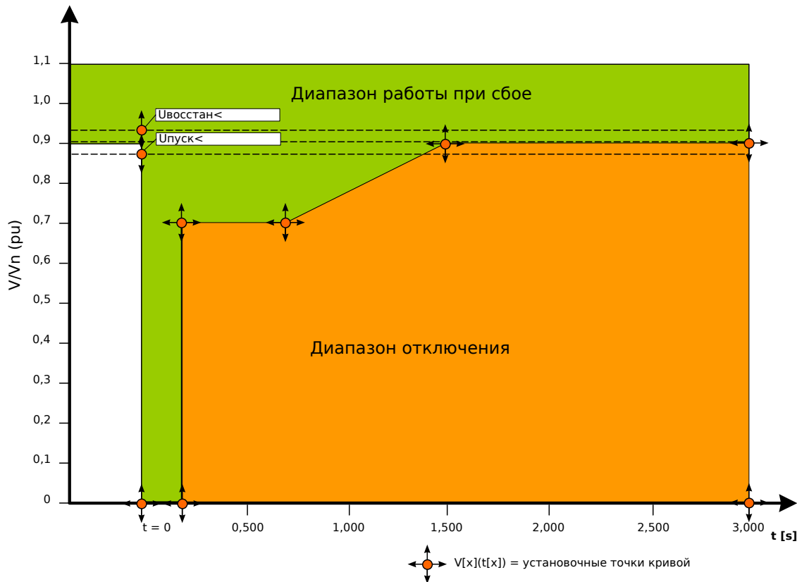
Рис. 144: Область продолжения работы и область отключения.
