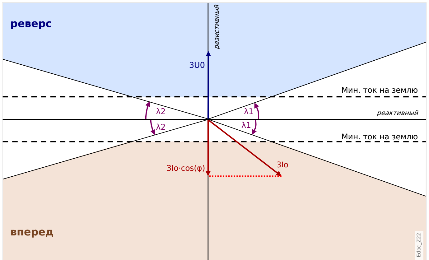
Рис. 76: Принцип определения направления для метода « \cos(\phi) ».
