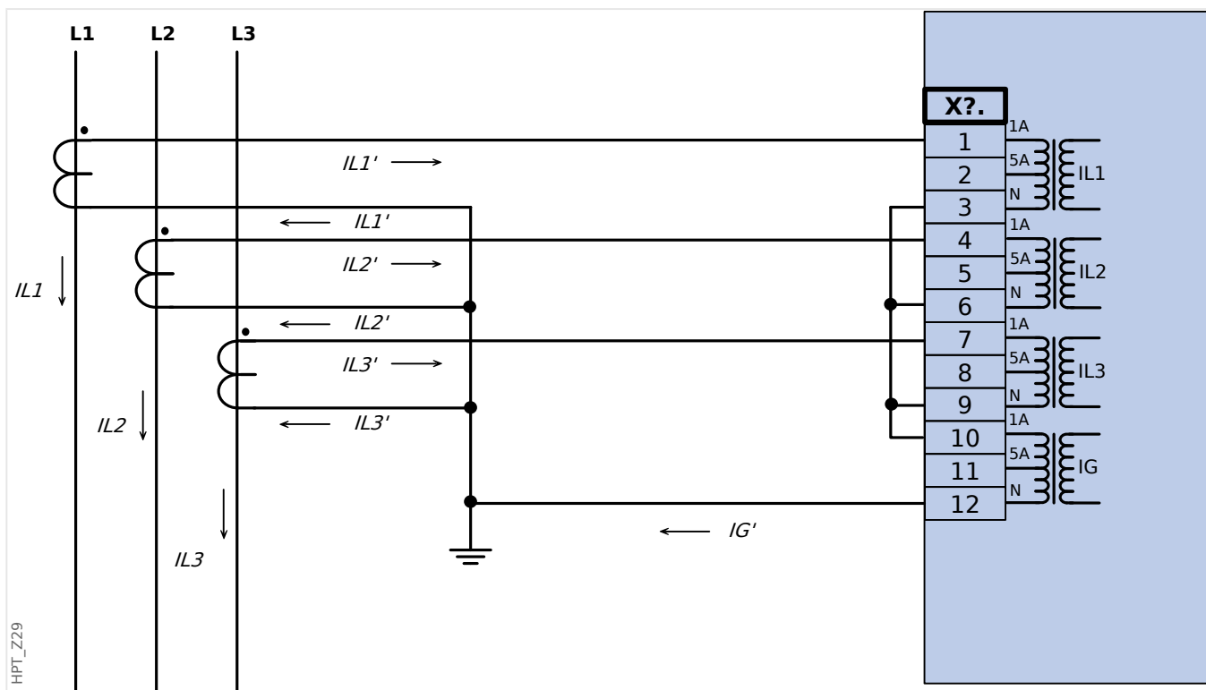
Fig. 23: Medição de corrente de trifásica; I_n secundário = 1 A. Medição corrente terra via conexão Holmgreen; IG_{nom} secundário = 1 A.
