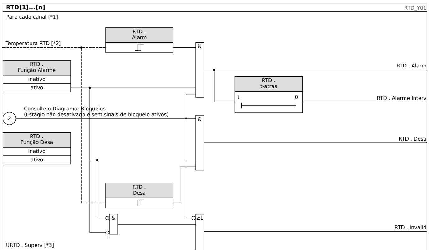
Fig. 148: O princípio geral de funcionamento (alarme atrasado, disparo sem atraso).
