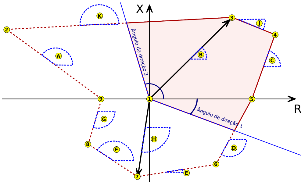
Fig. 95: Área operacional (colorida em vermelho brilhante) do tipo polígono, com »Ativação de direção« = "ativo".
