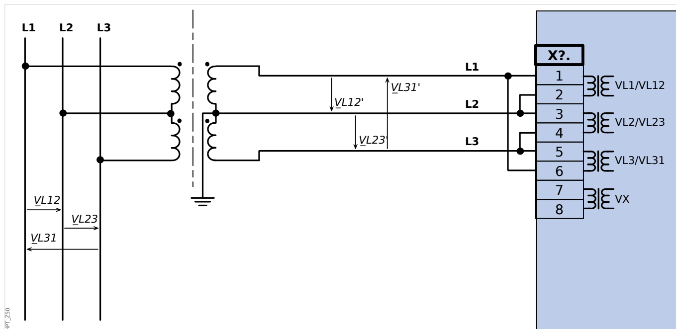
Fig. 42: Medição de voltagem bifásica - fiação das entradas de medição: "Delta Aber"
