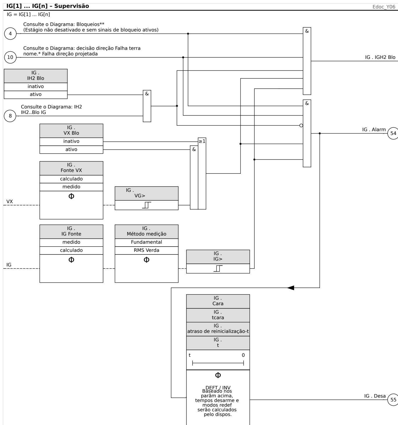
Fig. 111: Proteção de sobrecorrente de solo (aterramento), parte 1 (função de supervisão, decisão de disparo).
