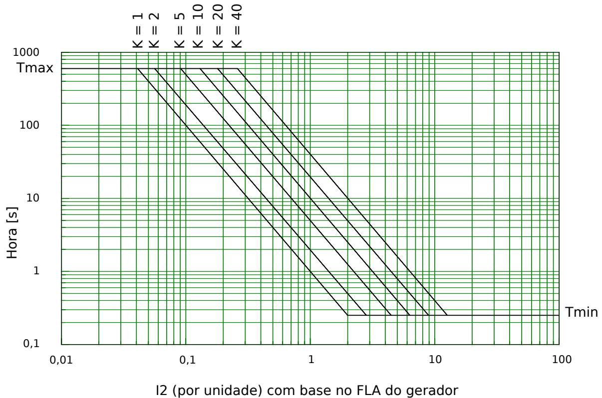
Fig. 113: Curvas de disparo de desequilíbrio do gerador.
