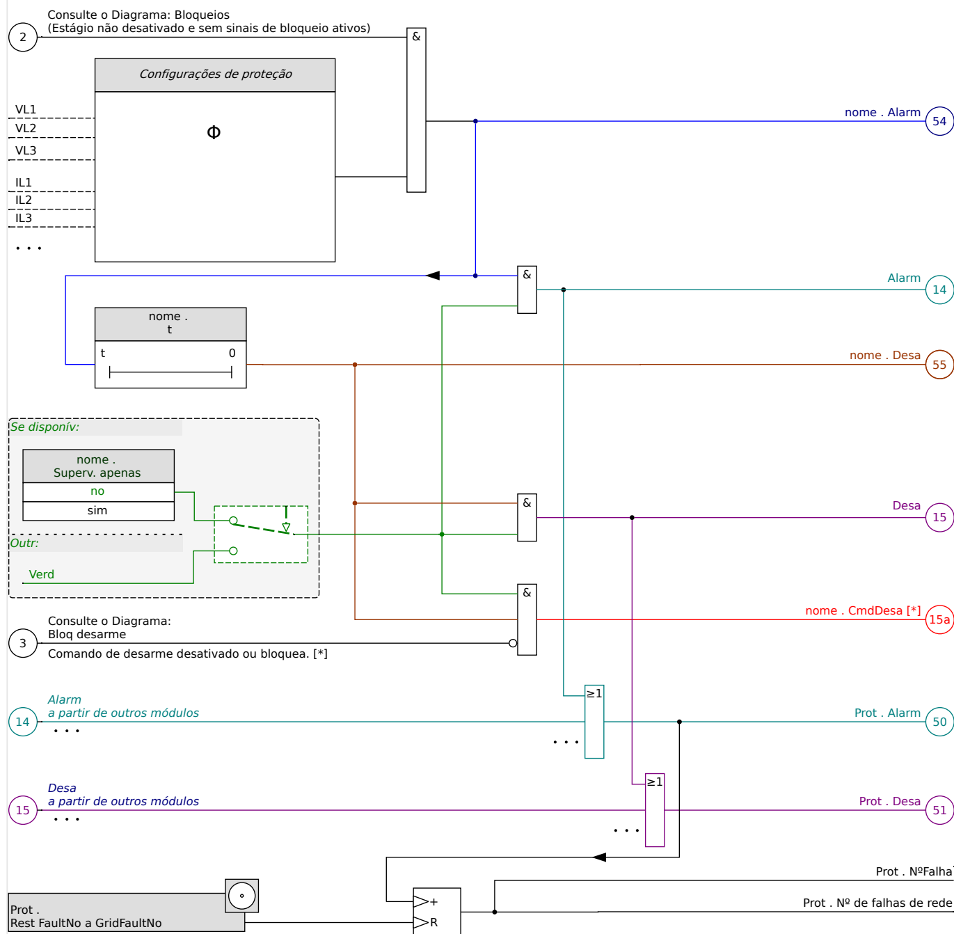
Fig. 71: Esboço rápido da funcionalidade de qualquer HighPROTEC elemento de proteção.
