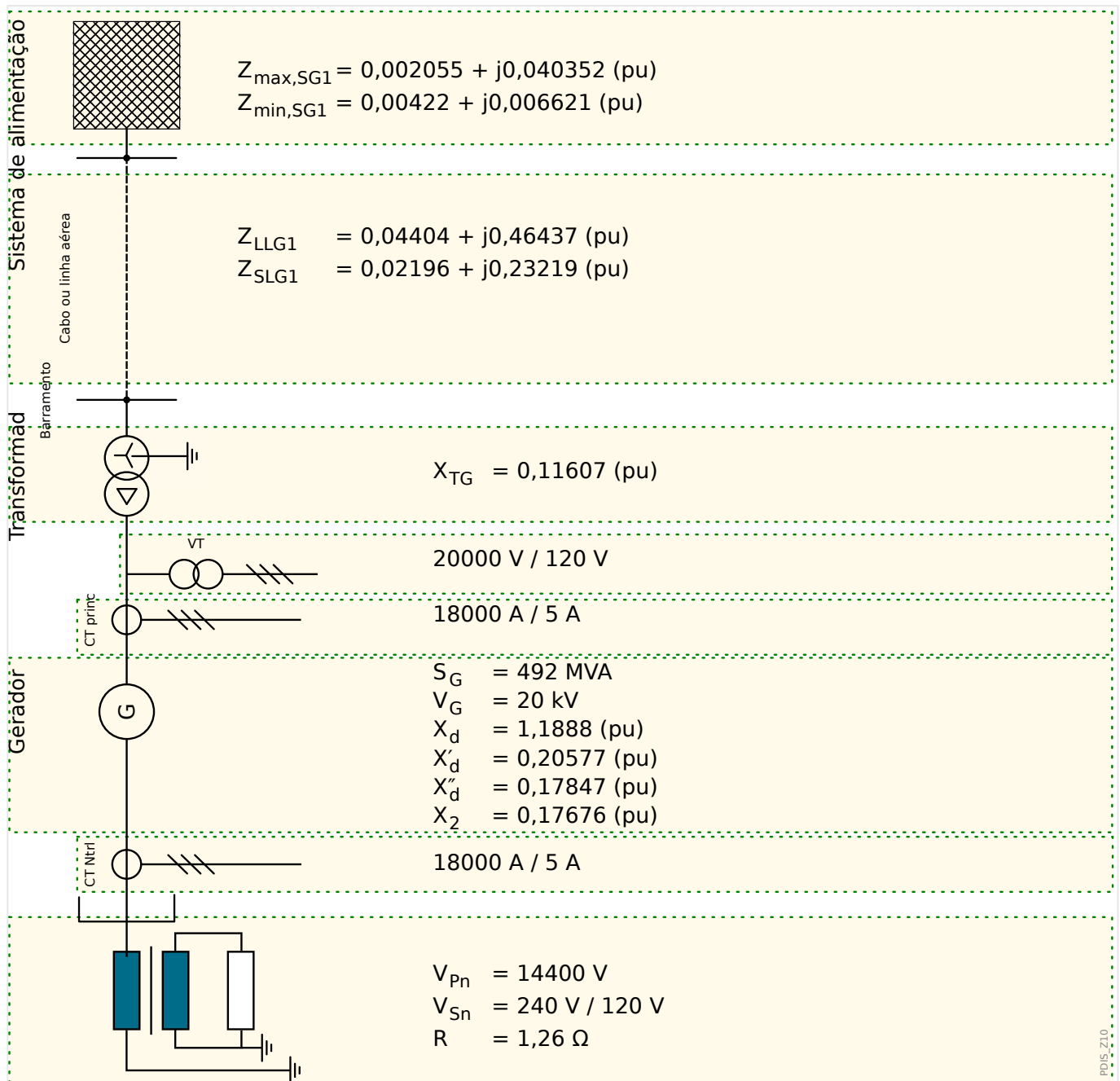
Fig. 99: Diagrama de linha única com dados baseados em gerador.
