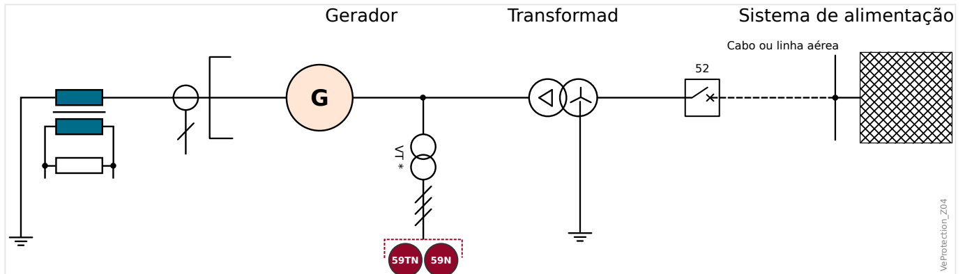
Fig. 128: 100% de proteção contra falha no aterramento do estator obtida com uma combinação ANSI 59TN/59N.
