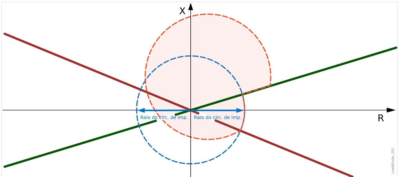
Fig. 109: Zona de disparo da proteção de distância (área vermelha) com difusor de carga ativa.
