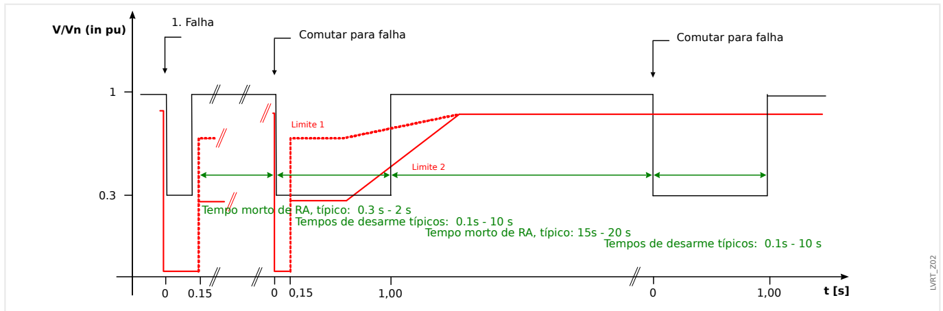
Fig. 143: Percurso de uma curva de tensão durante um autorreligamento malsucedido de dois disparos; fonte: Technische Richtlinie, Erzeugungsanlagen am Mittelspannungsnetz, Ausgabe Juni 2008, BDEW Bundesverband der Energie- und Wasserwirtschaft e.V. (página 89).
