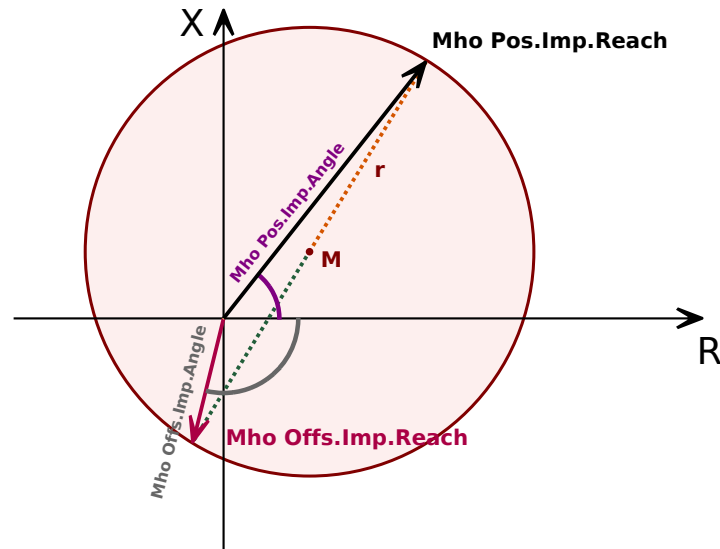
Fig. 92: Área operacional (colorida em vermelho brilhante) do tipo (círculo) MHO, com »Ativação de direção« = "inativo".
