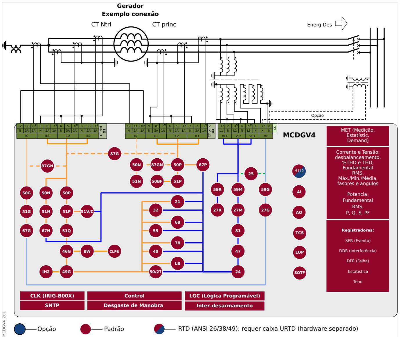
Fig. 1: Visão geral funcional do MCDGV4.
