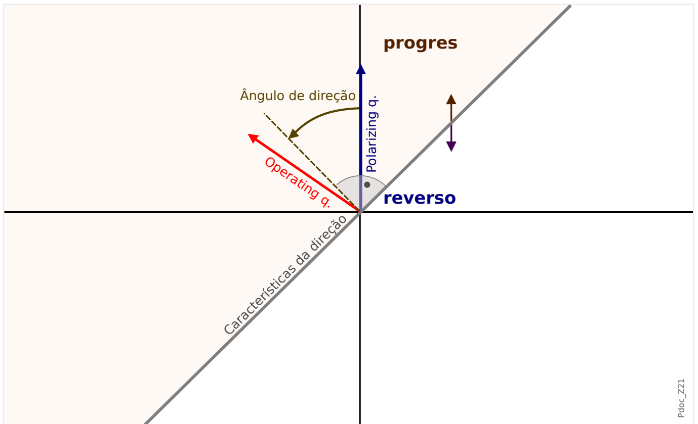
Fig. 72: Princípio de detecção da direção de falhas de fase
