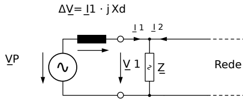
Fig. 129: Circuito equivalente no gerador síncrono em paralelo com a rede.
