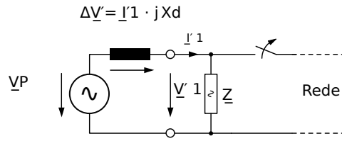
Fig. 131: Circuito equivalente em falha da rede
