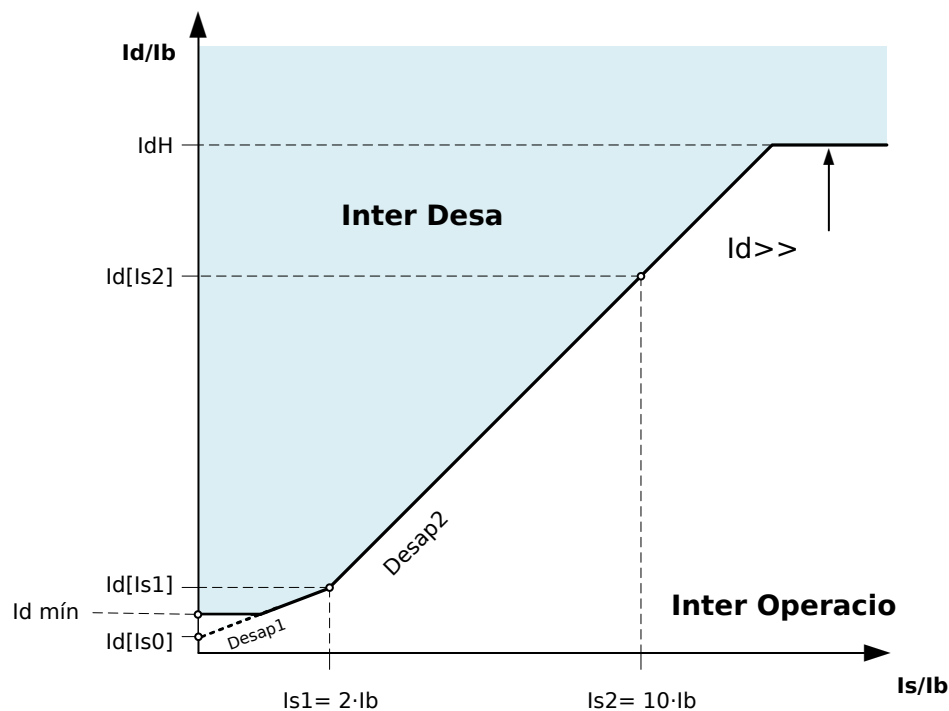
Fig. 86: Etapa da Proteção Diferencial Irrestrita de Alta Definição IdH.
