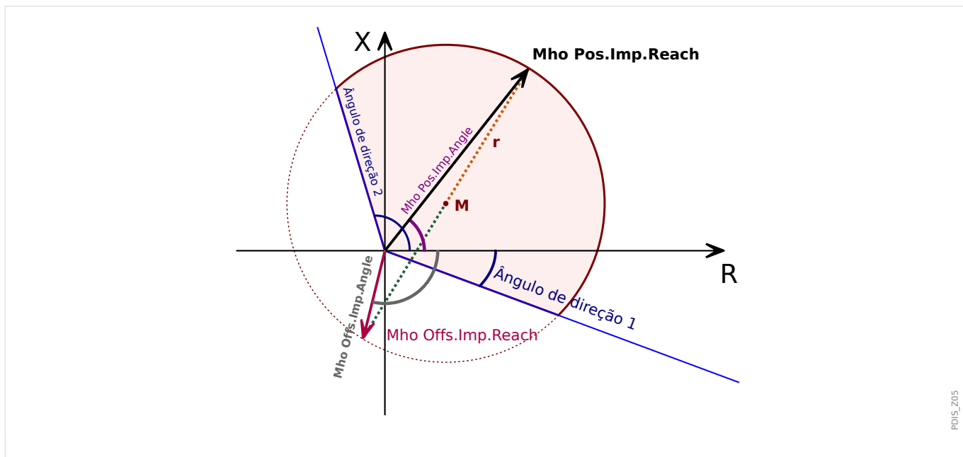
Fig. 93: Área operacional (colorida em vermelho brilhante) do tipo (círculo) MHO, com »Ativação de direção« = “ativo”.
