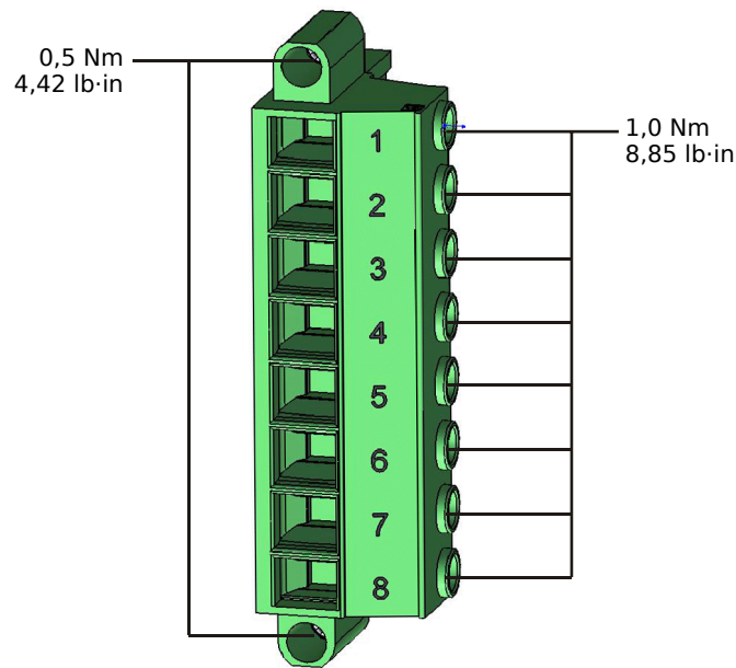
Fig. 175: Terminais de medição de tensão da placa de medição "TU" (↳ "TU - Entradas de Medição de Tensão").
