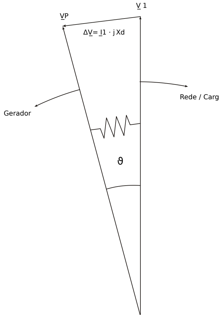
Fig. 130: Vetores de voltagem em operação paralela.
