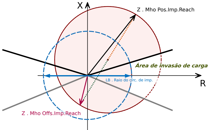
Fig. 96: Característica de impedância operacional (colorida em vermelho brilhante) com invasão de carga ativa.
