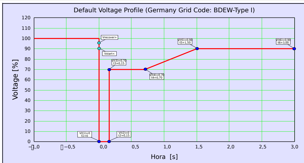
Fig. 145: Perfil padrão do LVRT (BDEW-Tipo I).
