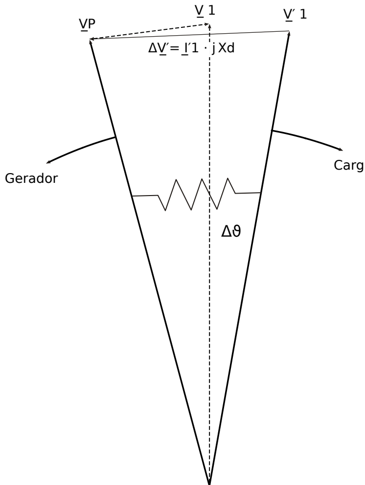
Fig. 132: Vetores de tensão em falha da rede
