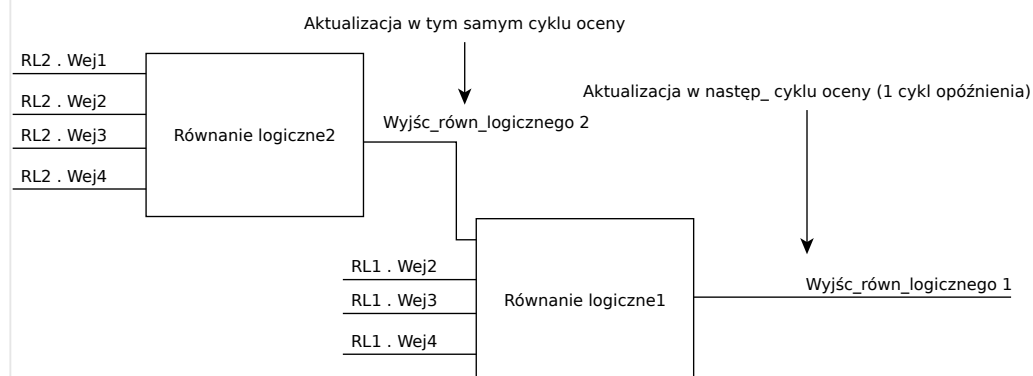
Rys. 170: Ukł. kaskadowy w porządku malejącym
