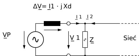
Rys. 129: Schemat zastępczy dla prądnicy synchronicznej pracującej równolegle z siecią.
