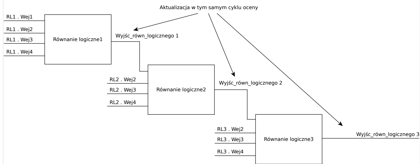
Rys. 169: Ukł. kaskadowy w porządku rosnącym
