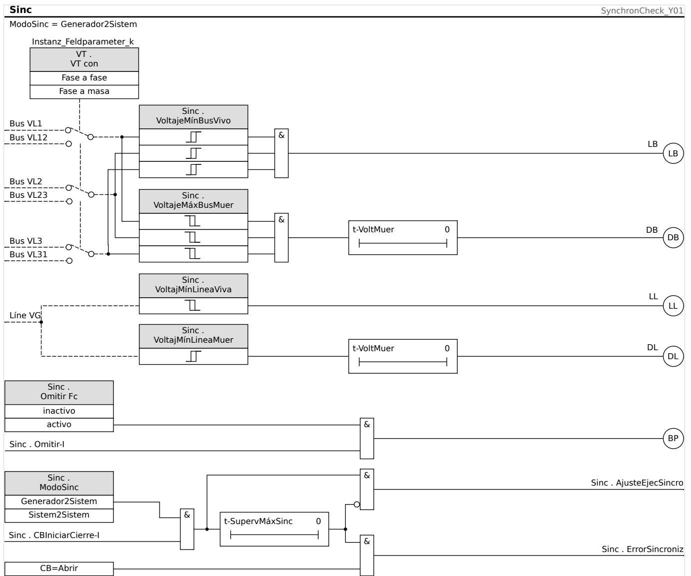
Fig. 137: Funcionalidad del módulo »Sinc«, «Generador2Sistem».
