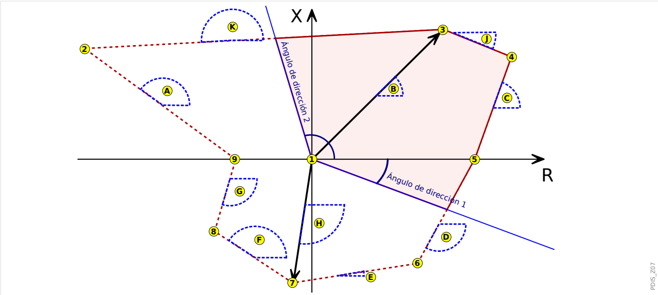
Fig. 95: Área de operación (en color rojo brillante) del tipo polígono, con »Activar dirección« = "activo".
