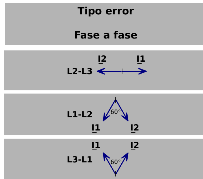
Fig. 90: Fasores de corriente de secuencia de fase positiva y negativa para distintos tipos de fallo.
