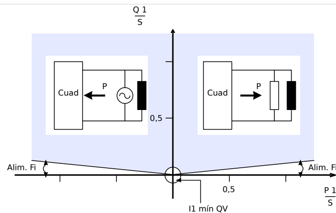
Fig. 140: Método 1: Supervisión de ángulo de potencia
