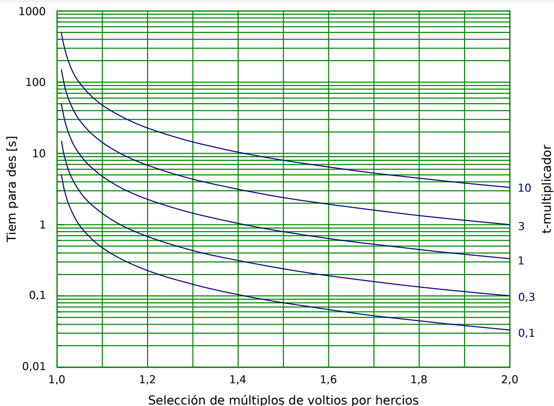
Fig. 116: Características/Forma curva: INV A
