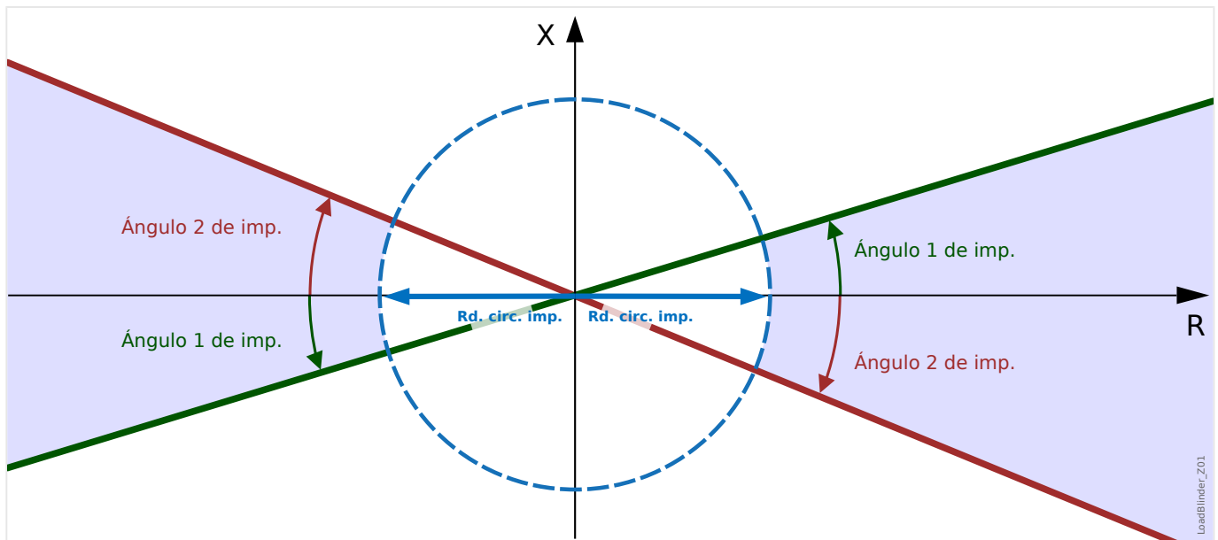
Fig. 108: Característica de blindaje de carga (zona resaltada de color azul).
