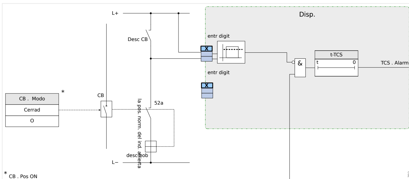
Fig. 151: Ejemplo de conexión: Supervisión del circuito de desconexión solo con un contacto auxiliar CB »Aux ON« (52a).
