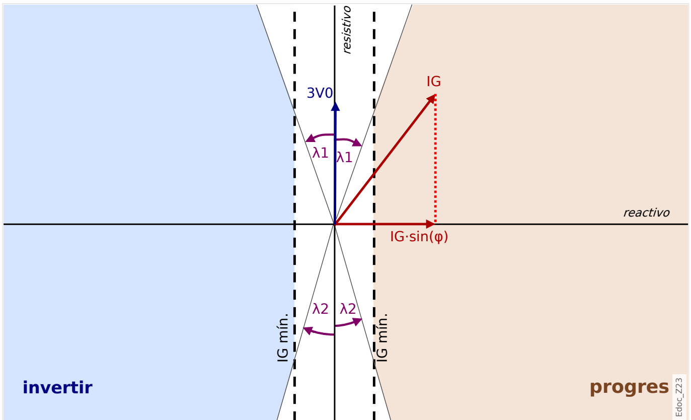
Fig. 77: Principio para determinar la dirección en el método "sin( \phi )".
