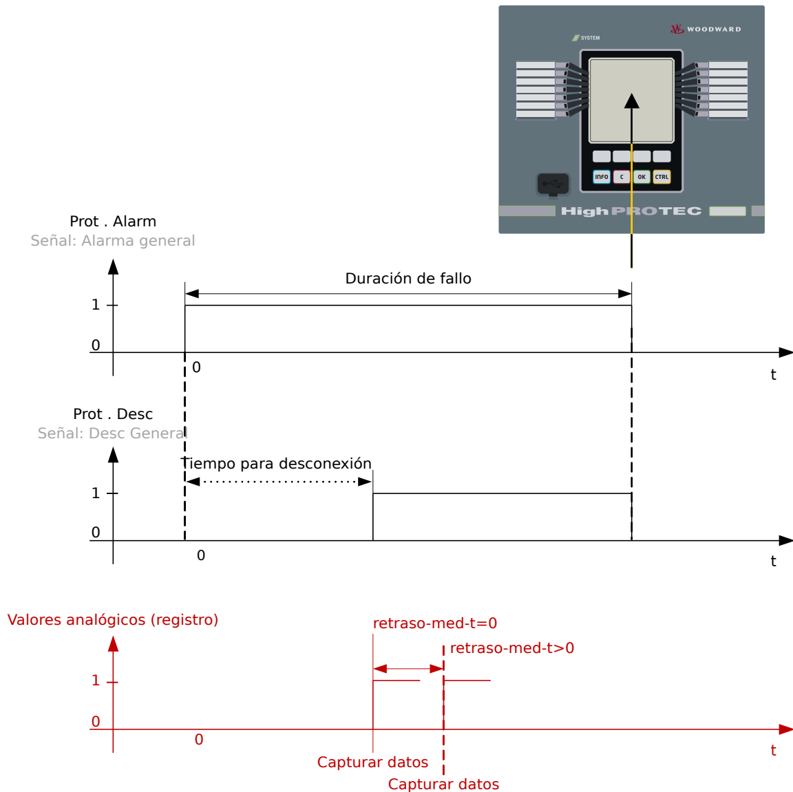
Fig. 164: Registrador de fallos: tiempos y duraciones.
