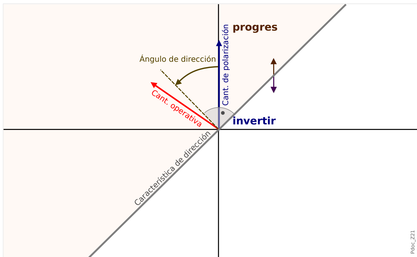
Fig. 72: Principio de detección de dirección de fallo de fase
