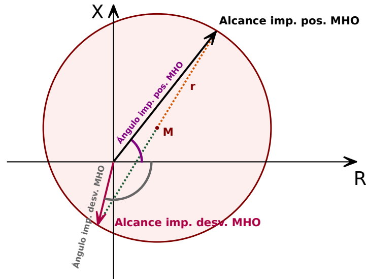
Fig. 92: Área de operación (en color rojo brillante) del tipo MHO (círculo), con «Activar dirección» = «inactivo».
