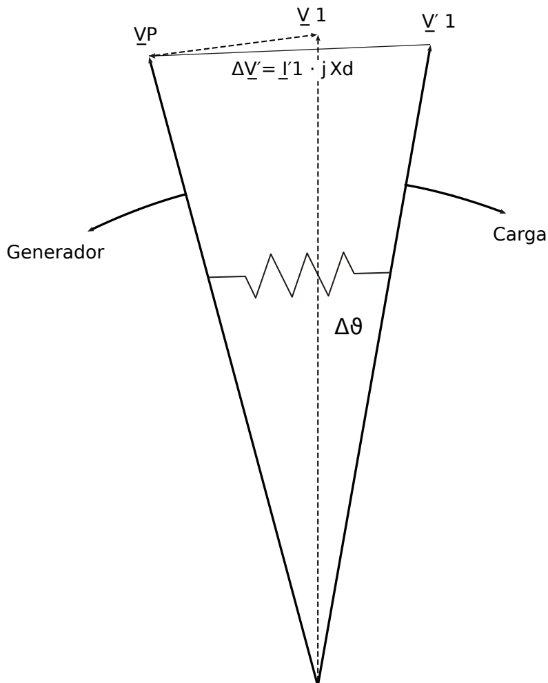
Fig. 132: Fallo de los vectores de tensión en la red.
