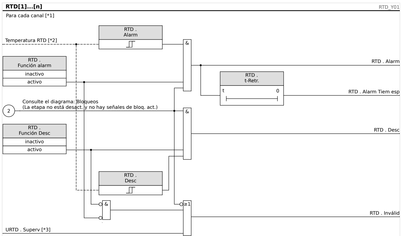
Fig. 148: El principio de funcionamiento general (alarma retrasada, desconexión sin retraso).
