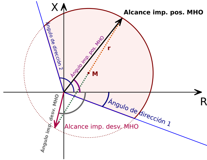
Fig. 93: Área de operación (en color rojo brillante) del tipo MHO (círculo), con «Activar dirección» = “activo”.
