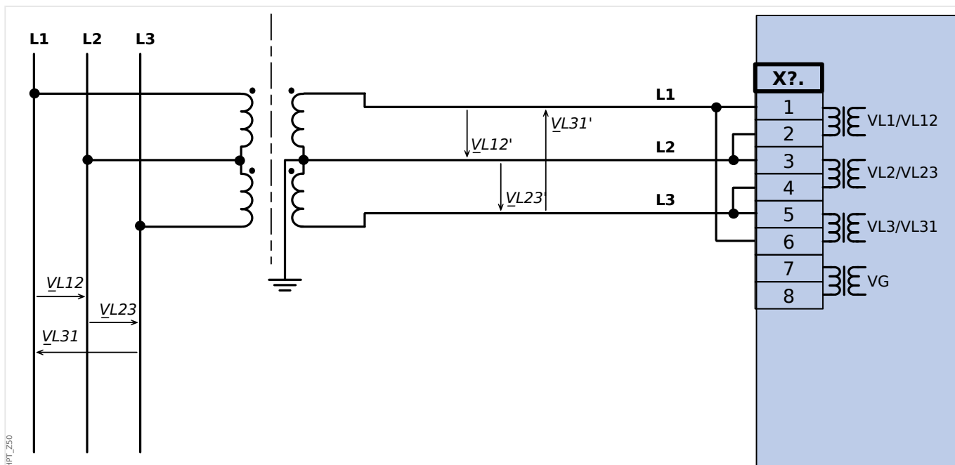
Fig. 42: Medida voltaje bifásico: cableado de las entradas de medida: "Abr. Delta"
