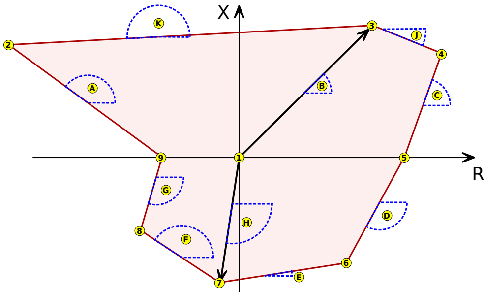
Fig. 94: Área de operación (en color rojo brillante) del tipo polígono, con «Activar dirección» = “inactivo”.
