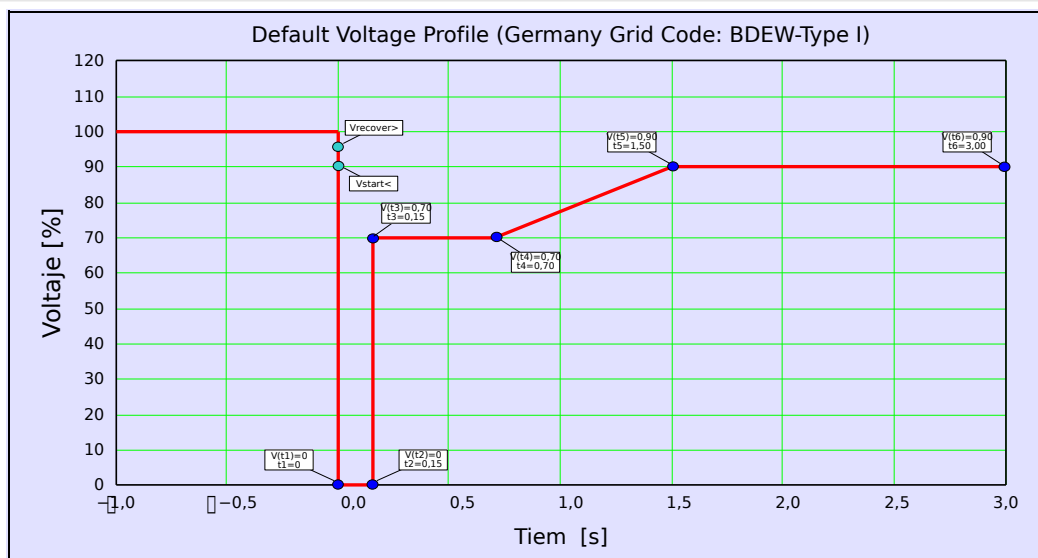
Fig. 145: Perfil de LVRT predeterminado (Tipo I de BDEW).
