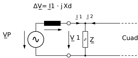
Fig. 129: Circuito equivalente en generador sincrónico en paralelo con la red de suministro eléctrico.
