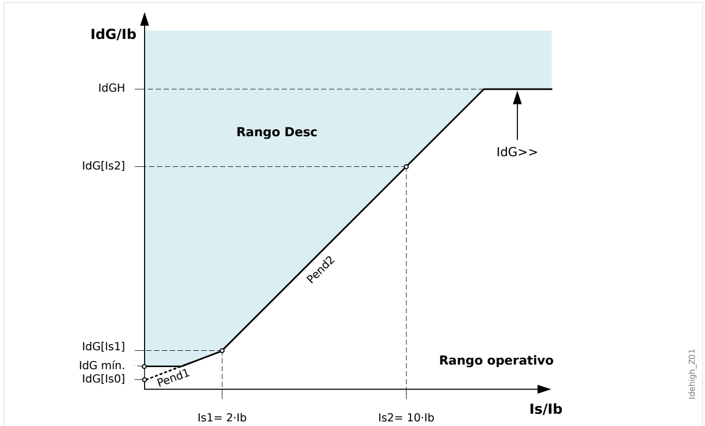
Fig. 88: Valor de selección \gg I_dG \gg de la corriente de diferencial de tierra basada en la corriente nominal \gg lb del objeto de protección relacionado.
