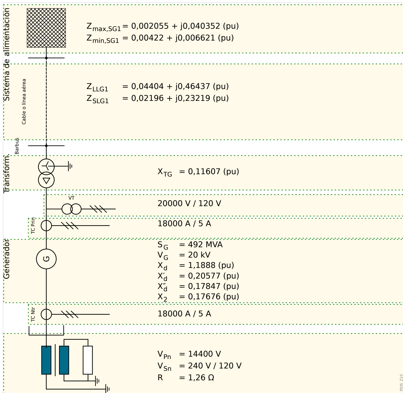
Fig. 99: Diagrama de línea única con datos basados en el generador.
