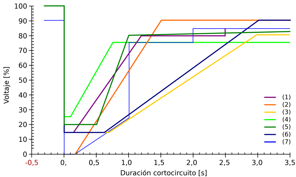
Fig. 142: Estándares de LVRT; fuente: eBWK Bd. 60 (2008) N.º 4. Autores: Dipl.-Ing. Thomas Smolka, Dr.-Ing. Karl-Heinz Weck, Zertifizierungstelle der FGH e.V., Mannheim, sowie Dipl.-Ing. (FH) Matthias Bartsch, Enercon GmbH, Aurich.
