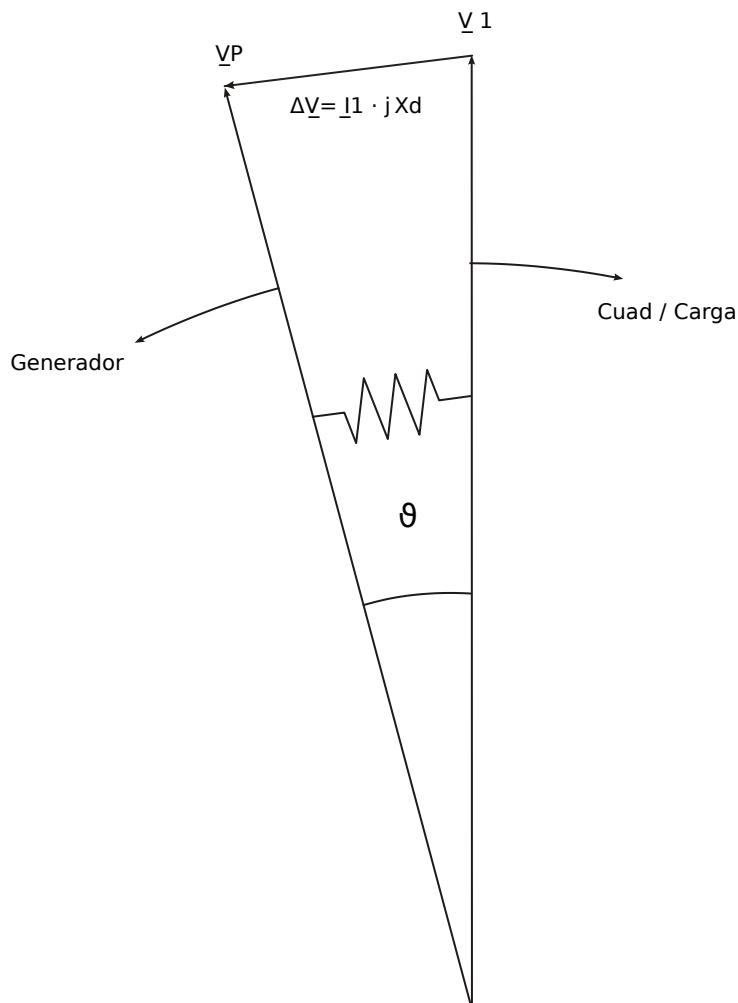
Fig. 130: Vectores de tensión en funcionamiento en paralelo con la red de suministro eléctrico.
