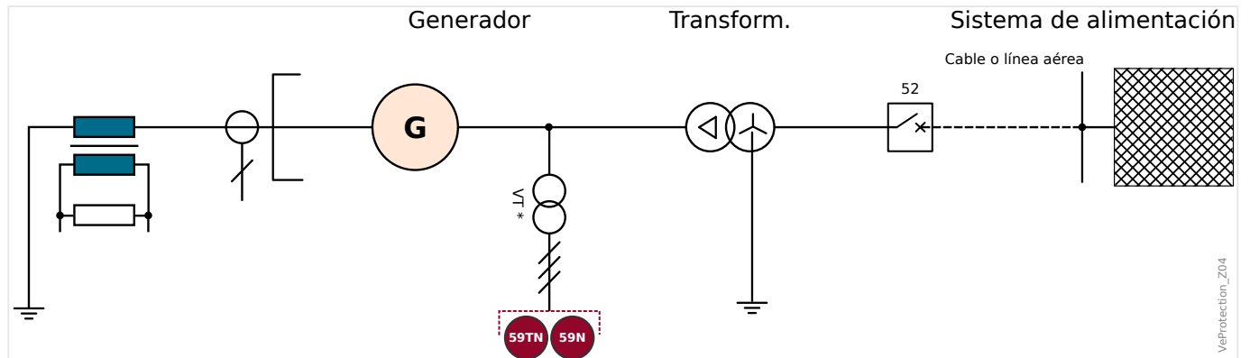
Fig. 128: Protección de fallo de tierra de estator del 100% obtenida con la combinación ANSI 59TN/59N.
