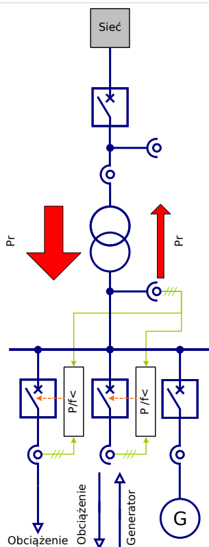
Rys. 95: Zdecentralizowane podczęstotliwościowe zmniejszanie obciążenia w sieciach z tymczasowym zasilaniem.
