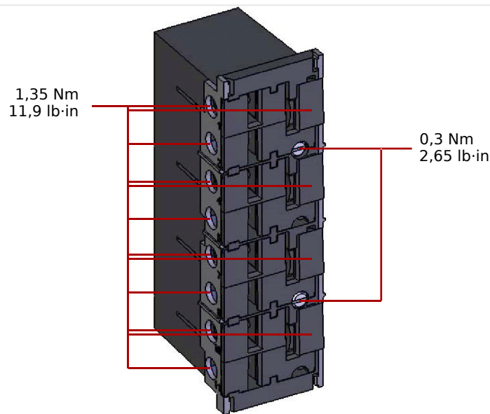
Rys. 138: Łącznik wtykowy ze zintegrowanym elementem zwarciovym (konwencjonalne wejścia prądowe)
