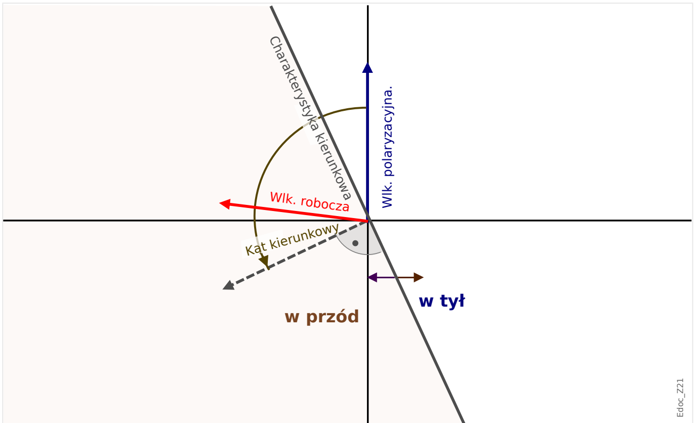
Rys. 63: Zasada określania kierunku obowiązująca dla wszystkich metod z wyjątkiem „ \cos(\phi) ”, „ \sin(\phi) ”.
