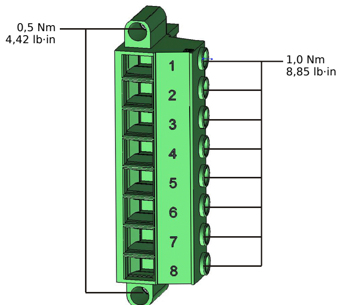
Rys. 139: Zaciski pomiaru napięcia karty pomiarowej „TU” (↳ „TU — wejścia do pomiaru napięcia”).
