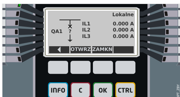
Rys. 119: Przykład strony sterowania z wyłącznikiem w pozycji zakłóconej (lub nieprawidłowej).
