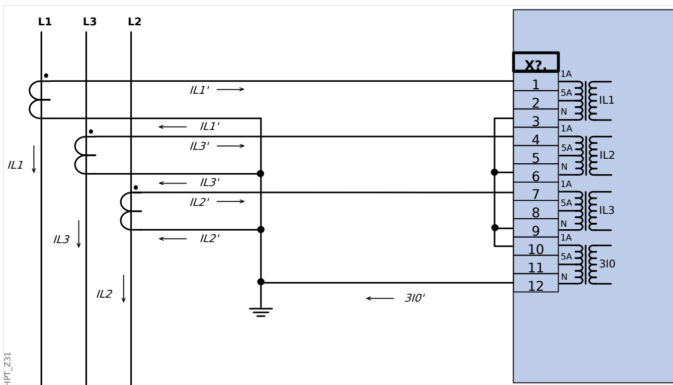
Rys. 24: Trójfazowy pomiar prądu; I_n wtórny = 1 A. Pomiar prądu doziemnego w układzie Holmgreena 310n wtórny = 1 A.
