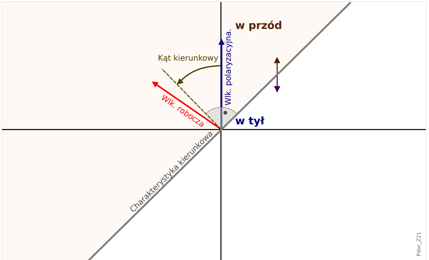
Rys. 61: Zasada wykrywanie kierunku zwarcia międzyfazowego.
