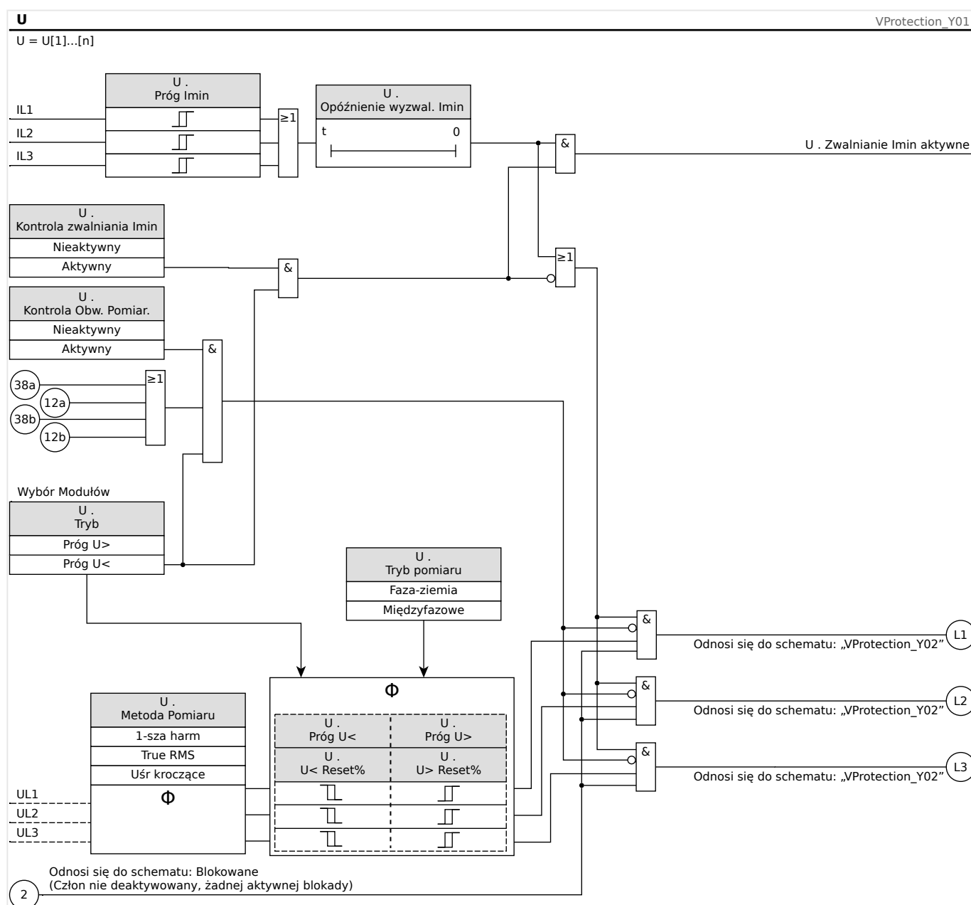
Rys. 73: Działanie modułu zabezpieczenia napięciowego, część 1.
