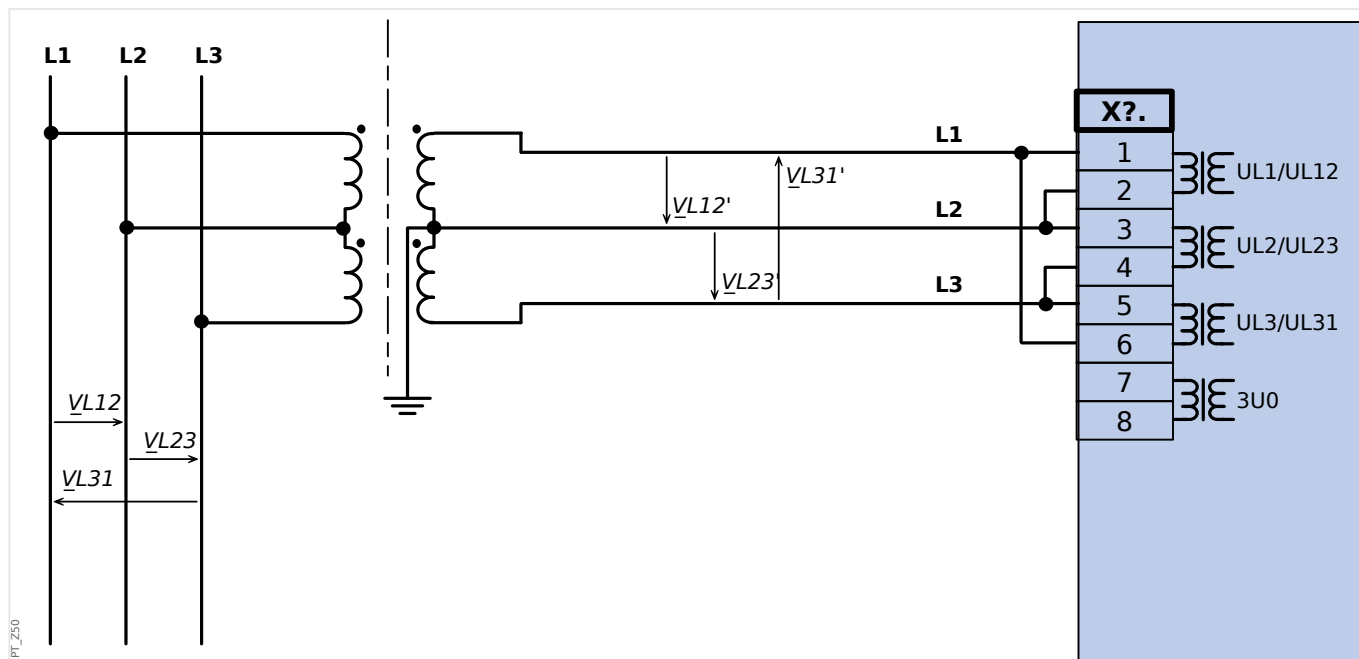
Rys. 34: Pomiar napięcia dla dwóch faz w układzie otwartego trójkąta
