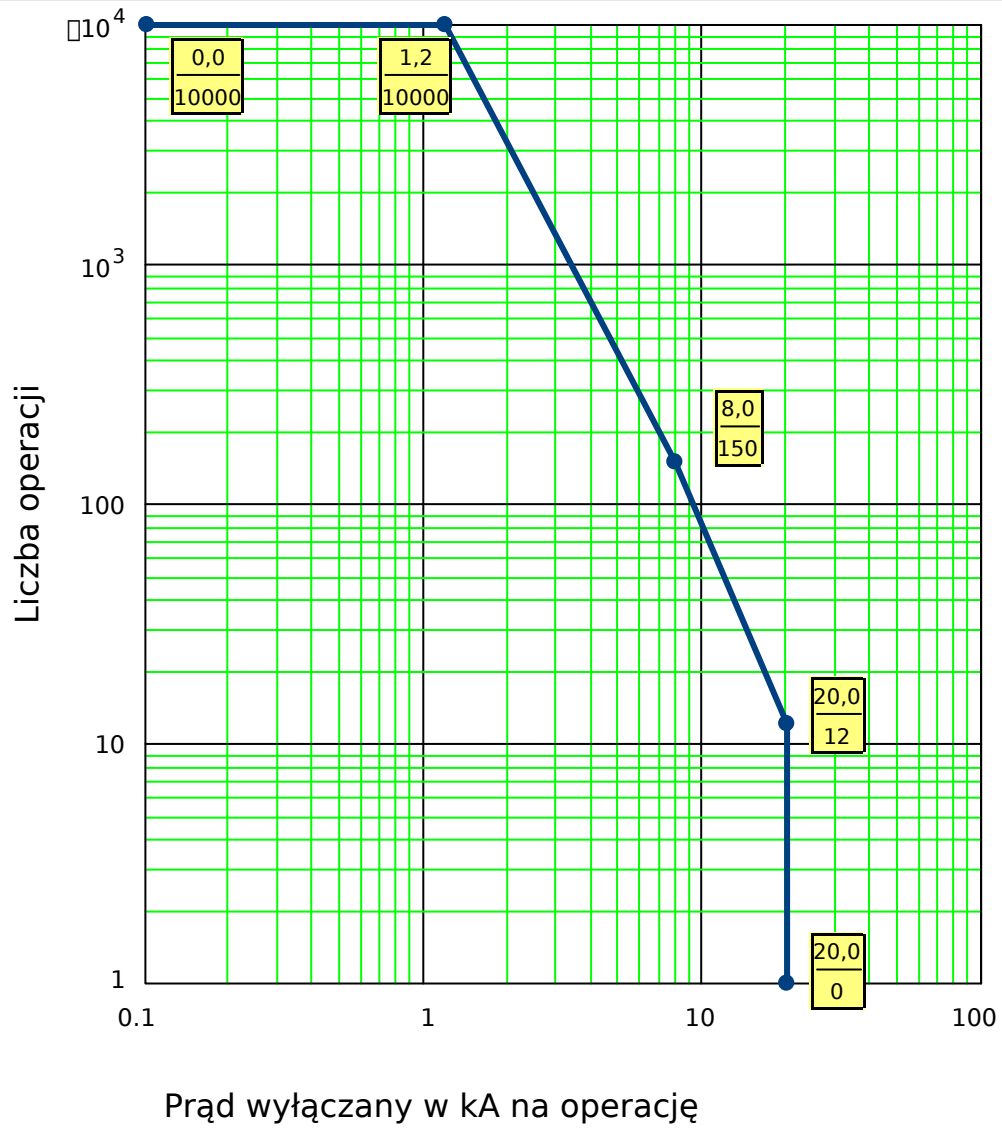
Rys. 123: Krzywa konserwacji wyłącznika typowego wyłącznika 25 kV
