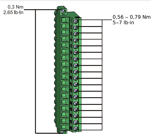
Rys. 140: Zaciski pomiaru napięcia kart pomiarowych „TU-OR5” i „TU-DI8”).
