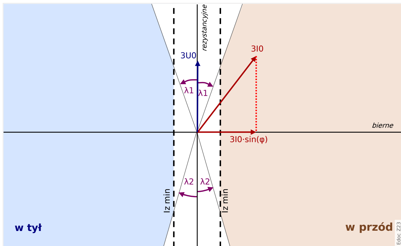
Rys. 66: Zasada określania kierunku metodą „sin( \phi )”.
