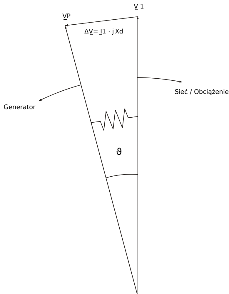
Rys. 84: Wektory napięcia przy pracy równoległej z siecią.
