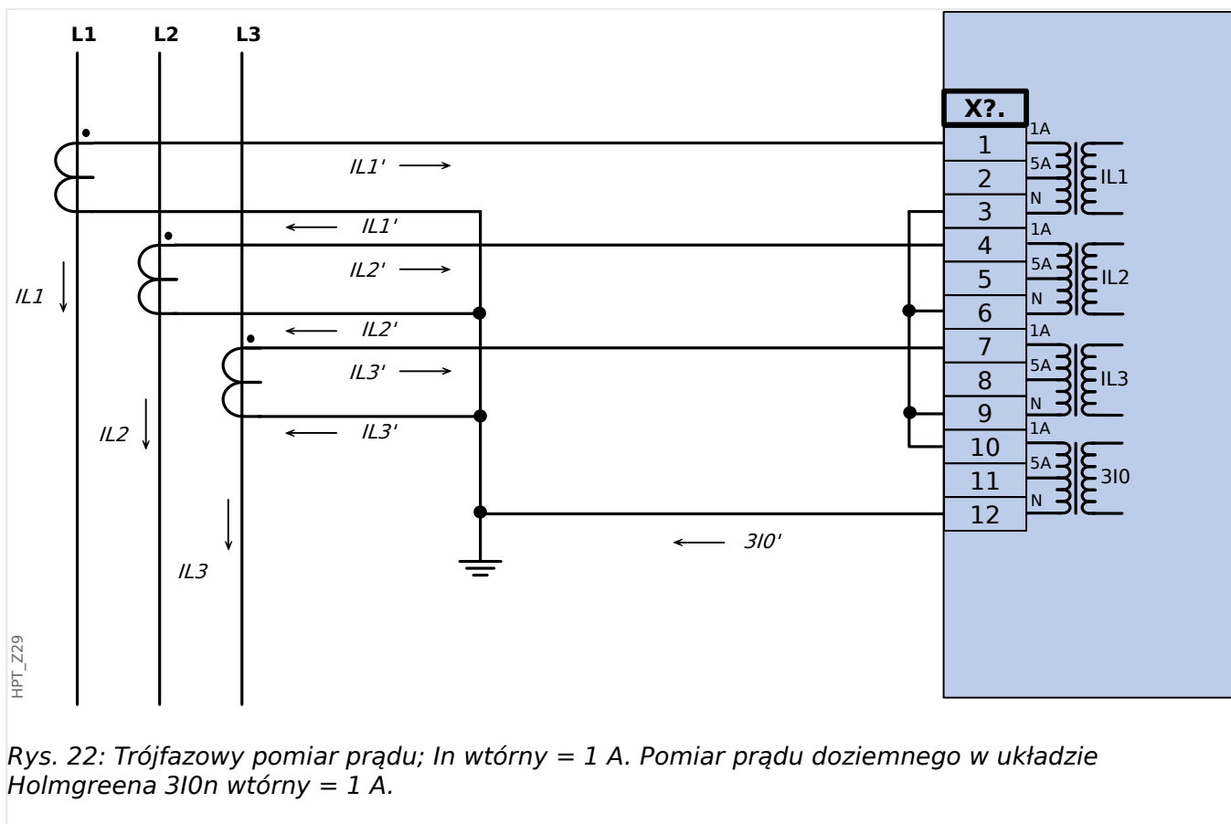
Rys. 21: Trójfazowy pomiar prądu; I_n wtórny = 5 A. Pomiar prądu doziemnego w układzie Holmgreena 310n wtórny = 5 A.
