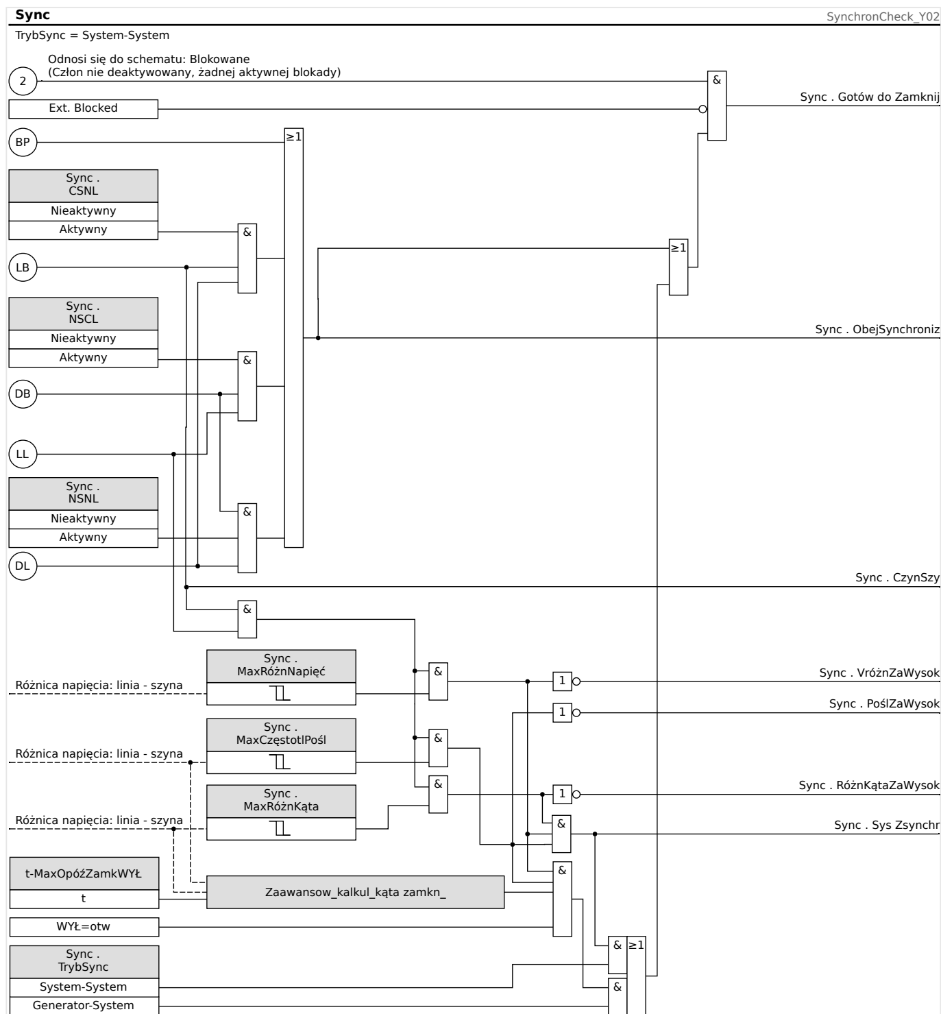
Rys. 111: Działanie modułu „Sync”, „System-System”.
