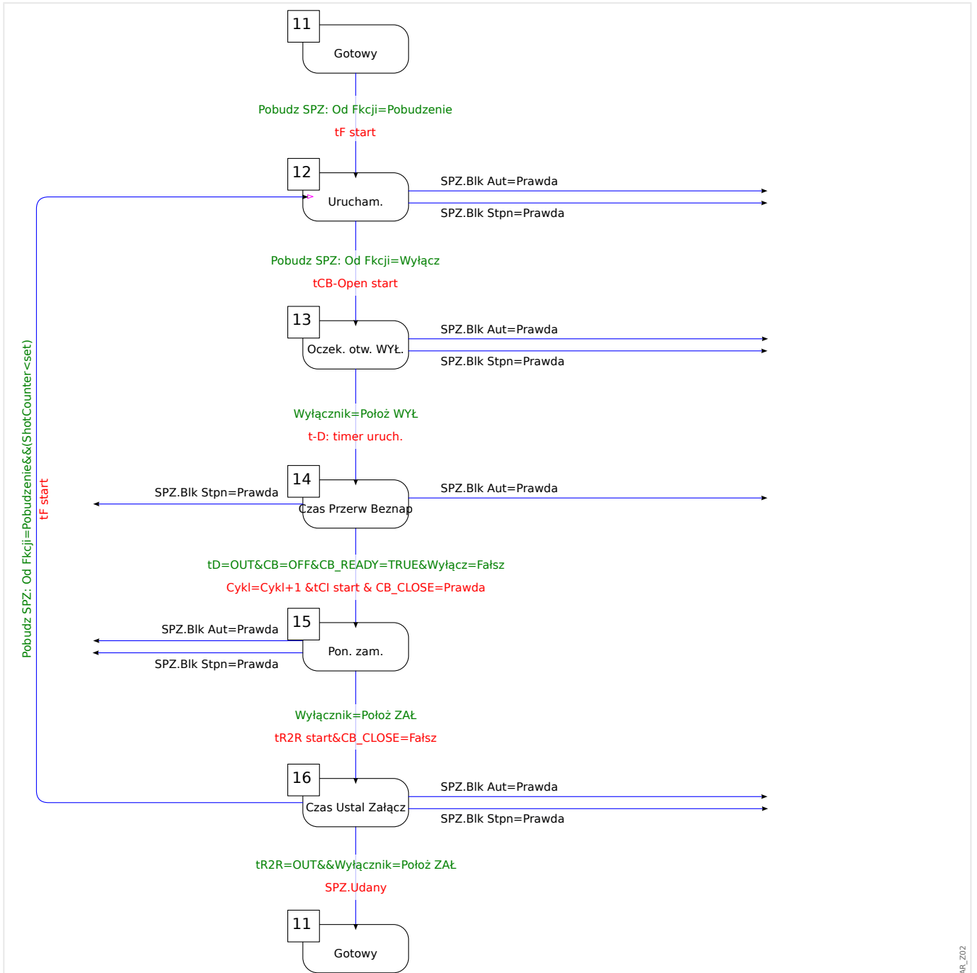
Rys. 101: Cykl pracy SPZ (stan 4).
