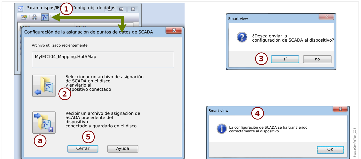
Fig. 58: Ejemplo de uso de Smart view para transferir el archivo *.HptSMap al dispositivo de protección.
