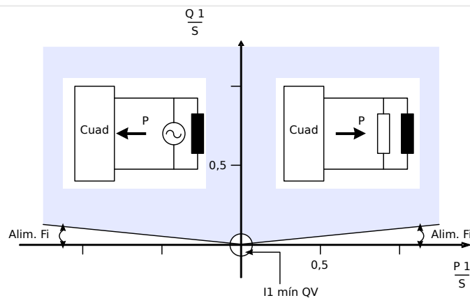
Fig. 90: Método 1: Supervisión de ángulo de potencia
