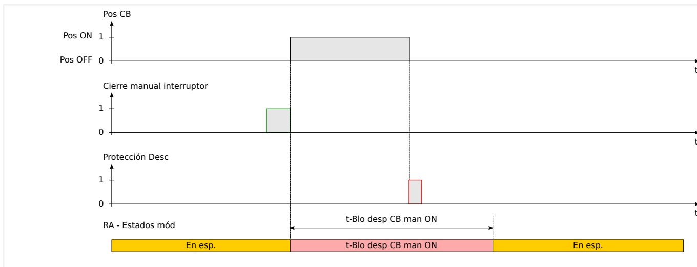
Fig. 105: Desconexión de protección mientras transcurre el tiempo de bloqueo de cierre manual.
