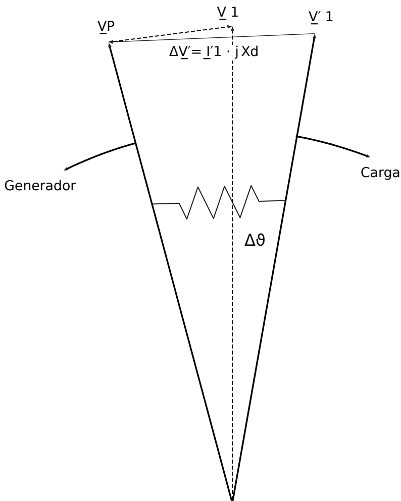
Fig. 86: Fallo de los vectores de tensión en la red.
