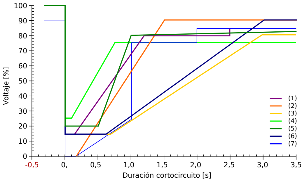
Fig. 76: Estándares de LVRT; fuente: eBWK Bd. 60 (2008) N.º 4. Autores: Dipl.-Ing. Thomas Smolka, Dr.-Ing. Karl-Heinz Weck, Zertifizierungstelle der FGH e.V., Mannheim, sowie Dipl.-Ing. (FH) Matthias Bartsch, Enercon GmbH, Aurich.
