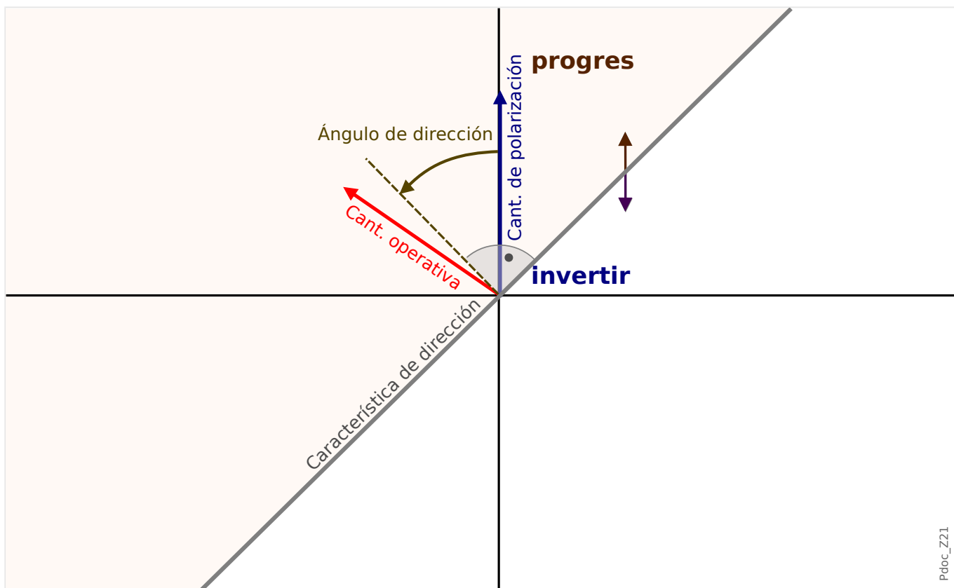
Fig. 61: Principio de detección de dirección de fallo de fase
