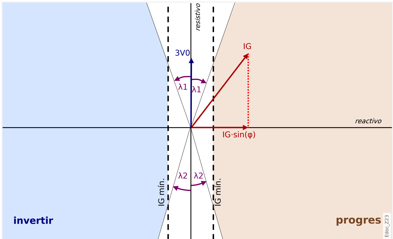
Fig. 66: Principio para determinar la dirección en el método "sin(φ)".
