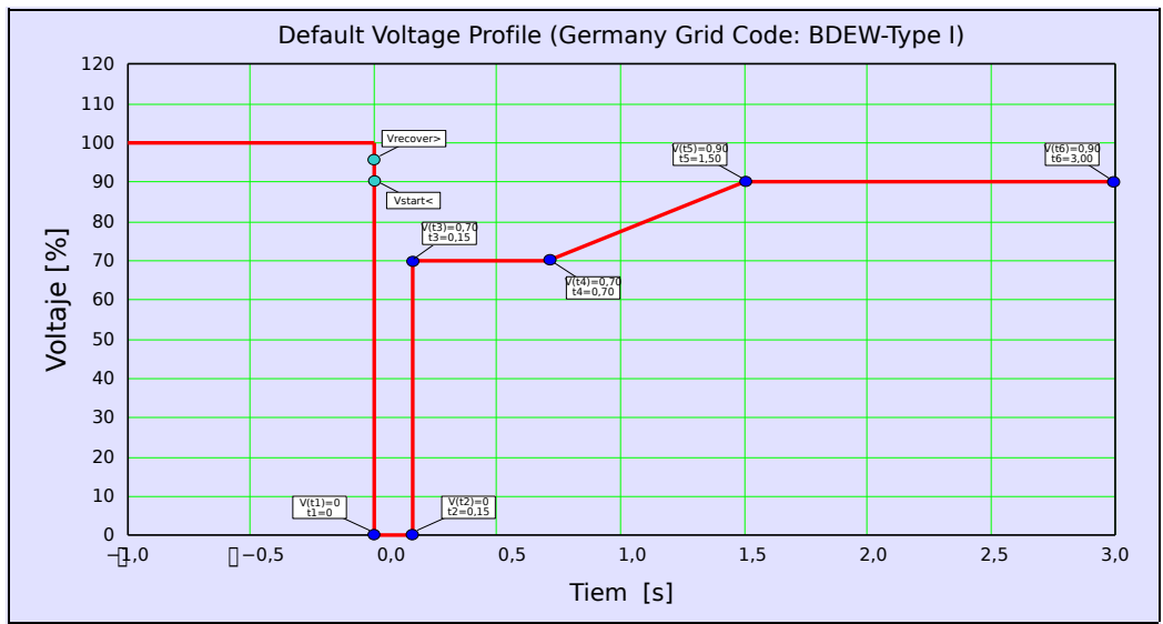
Fig. 79: Perfil de LVRT predeterminado (Tipo I de BDEW).
