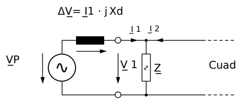
Fig. 83: Circuito equivalente en generador sincrónico en paralelo con la red de suministro eléctrico.
