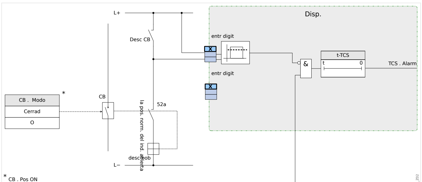
Fig. 115: Ejemplo de conexión: Supervisión del circuito de desconexión solo con un contacto auxiliar CB »Aux ON« (52a).
