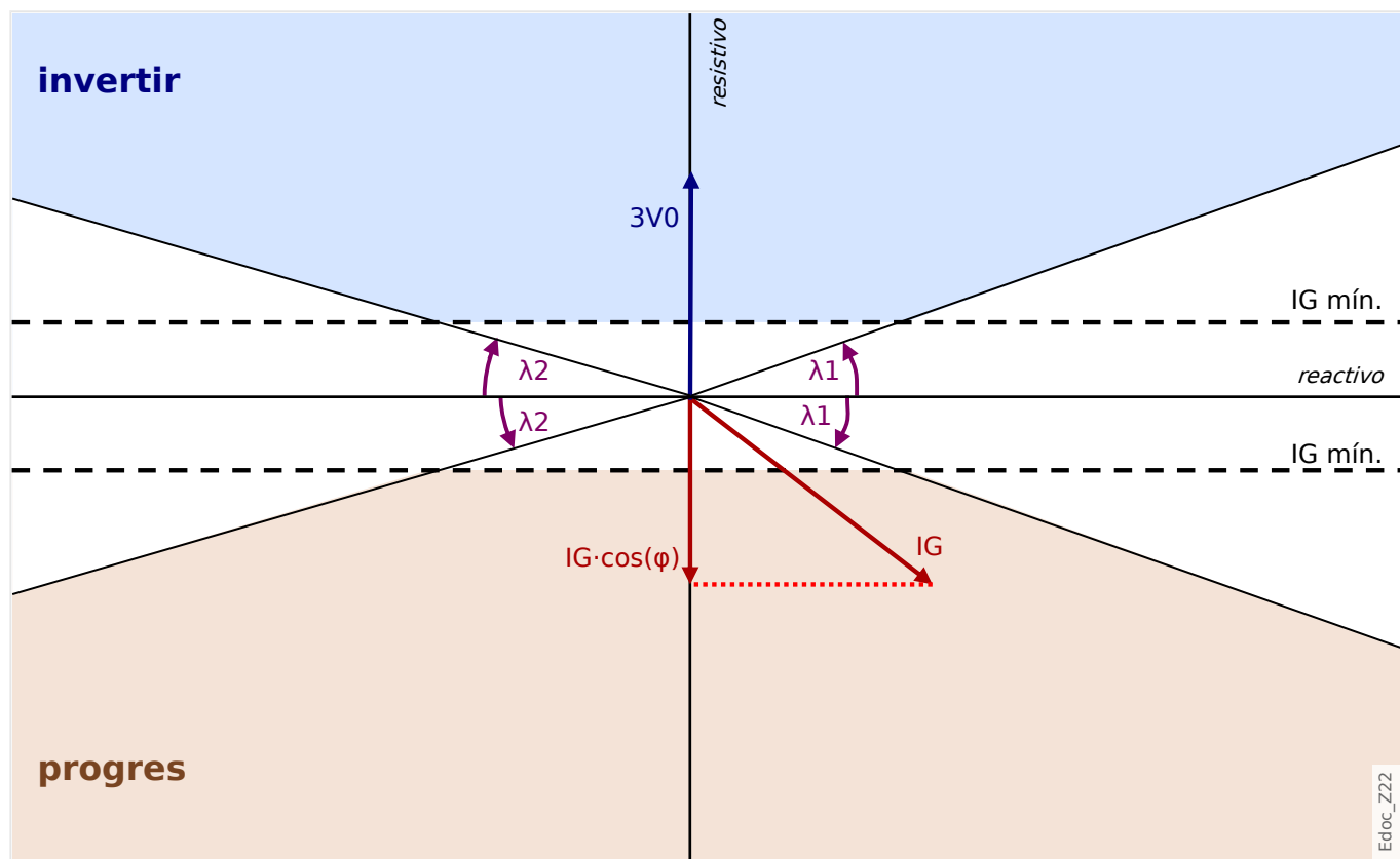
Fig. 65: Principio para determinar la dirección en el método "cos(φ)".
