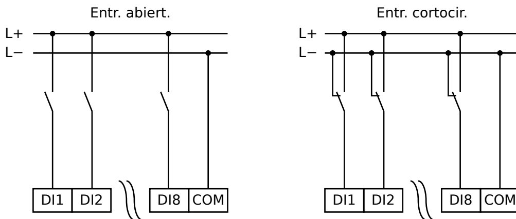
Fig. 141: Estado seguro de entradas digitales
