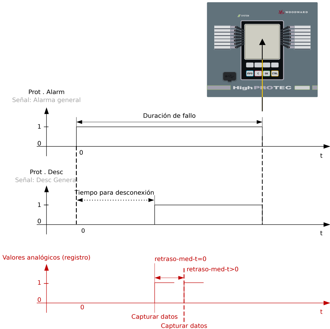
Fig. 128: Registrador de fallos: tiempos y duraciones.
