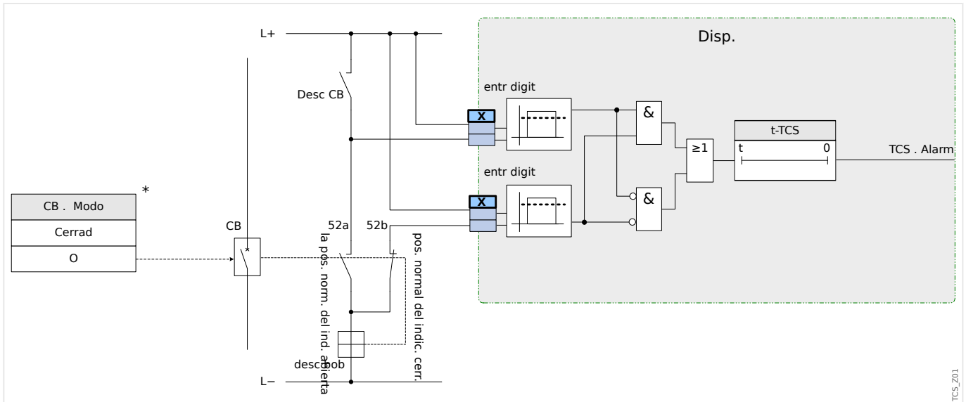
Fig. 114: Ejemplo de conexión: Supervisión del circuito de desconexión con dos contactos auxiliares CB »Aux ON« (52a) and »Aux OFF« (52b).
