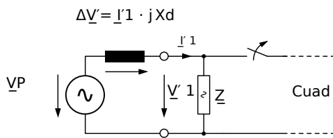
Fig. 85: Circuito equivalente en fallo de red eléctrica.
