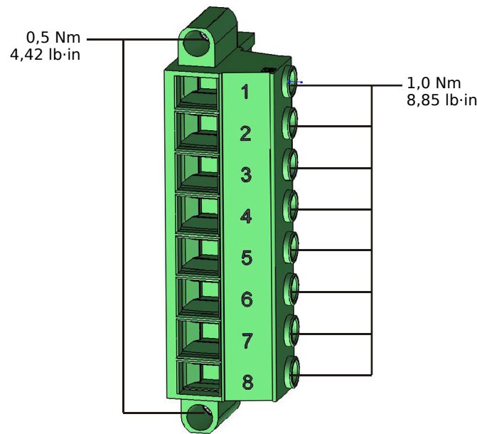
Fig. 139: Terminales de medición de tensión de la tarjeta de medición “TU” (↳ «TU - Entradas de medición de tensión»).
