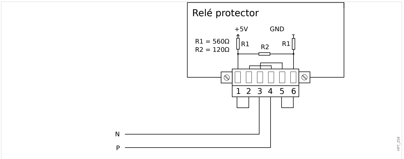
Fig. 48: Ejemplo de cableado, dispositivo en el final de BUS (ajuste de puentes de cable para activar el resistor de terminal integrado)
