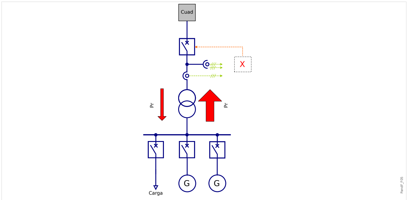
Fig. 96: Uso centralizado en redes con alimentación predominante.
