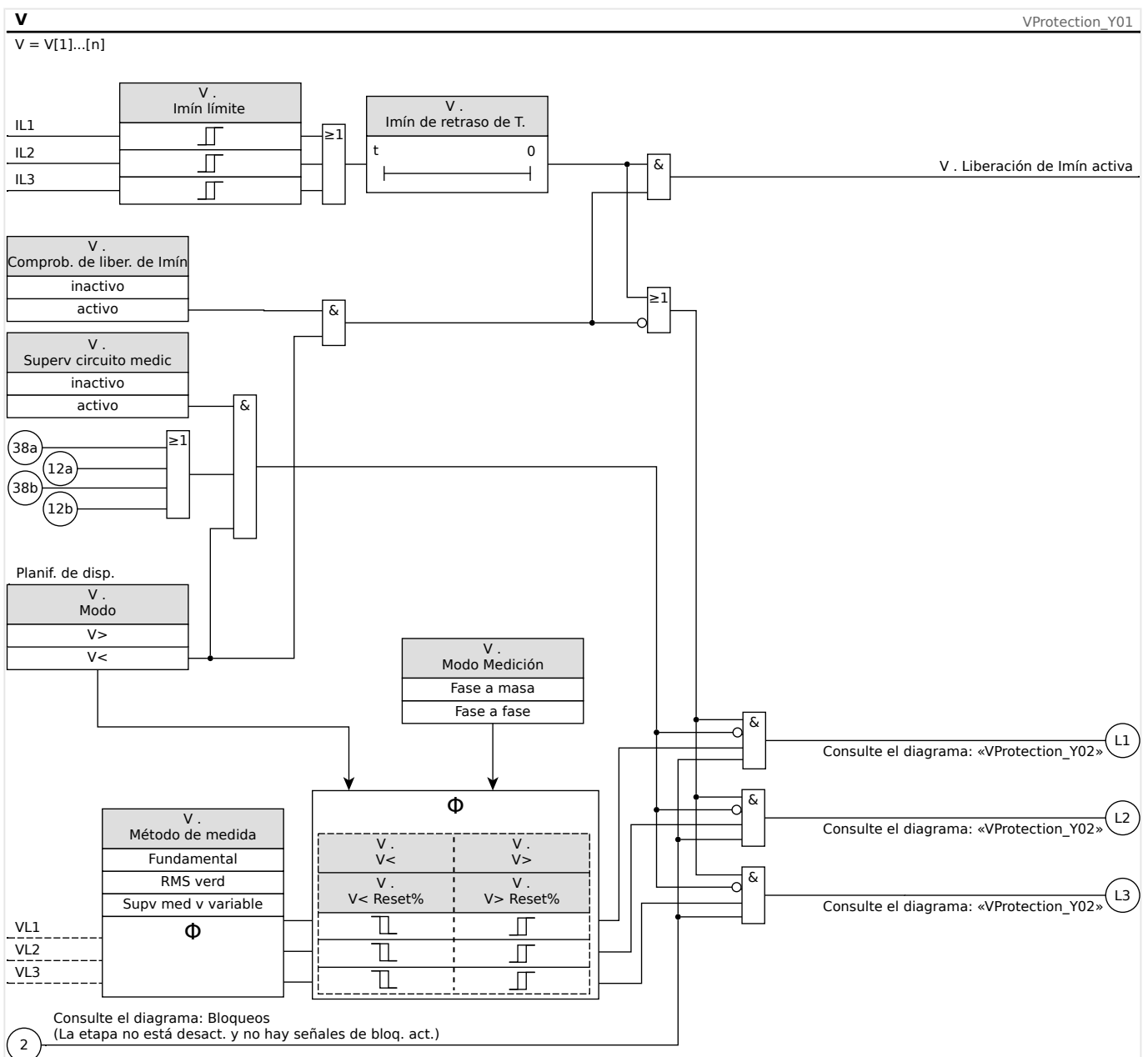
Fig. 73: Funcionalidad del módulo de protección de tensión, parte 1.
