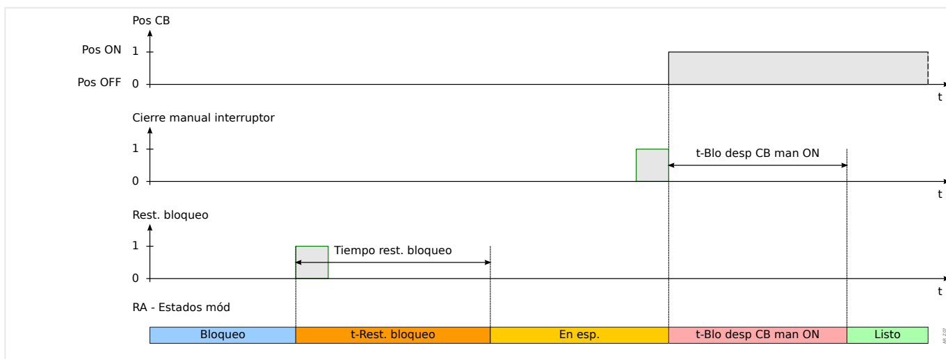
Fig. 106: Lógica de reinicio de bloqueo de AR en caso de que el reinicio de bloqueo llegue antes de que se cierre el interruptor manualmente.
