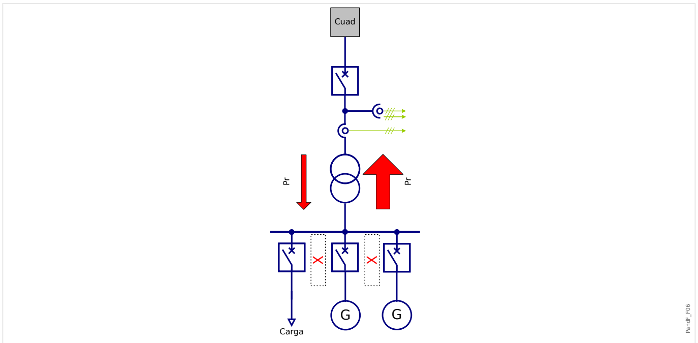
Fig. 97: Uso descentralizado en redes con alimentación predominante.
