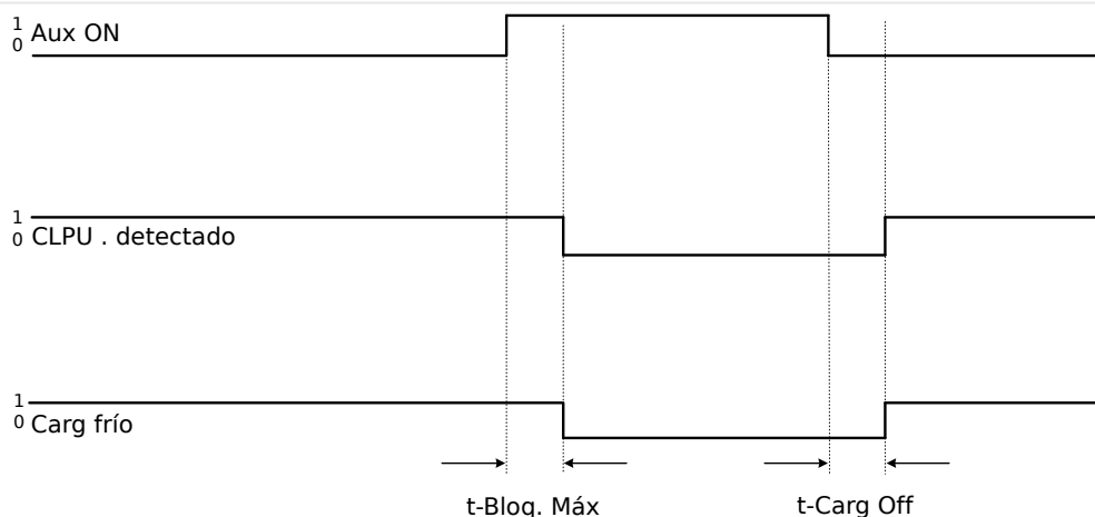
Fig. 112: Modo de ejemplo: Posición de interruptor.
