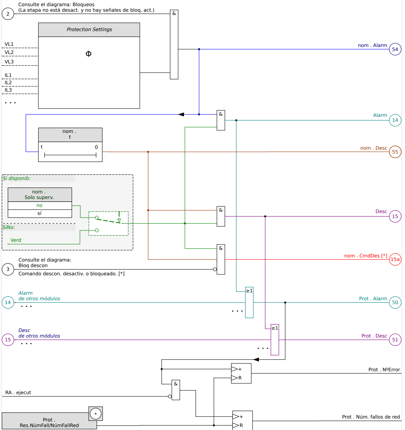
Fig. 60: Descripción a grandes rasgos de la funcionalidad de cualquier elemento de protección de HighPROTEC.
