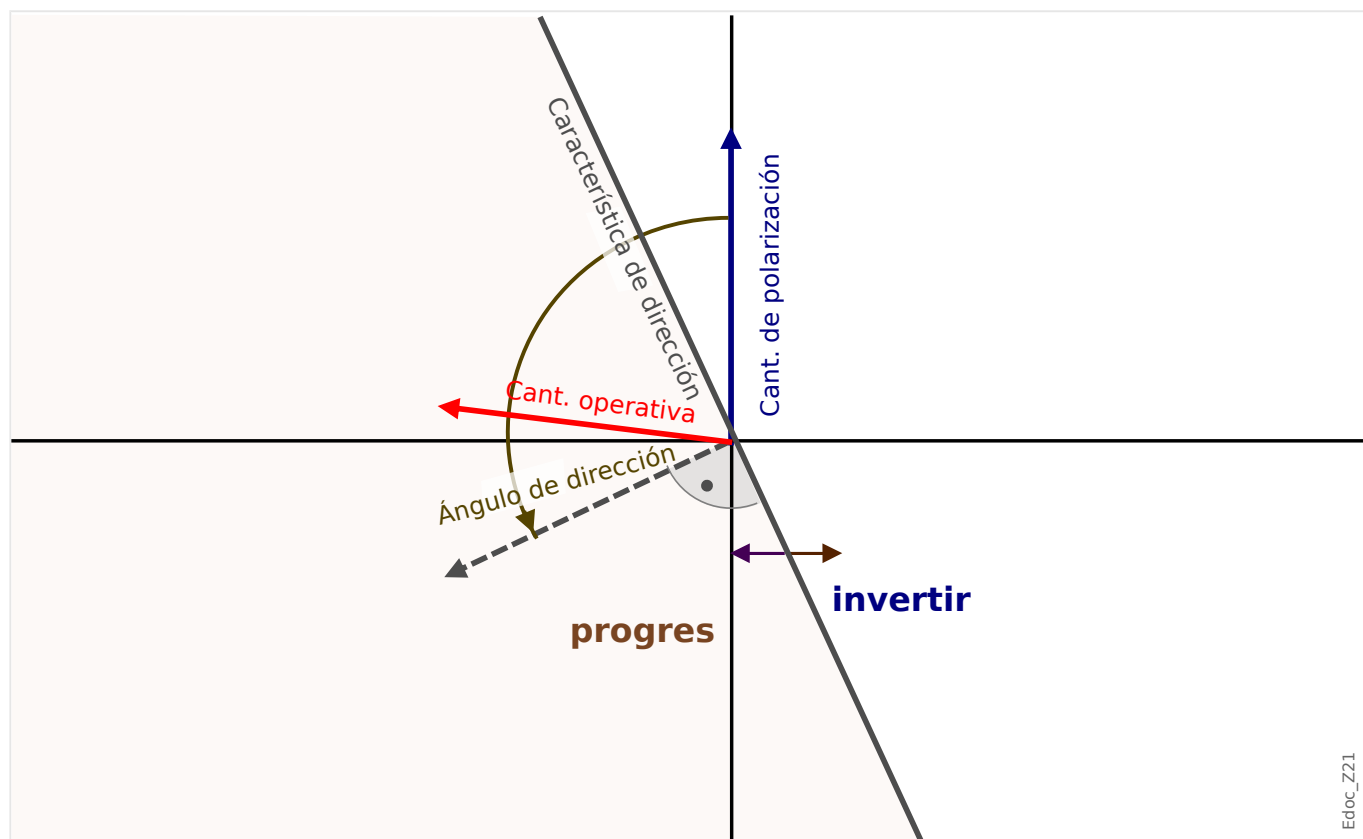
Fig. 63: Principio para determinar la dirección en todos los métodos, excepto “ \cos(\phi) ”, “ \sin(\phi) ”.
