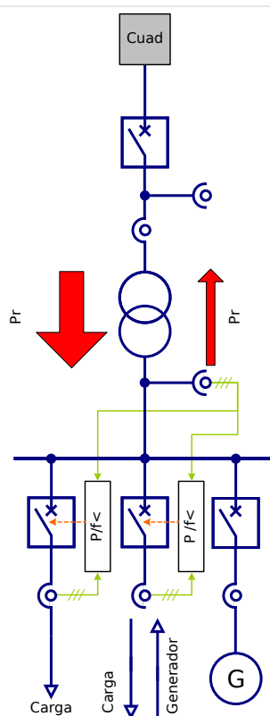
Fig. 95: Reducción de carga descentralizada por subfrecuencia en redes eléctricas con alimentación temporal.
