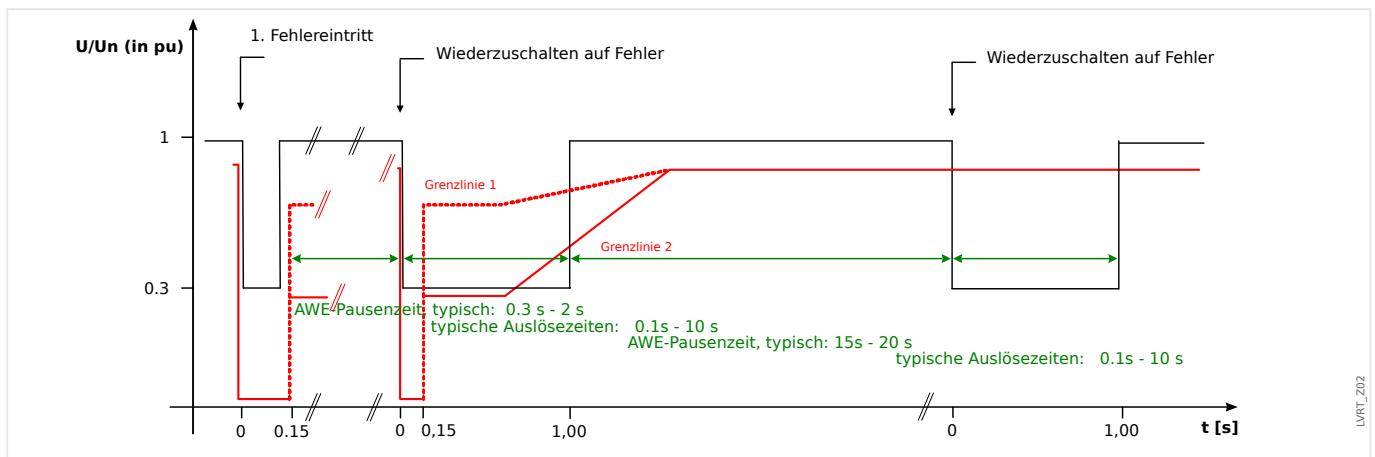
Abb. 76: Spannungsverlauf während einer zweischüssigen, nicht erfolgreichen AWE, aus: Technische Richtlinie, Erzeugungsanlagen am Mittelspannungsnetz, Ausgabe Juni 2008, BDEW Bundesverband der Energie- und Wasserwirtschaft e.V. (Page 89).
