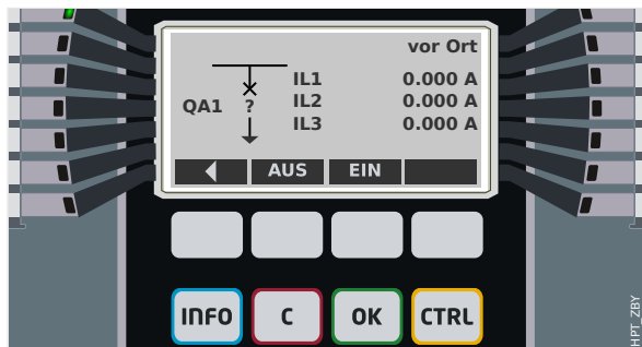
Abb. 118: Beispiel einer Steuer-Seite mit „Leistungsschalter“ in Störstellung (bzw. unplausiblem Zustand).
