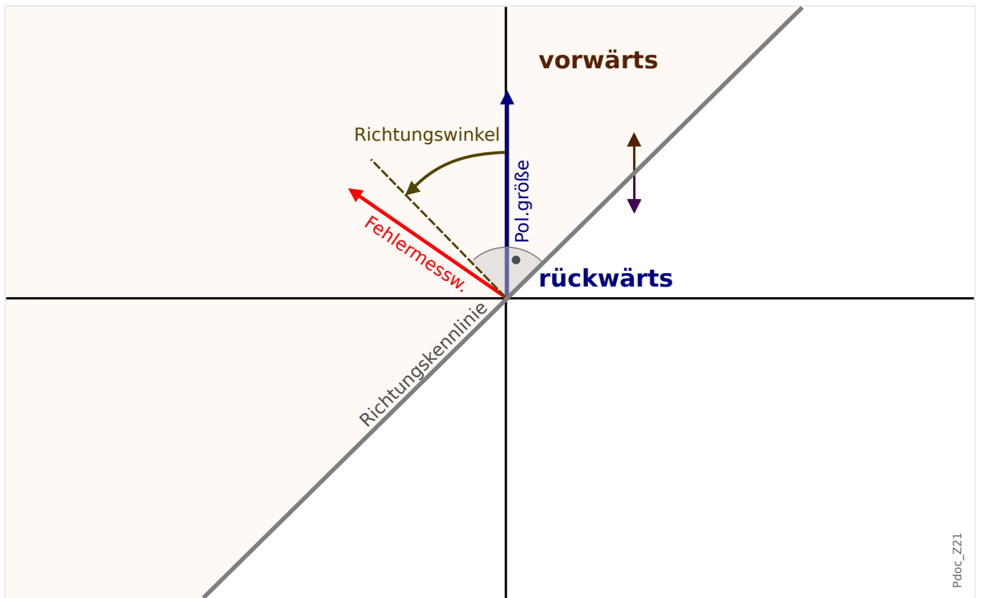
Abb. 61: Prinzip der Richtungserkennung von Phasenfehlern.
