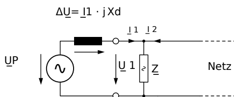
Abb. 82: Ersatzschaltbild netzparalleler Synchrongenerator
