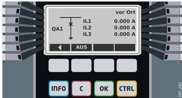
Abb. 117: Beispiel einer Steuer-Seite mit geschlossenem „Leistungsschalter“.
