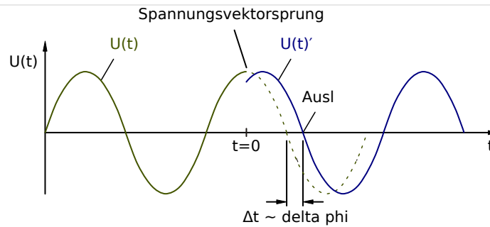
Abb. 86: Spannungsvektorsprung.
