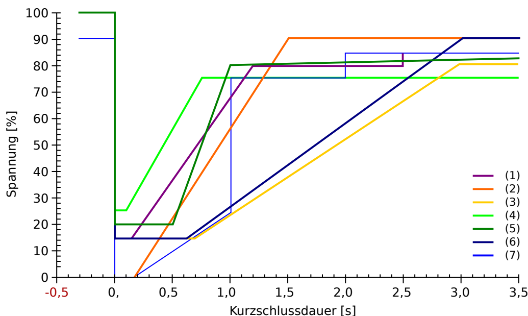
Abb. 75: Nationale LVRT-Standards, aus: eBWK Bd. 60 (2008) Nr. 4. Autoren: Dipl.-Ing. Thomas Smolka, Dr.-Ing. Karl-Heinz Weck, Zertifizierungstelle der FGH e.V., Mannheim, sowie Dipl.-Ing. (FH) Matthias Bartsch, Enercon GmbH, Aurich.
