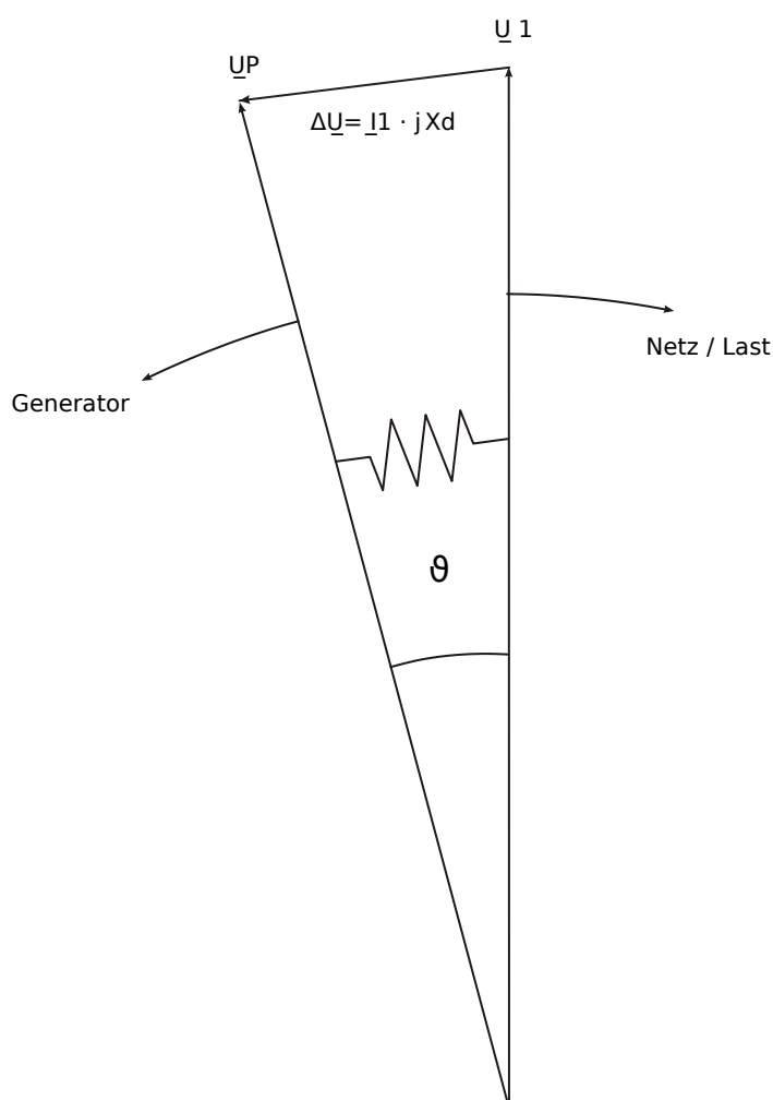
Abb. 83: Polradwinkel bei konstanter Belastung des Generators.
