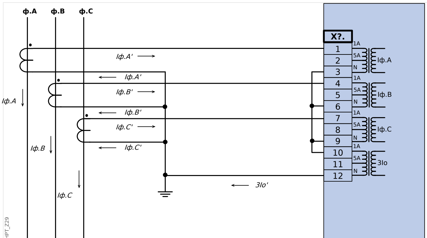
Рис. 22: Измерение фазных токов по схеме «полной» звезды; I_n вторичн. = 1 А. Ток на землю, измеряемый через соединение по схеме Холмгрин 3I_0 .ном.втор. = 1 А.
