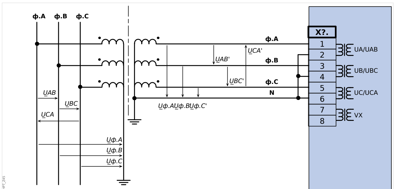
Рис. 30: VT Зуе: Измерение трехфазного напряжения по схеме «звезда»
