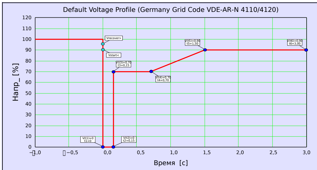
Рис. 88: Профиль LVRT по умолчанию (тип I).
