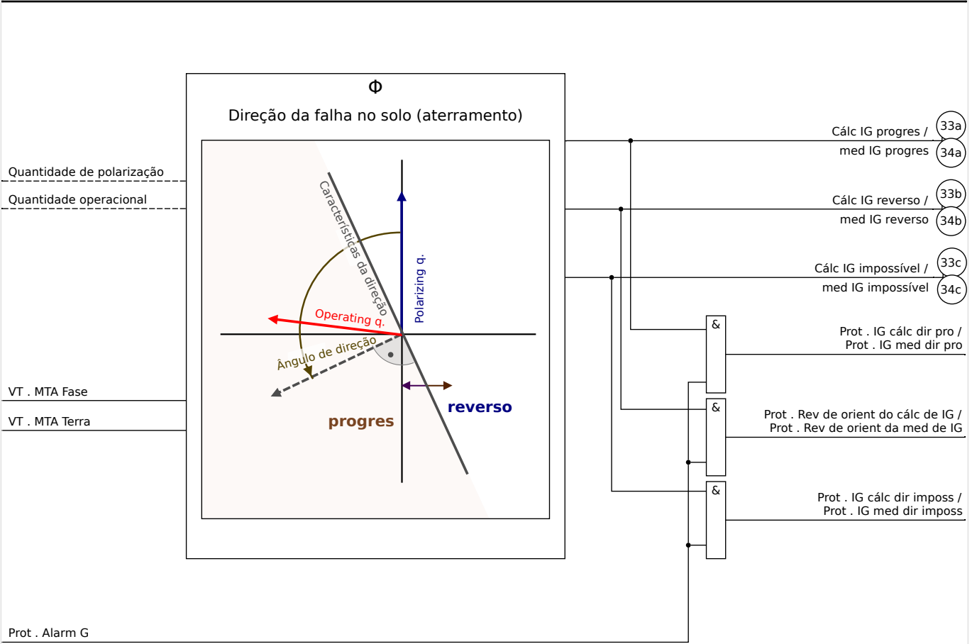
Fig. 65: Determinação da direção para todos os métodos, exceto "cos( \phi )", "sin( \phi )".
