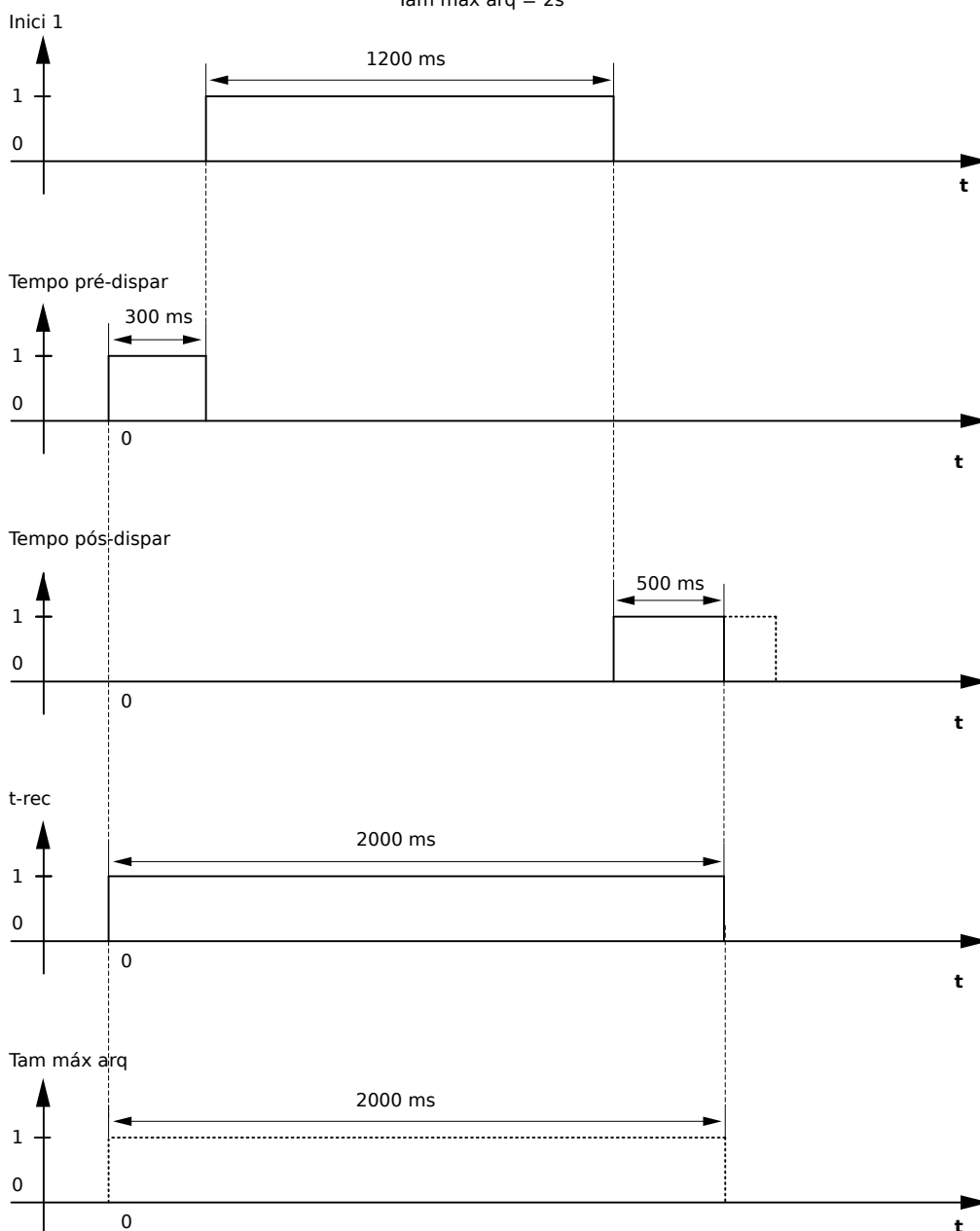
Fig. 135: Exemplo de Gráfico de Prazo do Gravador de Perturbação I
