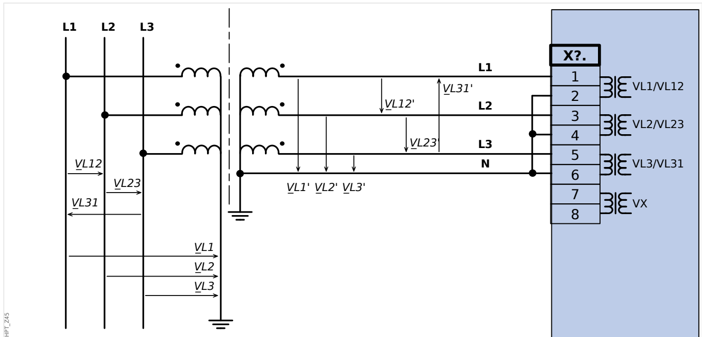
Fig. 30: VT Wye: Medição de voltagem trifásica - fiação das entradas de medição: "conexão estrela"
