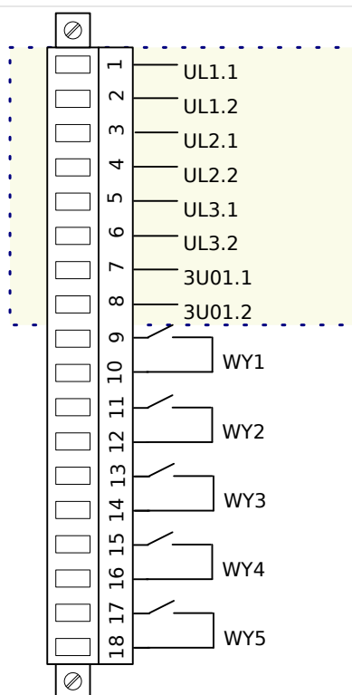
Rys. 29: Przepisanie elektromechaniczne
