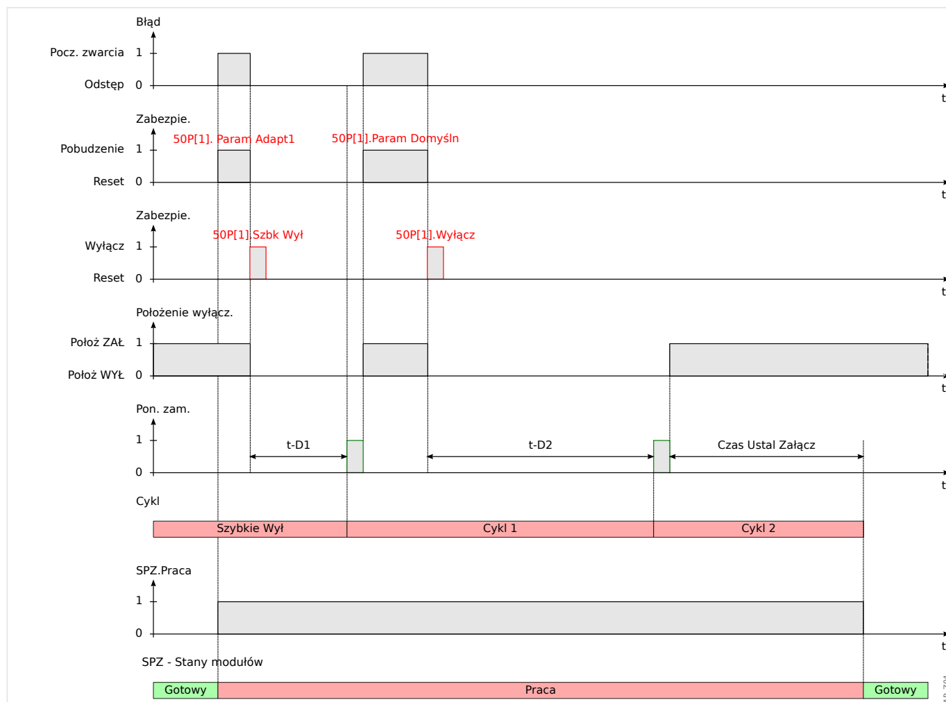
Rys. 112: Schemat czasów SPZ w przypadku udanego planu SPZ z 2 próbami i przyspieszeniem przy próbie wstępnej
