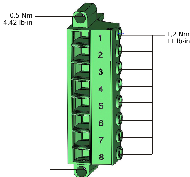
Rys. 146: Zaciski pomiaru napięcia karty pomiarowej „TU” (↳ „3.6.1 TU – wejścia do pomiaru napięcia”).
