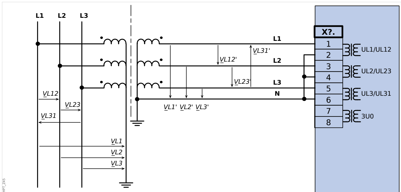
Rys. 30: Przekładnik napięciowy połączony w gwiazdę: Trójfazowy pomiar napięcia w układzie gwiazdy
