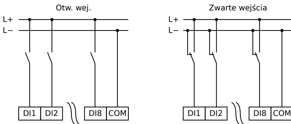
Rys. 148: Stan bezpieczny wejść dwustanowych
