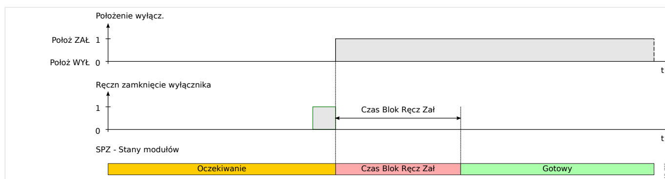
Rys. 113: Stany SPZ podczas ręcznego zamykania wyłącznika.
