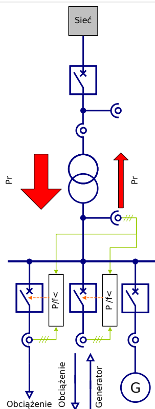
Rys. 104: Zdecentralizowane podczęstotliwościowe zmniejszanie obciążenia w sieciach z tymczasowym zasilaniem.
