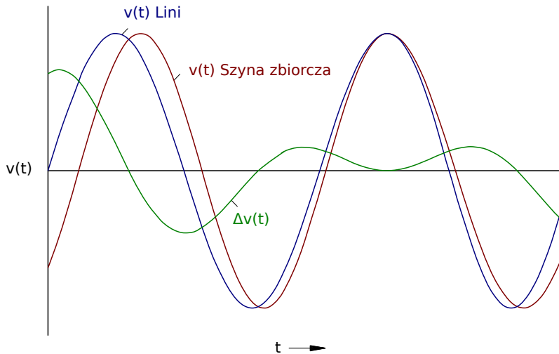
Rys. 118: Krzywa napięciowa ze zwiększoną rozdzielczością.
