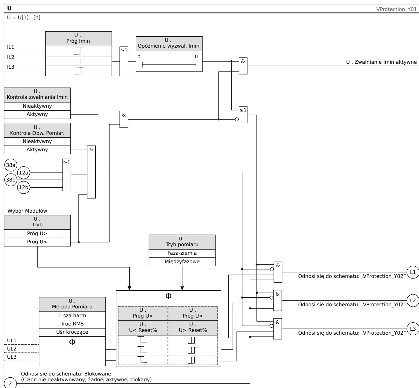
Rys. 82: Działanie modułu zabezpieczenia napięciowego, część 1.
