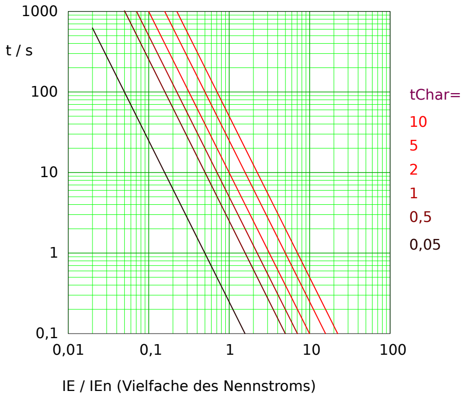
Abb. 93: Auslösekurve „I2T“, wobei nur der Bereich IE > I_{E>} jeweils anwendbar ist. Beispieldiagramm für gemessenen (nicht empfindlichen) Erdstrom.
