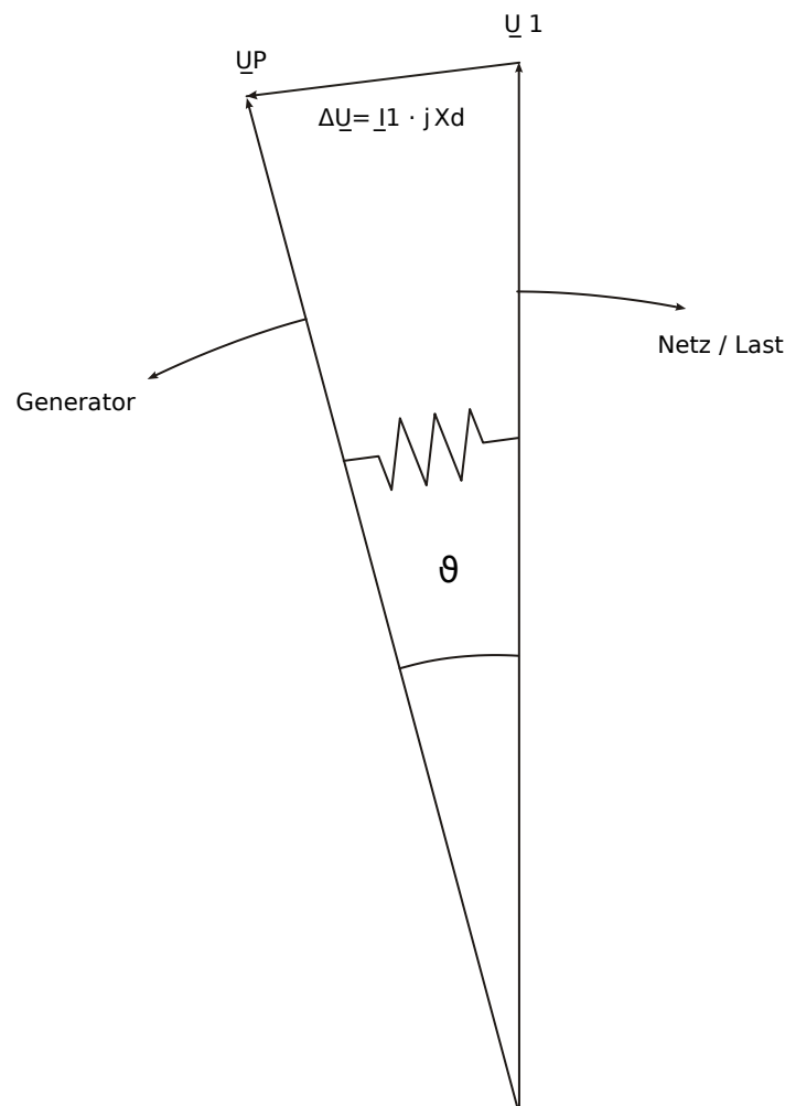
Abb. 109: Polradwinkel bei konstanter Belastung des Generators.
