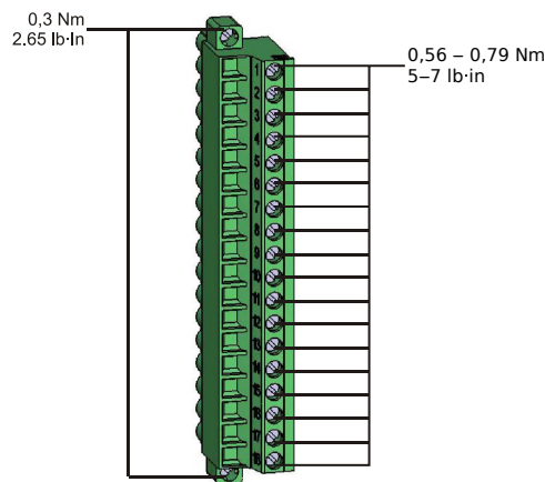
Abb. 165: Spannungsmessstecker der Spannungsmesskarten „TU-OR5“ und „TU-DI8“.
