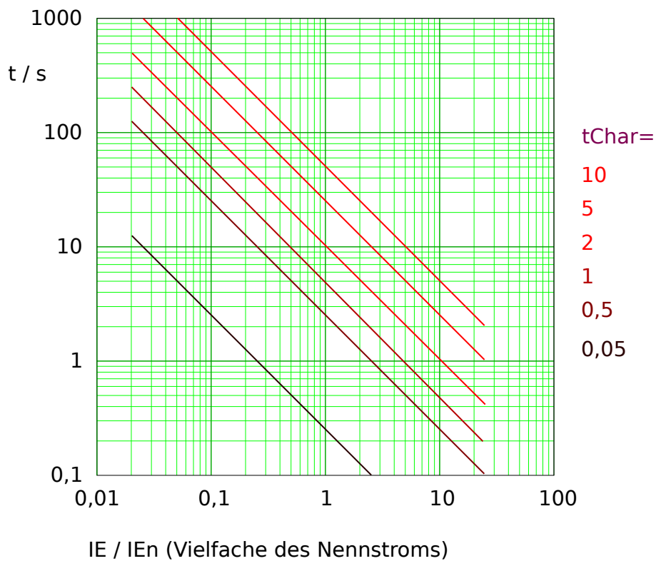
Abb. 92: Auslösekurve „IT“, wobei nur der Bereich IE > I_{E>} jeweils anwendbar ist. Beispieldiagramm für gemessenen (nicht empfindlichen) Erdstrom.
