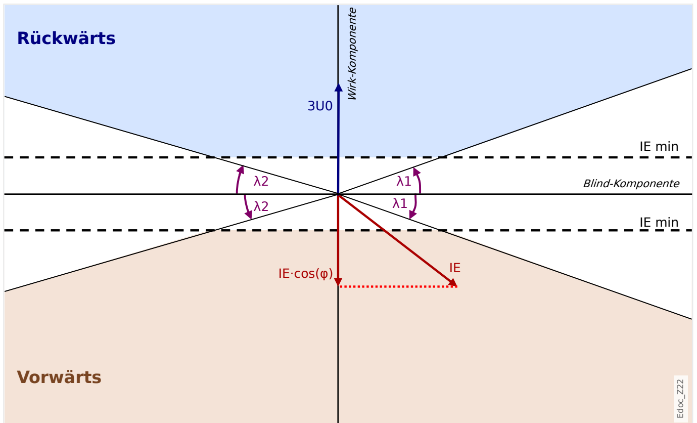
Abb. 65: Richtungserkennung nach der Methode „ \cos(\phi) “.
