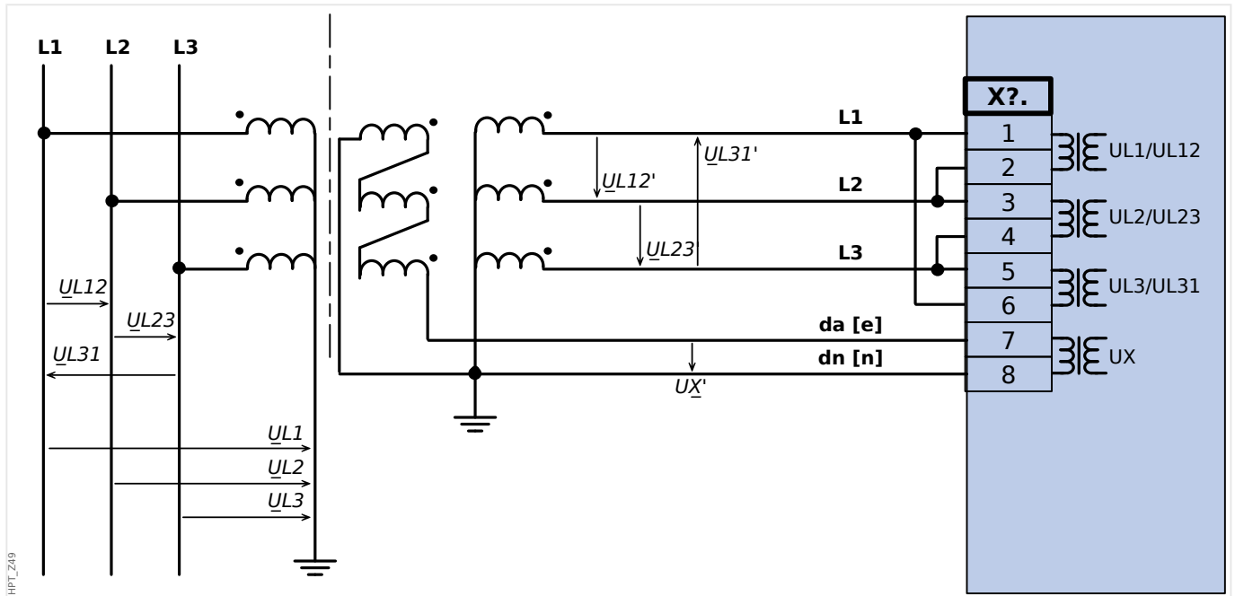
Abb. 33: Drei Spannungswandler mit Geräteanschluss in Dreieckschaltung Erfassung der Verlagerungsspannung UE mit offener Dreieckschaltung e-n
