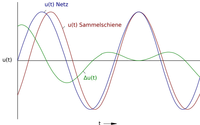
Abb. 135: Spannungsverlauf der Schwebespannung \Delta u(t) , vergrößert.
