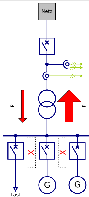
Abb. 123: Dezentraler Einsatz in Teilnetzen mit überwiegender Rückspeisung.
