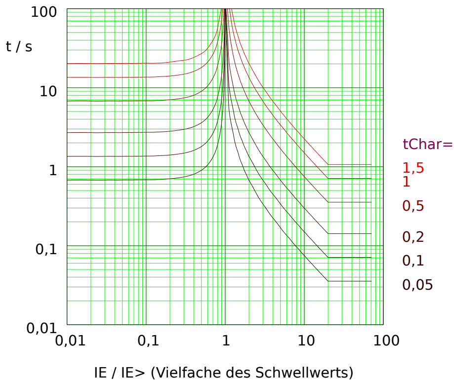
Abb. 83: VINV: Rückfallverzögerung (linke Hälfte, IE < I_{E>} ) und Auslöseverzögerung (rechte Hälfte, IE > I_{E>} ), Beispieldiagramm für I_{max} = 20 \cdot I_{E>} .
