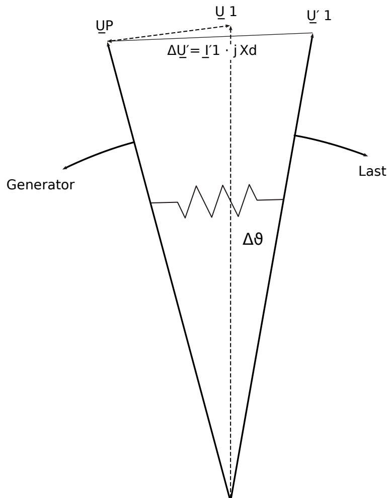
Abb. 111: Änderung des Polradwinkels bei plötzlicher Belastung des Generators.
