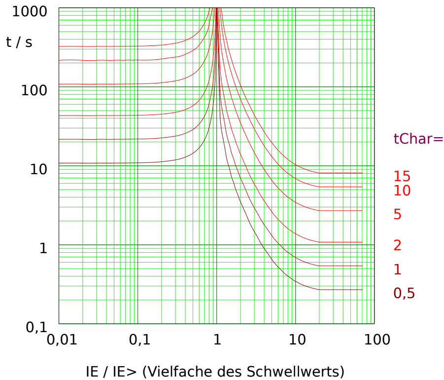
Abb. 88: VINV: Rückfallverzögerung (linke Hälfte, IE < I_{E>} ) und Auslöseverzögerung (rechte Hälfte, IE > I_{E>} ), Beispieldiagramm für I_{max} = 20 \cdot I_{E>} .
