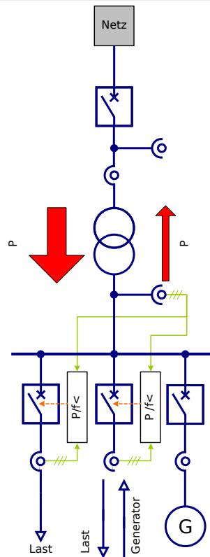
Abb. 121: Dezentrale Automatische Frequenzentlastung in Netzen mit zeitweiser Rückspeisung.
