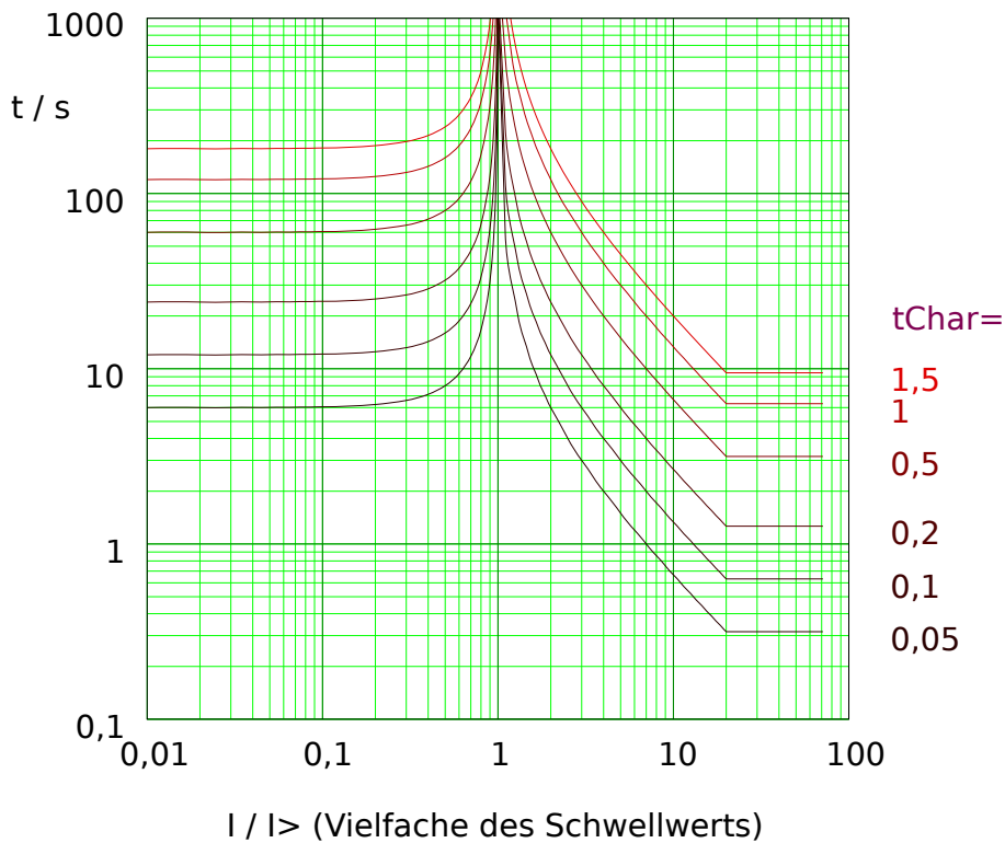
Abb. 73: LINV: Rückfallverzögerung (linke Hälfte, I < I_{>} ) und Auslöseverzögerung (rechte Hälfte, I > I_{>} ), Beispieldiagramm für I_{max} = 20 \cdot I_{>} .
