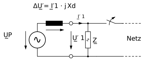
Abb. 110: Ersatzschaltbild Synchrongenerator bei Netzausfall.
