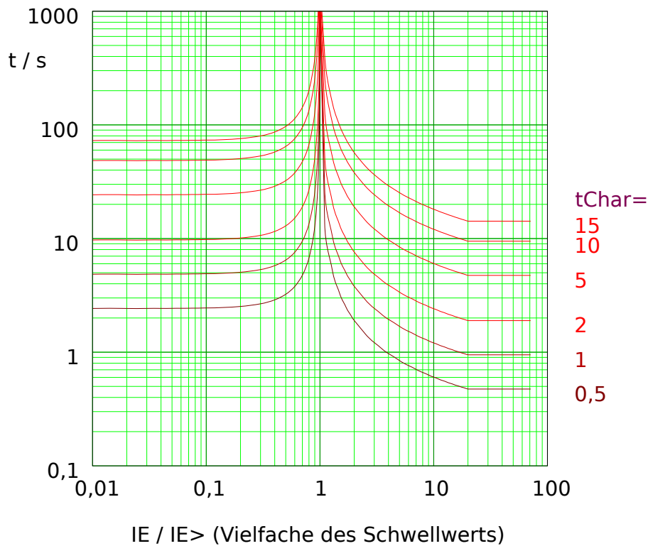
Abb. 87: MINV: Rückfallverzögerung (linke Hälfte, IE < I_{E>} ) und Auslöseverzögerung (rechte Hälfte, IE > I_{E>} ), Beispieldiagramm für I_{max} = 20 \cdot I_{E>} .
