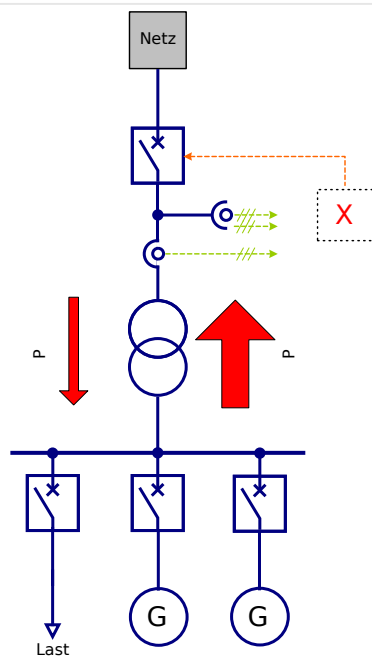
Abb. 122: Zentraler Einsatz in Teilnetzen mit überwiegender Rückspeisung.
