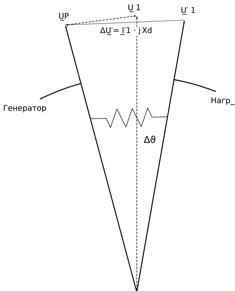
Рис. 86: Векторы напряжения при сбое электросети.
