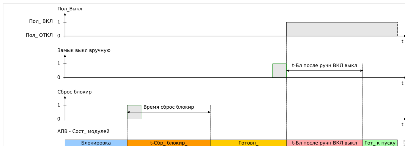
Рис. 106: Логика сброса блокировки АПВ при получении команды сброса блокировки перед замыканием выключателя вручную.
