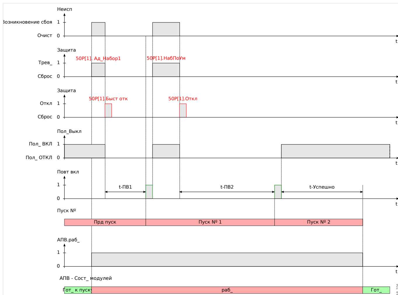
Рис. 103: Диаграмма синхронизации автоматического повторного включения для схемы с 2 удачными попытками автоматического повторного включения и ускорением перед импульсом.
