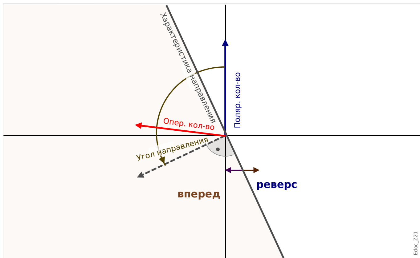
Рис. 63: Принцип определения направления для всех методов, кроме « \cos(\phi) » и « \sin(\phi) ».
