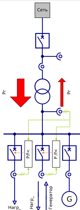
Рис. 95: Децентрализованная автоматическая частотная разгрузка в сетях с временным электроснабжением.
