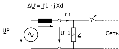
Рис. 85: Эквивалентная цепь при сбое электросети.
