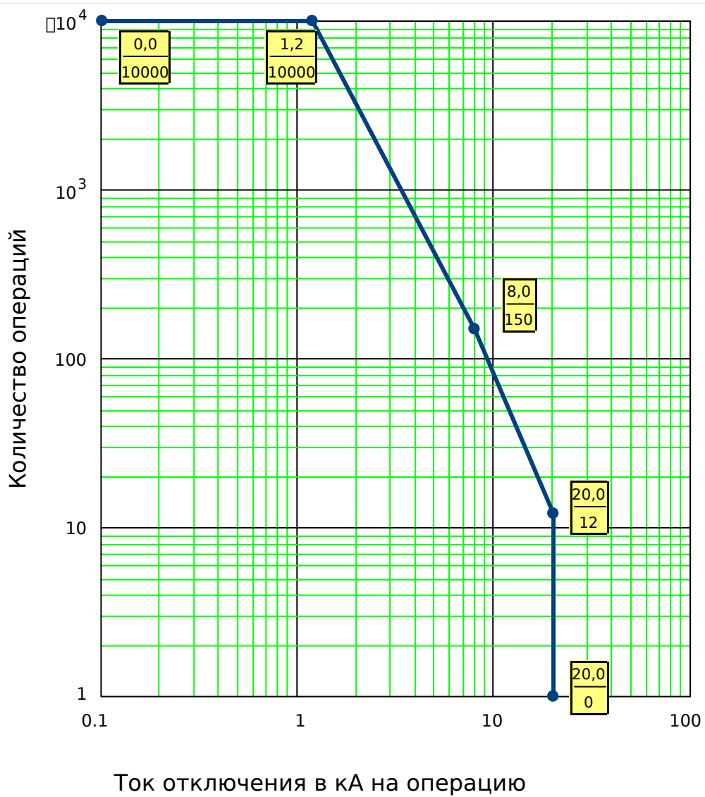
Рис. 123: Эксплуатационная кривая выключателя для типичного выключателя 25кВ
