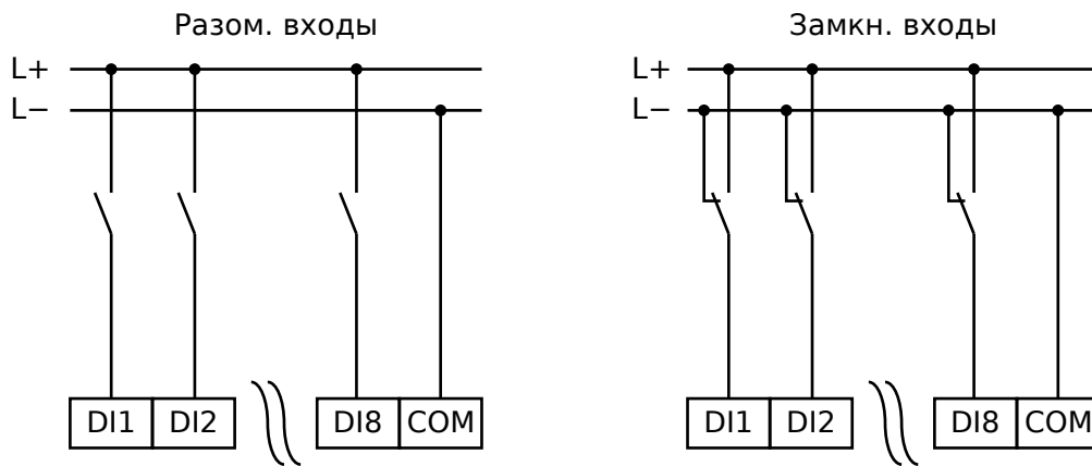
Рис. 141: Безопасное состояние цифровых входов
