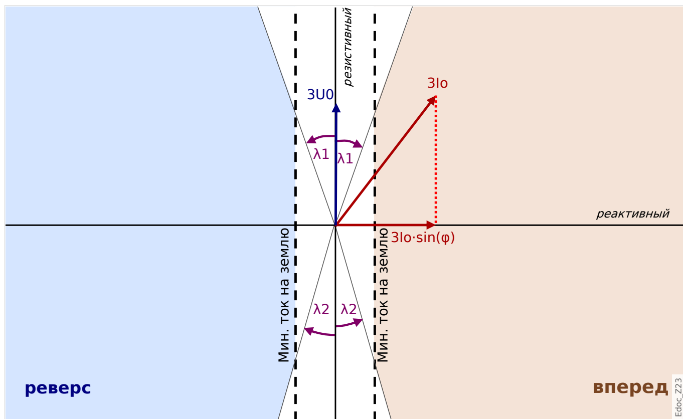
Рис. 66: Принцип определения направления для метода « \sin(\phi) ».
