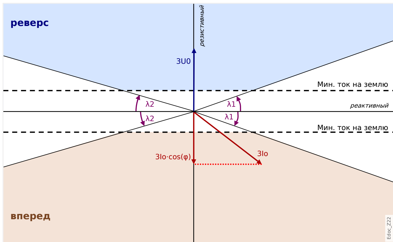
Рис. 65: Принцип определения направления для метода « \cos(\phi) ».
