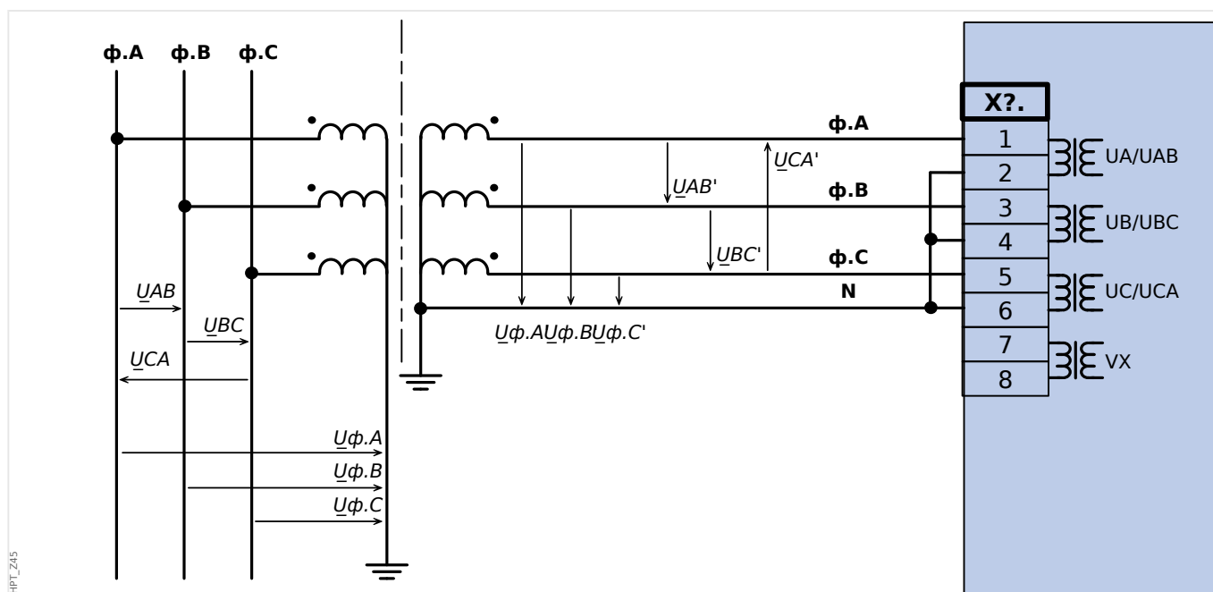
Рис. 30: VT Wye: Измерение трехфазного напряжения по схеме «звезда»
