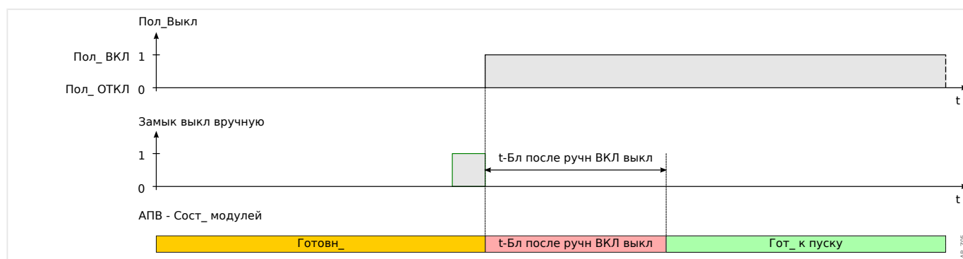
Рис. 104: Состояния автоматического повторного включения во время замыкания выключателя вручную.
