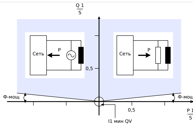
Рис. 90: Метод 1: контроль угла мощности.
