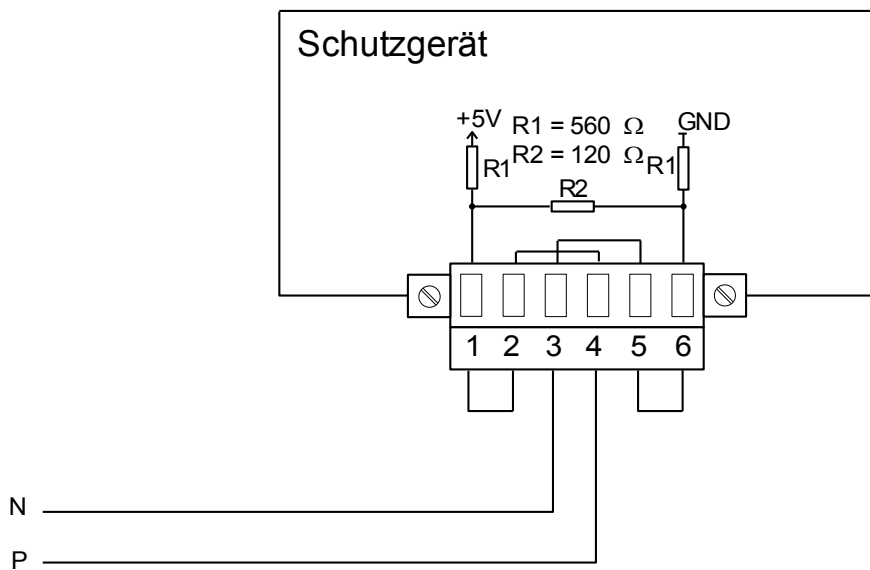
Typ 1 Verdrahtungsbeispiel, Gerät am Ende des Busses (Benutzen des integrierten Abschlusswiderstands)
