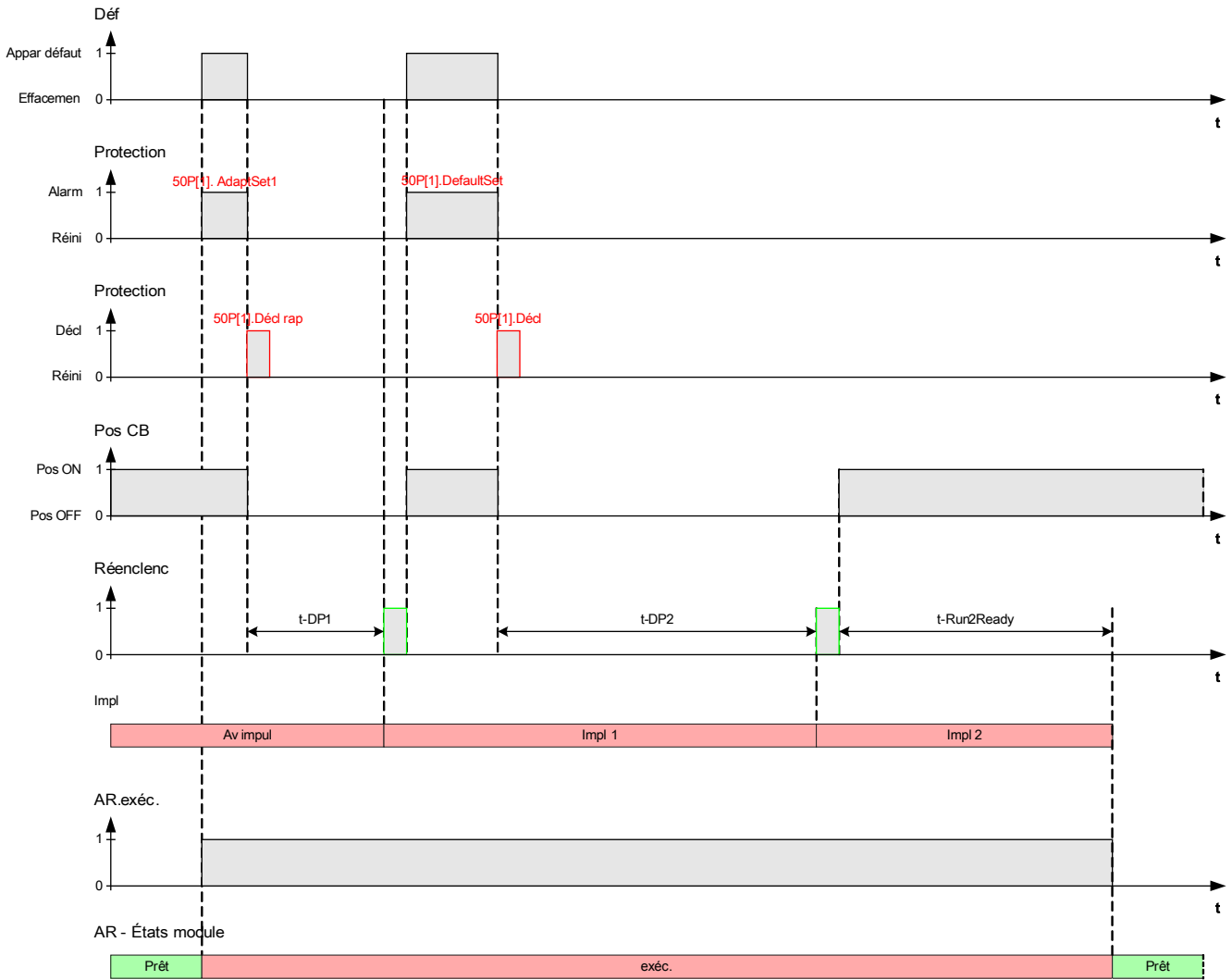
Diagramme de temporisation de réenclenchement automatique pour un schéma de réenclenchement automatique à 2 impulsions réussi avec une accélération à la pré-impulsion
