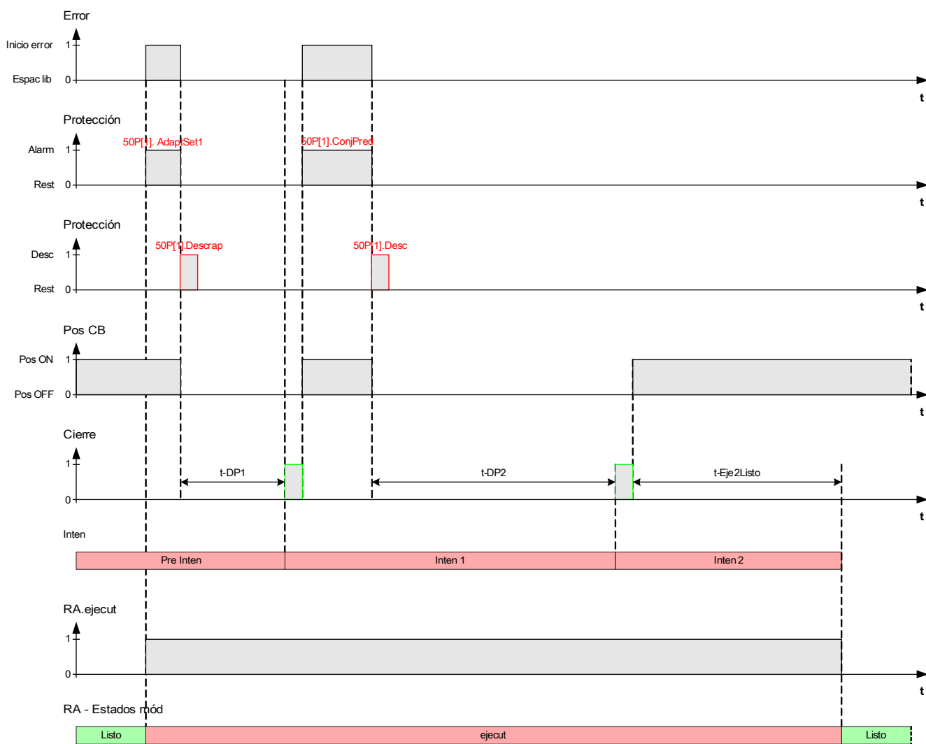
Diagrama de tiempo de reconexión automática para el esquema de reconexión automática de 2 intentos correcta con aceleración en intento previo
