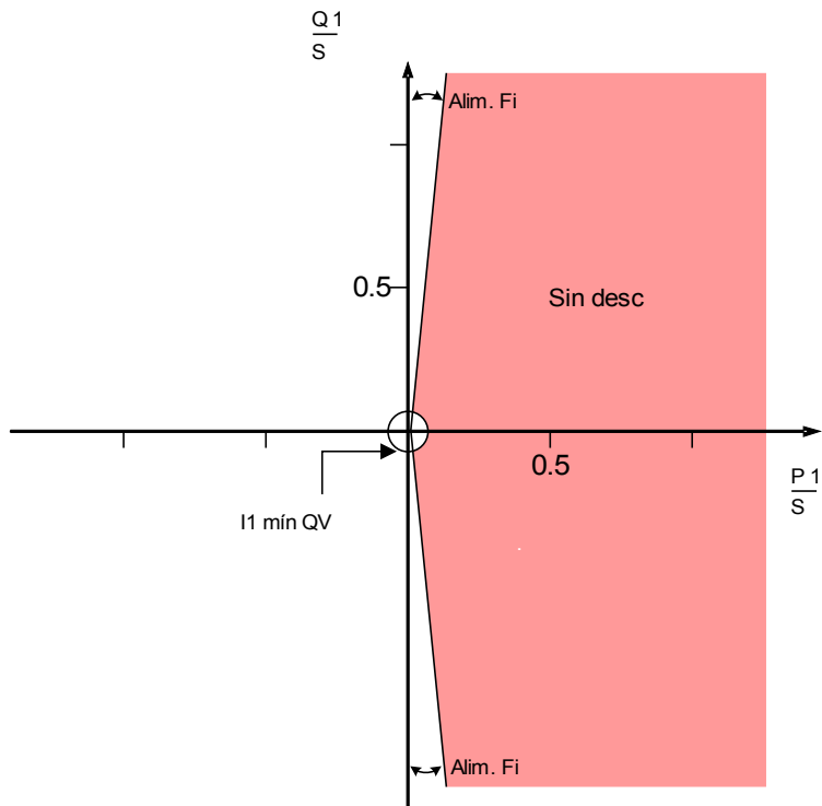
Método UFLS = Superv. Ángulo Potencia
