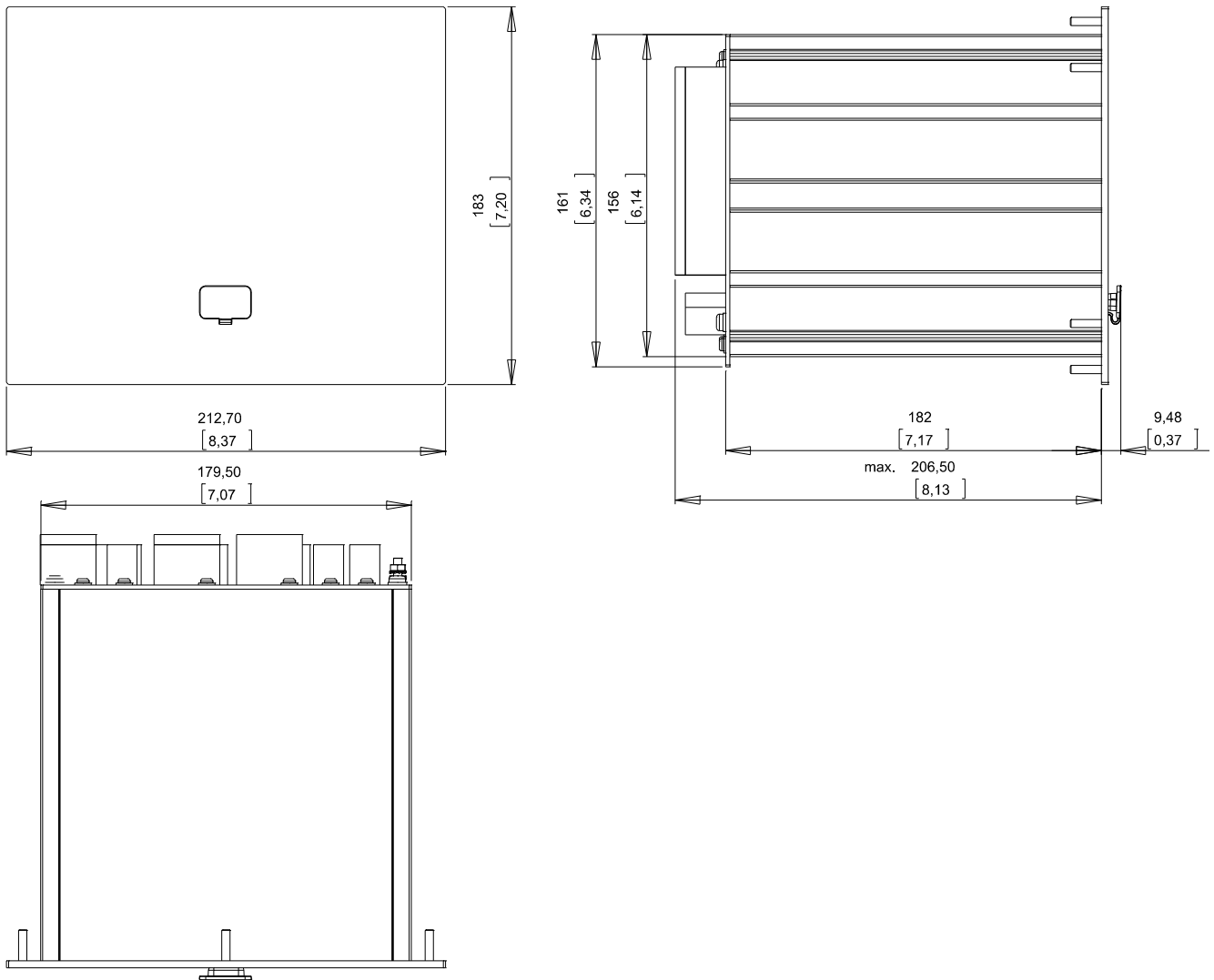
Vista de 3 lados, carcasa B2 (dispositivos con 8 teclas)
