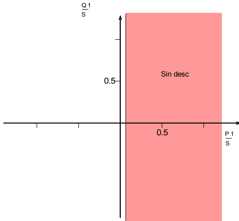
Método UFLS = Superv. de potencia activa pura
