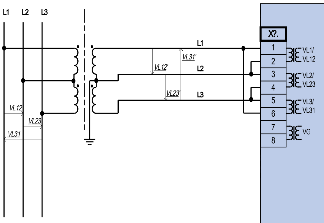
Medida voltaje bifásico: cableado de las entradas de medida: "Abr. Delta"
