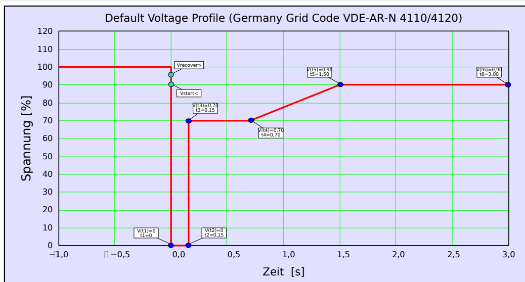
Abb. 105: LVRT-Werkseinstellung (Typ I).
