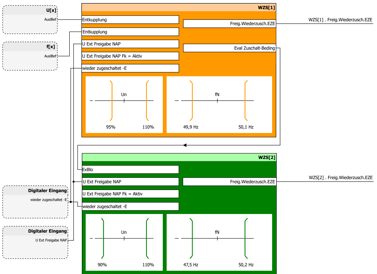
Abb. 119: Applikationsbeispiel für ein (Wieder-)Zuschalten in Abhängigkeit von einer vorherigen Auslösung des Entkuppungsschutzes.
