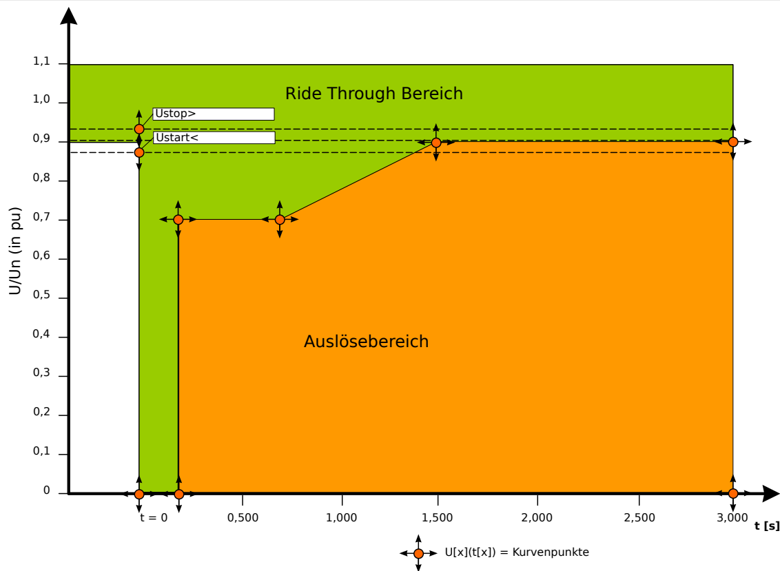
Abb. 104: Spannungs-Zeit-Profil und Auslösebereich.
