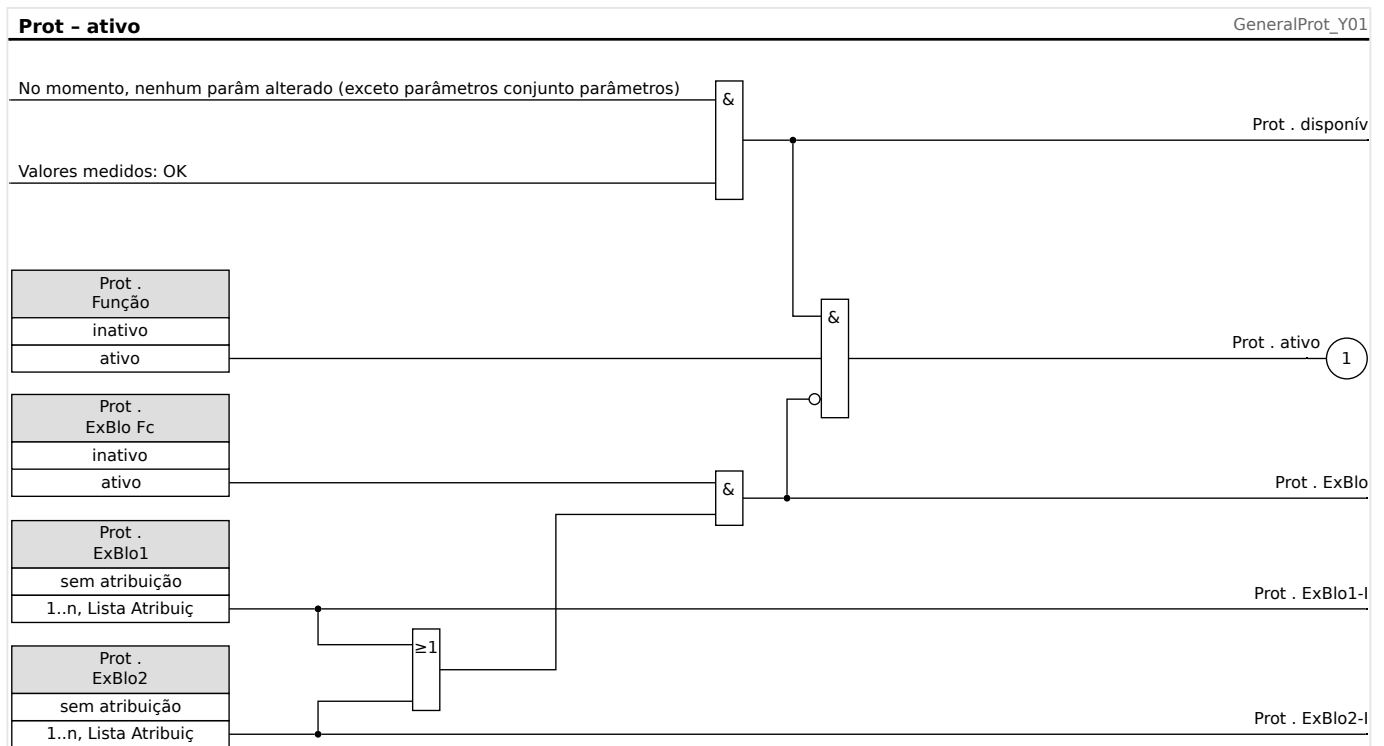
Fig. 60: Disponibilidade do módulo de proteção geral.
