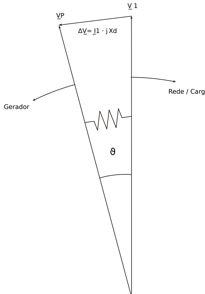
Fig. 93: Vetores de tensão em operação paralela.
