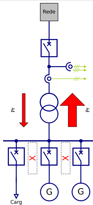
Fig. 106: Uso descentralizado em redes com fonte de alimentação predominante.
