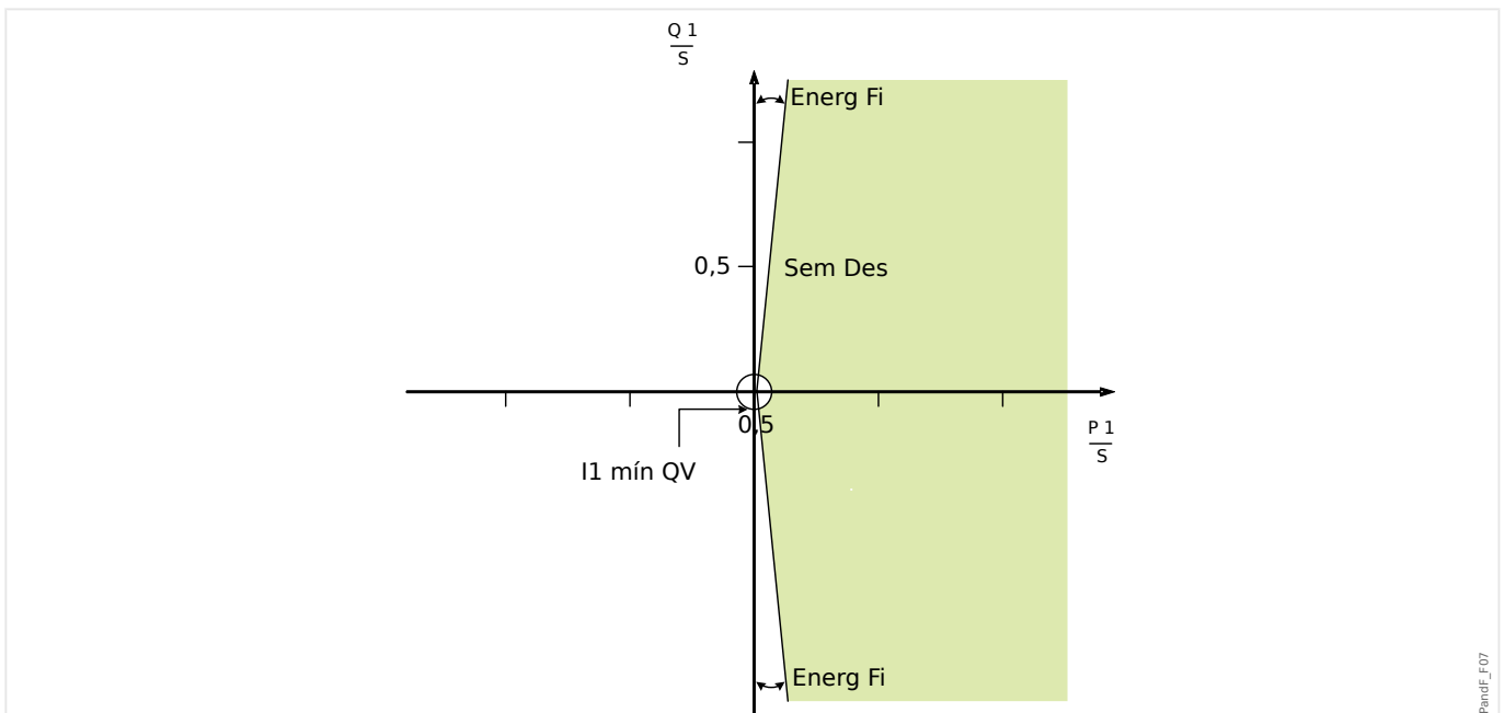
Fig. 107: Método 1 (Supervisão de Ângulo de Energia): “Método UFLS” = “Supervisão Âng Energ”.
