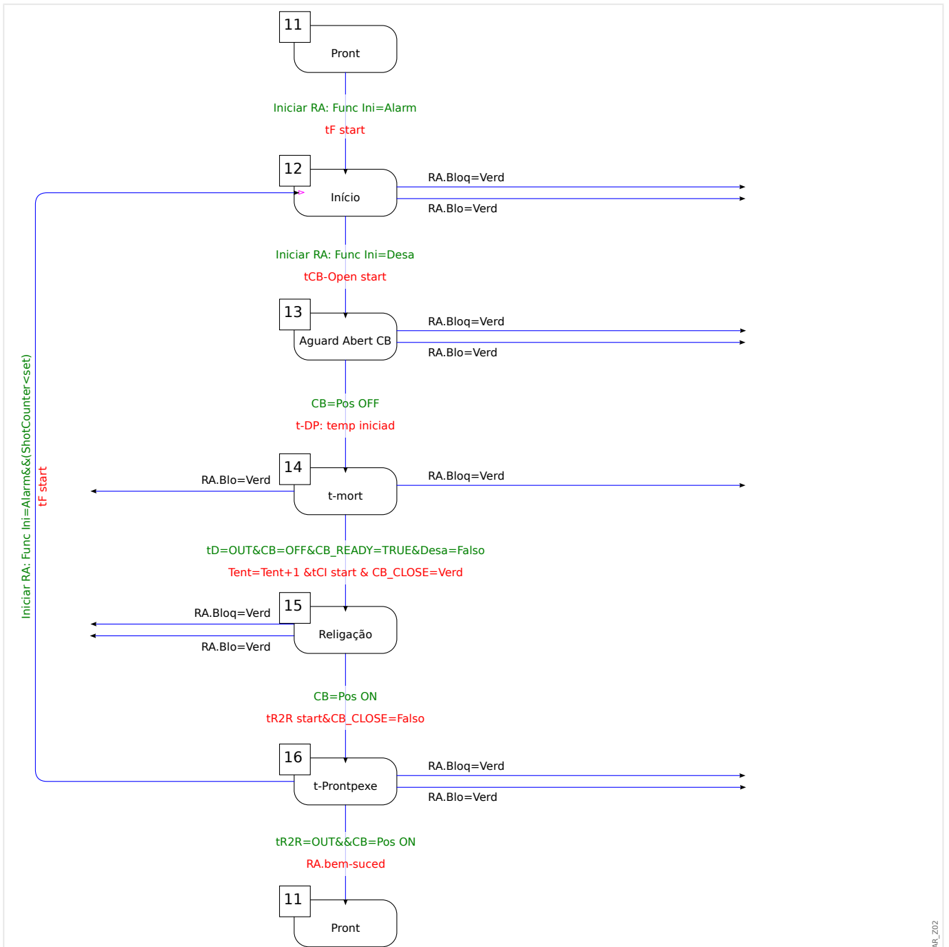
Fig. 110: Ciclo de execução de RA (estado 4).
