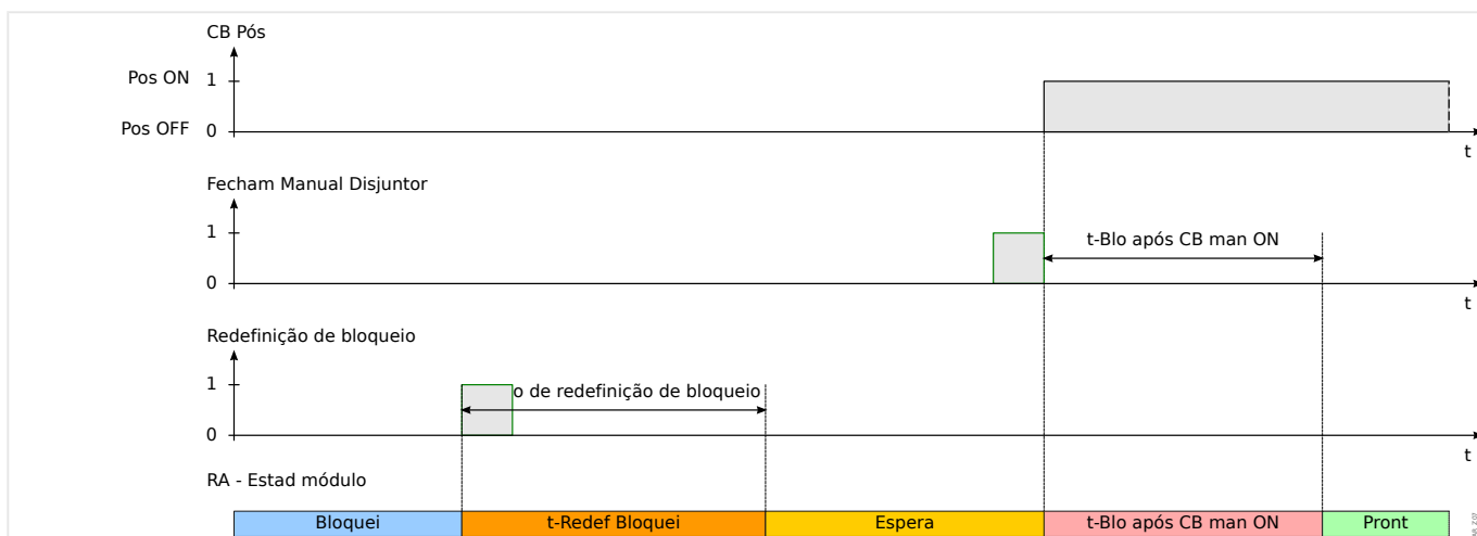
Fig. 115: A lógica de reinicialização de travamento no caso do reinício do travamento vir antes do fechamento manual do disjuntor
