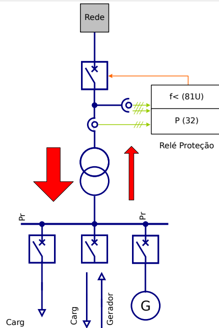
Fig. 103: Derramamento de carga de subfrequência centralizada em redes com fornecimento temporário de energia.
