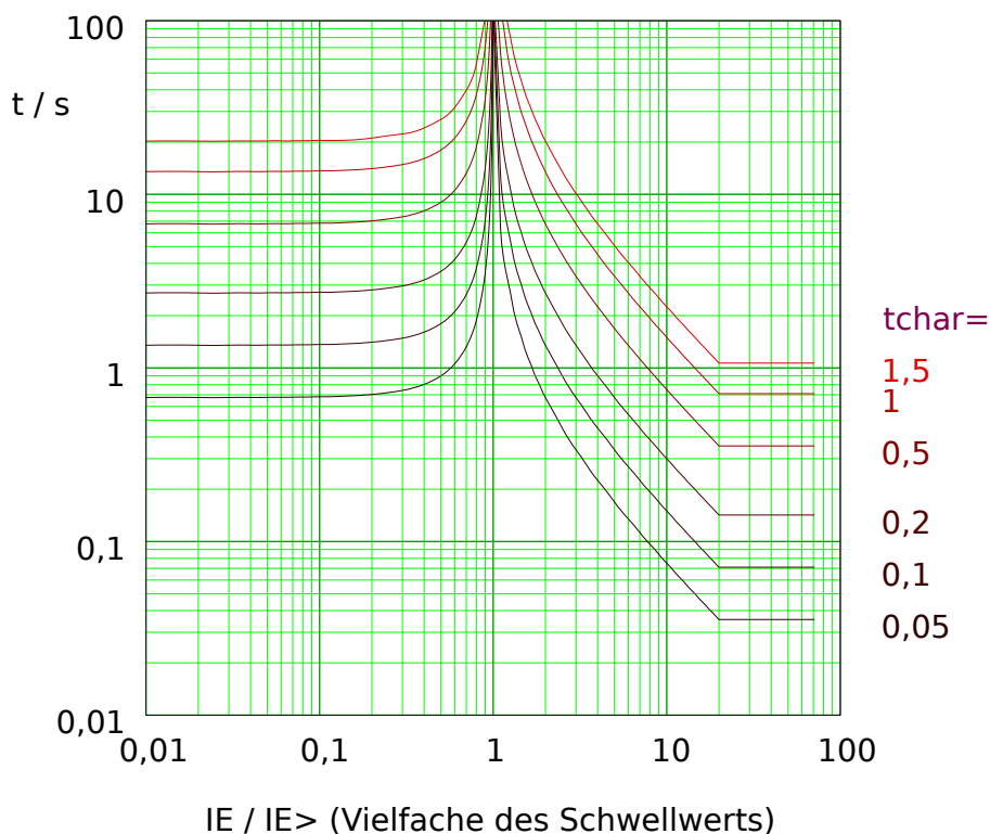
Abb. 83: VINV: Rückfallverzögerung (linke Hälfte, IE < IE> ) und Auslöseverzögerung (rechte Hälfte, IE > IE> ), Beispieldiagramm für I_{E,max} = 20 \cdot IE> .
