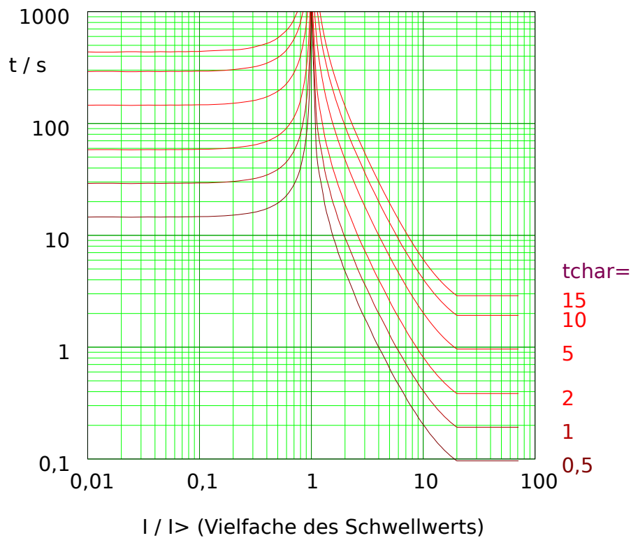
Abb. 76: EINV: Rückfallverzögerung (linke Hälfte, I < I> ) und Auslöseverzögerung (rechte Hälfte, I > I> ), Beispieldiagramm für I_{max} = 20 \cdot I> .
