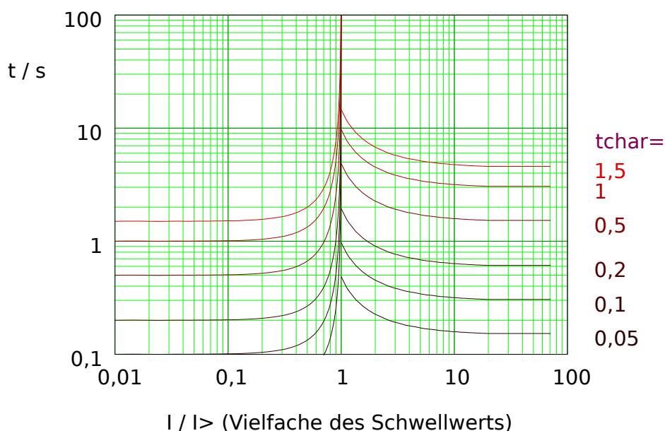
Abb. 77: RINV: Rückfallverzögerung (linke Hälfte, I < I_{max} ) und Auslöseverzögerung (rechte Hälfte, I > I_{max} ), Beispieldiagramm für I_{max} = 20 \cdot I_{nom} .
