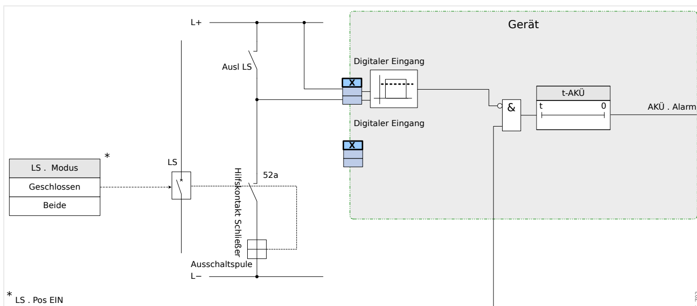
Abb. 141: Anschlussbeispiel: Auslösekreisüberwachung mit einem Hilfskontakt »Hiko EIN« (52a).
