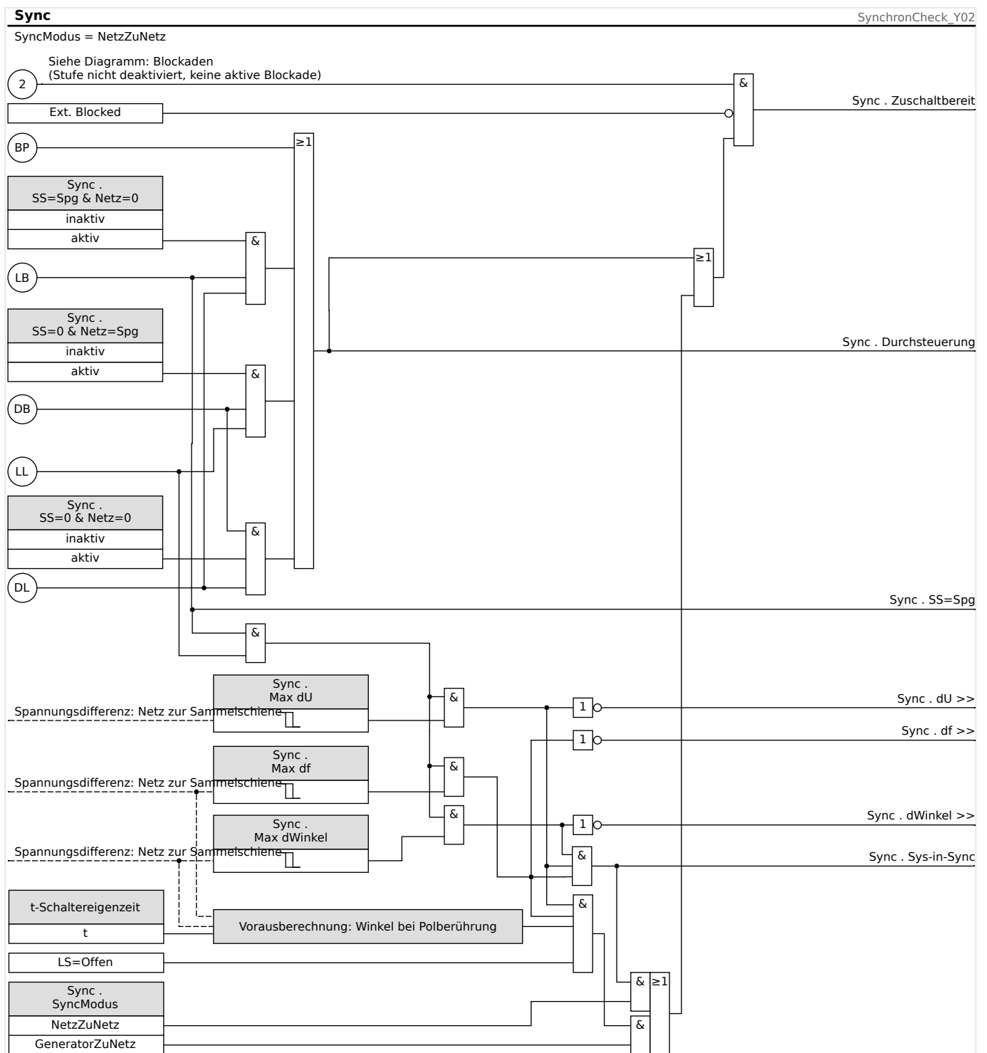
Abb. 137: Funktionalität des »Sync«-Moduls, „NetzZuNetz“.
