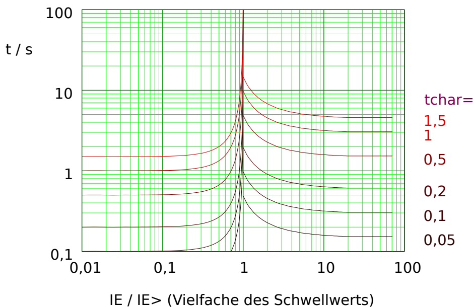
Abb. 89: RINV: Rückfallverzögerung (linke Hälfte, IE < IE> ) und Auslöseverzögerung (rechte Hälfte, IE > IE> ), Beispieldiagramm für I_{E,max} = 20 \cdot IE> .
