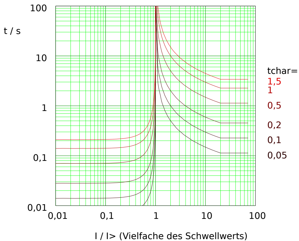
Abb. 70: NINV: Rückfallverzögerung (linke Hälfte, I < I_n ) und Auslöseverzögerung (rechte Hälfte, I > I_n ), Beispieldiagramm für I_{max} = 20 \cdot I_n .
