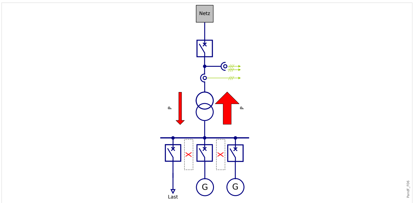
Abb. 123: Dezentraler Einsatz in Teilnetzen mit überwiegender Rückspeisung.
