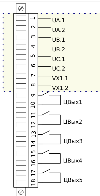
Рис. 29: Электромеханическая адресация
