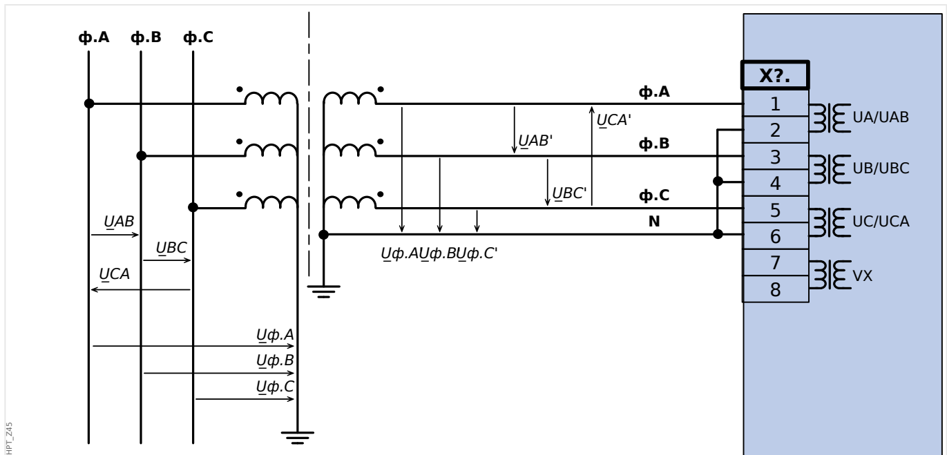
Рис. 30: VT Wye: Измерение трехфазного напряжения по схеме «звезда»
