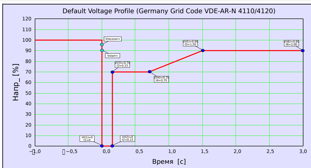
Рис. 80: Профиль LVRT по умолчанию (тип I).
