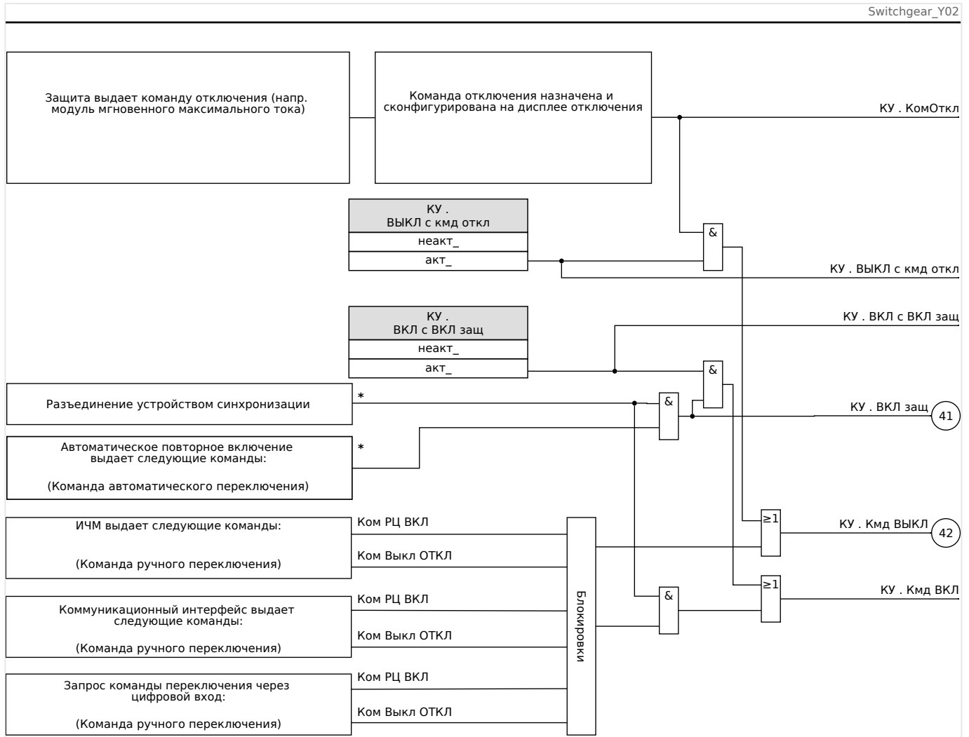
Рис. 122: Блокировки. (Детали, отмеченные «*»: наличие зависит от заказанного типа устройства.)
