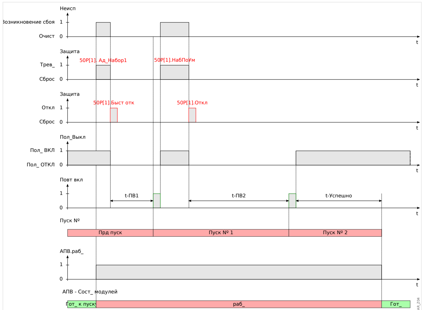
Рис. 104: Диаграмма синхронизации автоматического повторного включения для схемы с 2 успешными попытками автоматического повторного включения и ускорением перед импульсом.
