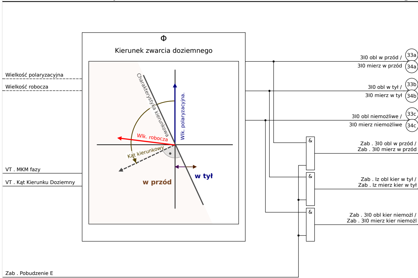
Rys. 65: Zasada określania kierunku obowiązująca dla wszystkich metod z wyjątkiem „cos( \phi )”, „sin( \phi )”.
