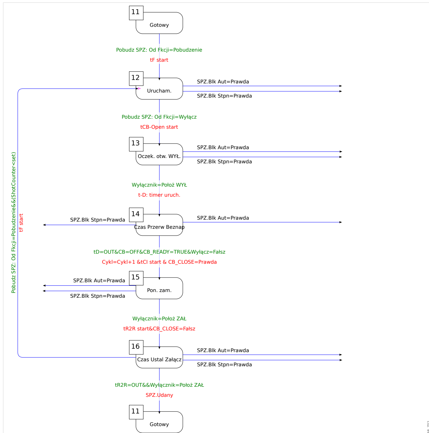
Rys. 102: Cykl pracy SPZ (stan 4).
