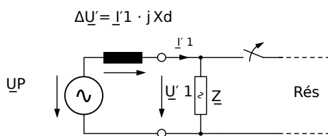
Fig. 86: Circuit équivalent en cas de coupure de réseau.
