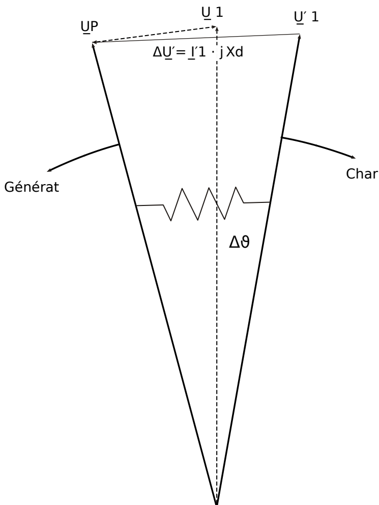
Fig. 87: Vecteurs de tension en cas de coupure de réseau.
