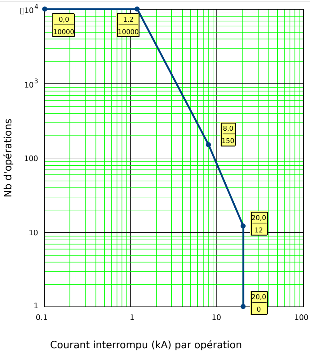
Fig. 124: Courbe de maintenance du disj pour un disj 25 ~kV typique
