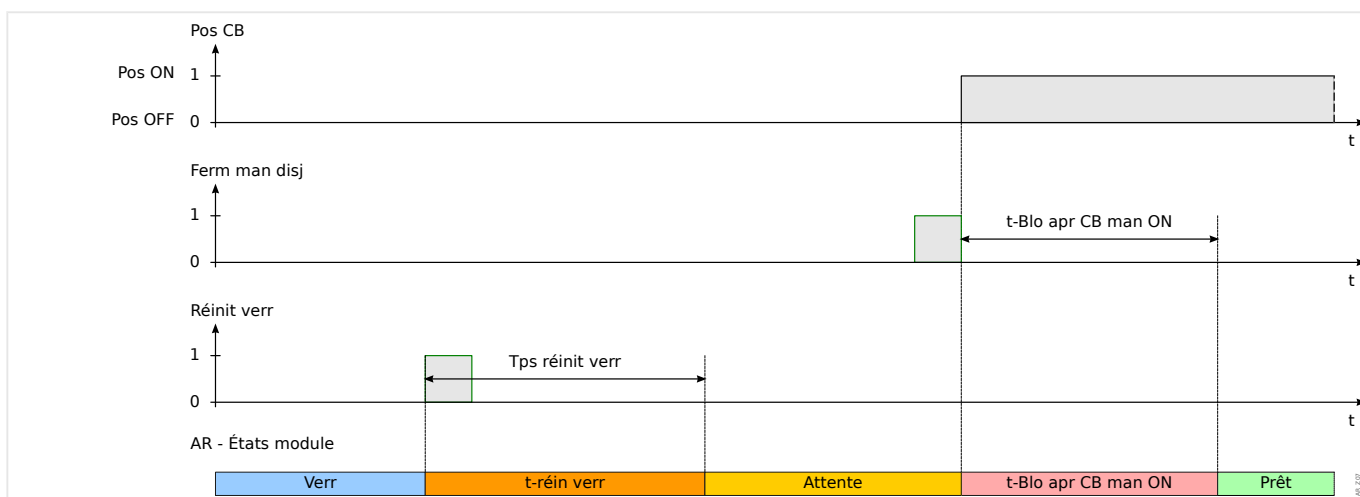
Fig. 107: Logique de réinitialisation du verrouillage du réenclenchement automatique si la réinitialisation du verrouillage se produit avant la fermeture du disjoncteur manuelle.
