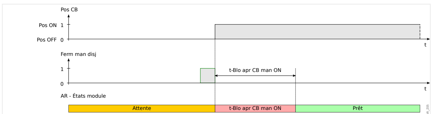
Fig. 105: États du réenclenchement automatique pendant la fermeture manuelle du disjoncteur.
