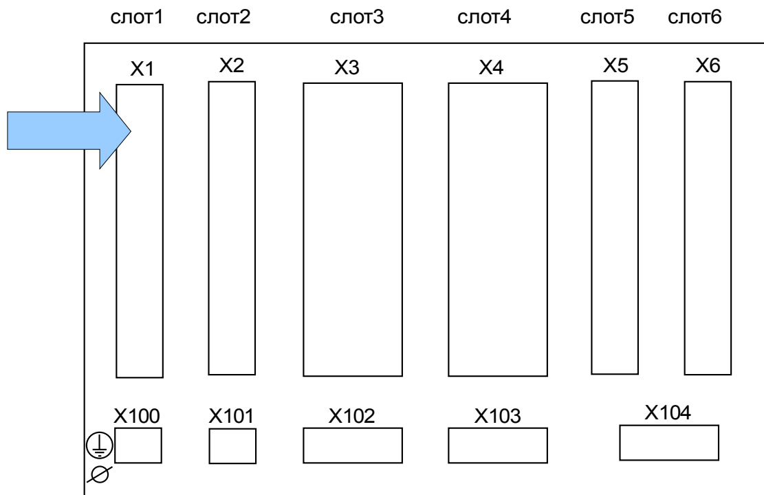
Задняя сторона устройства (слоты)
