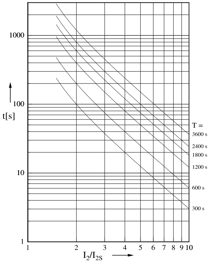
Abbildung 7.1: Auslösekennlinie
