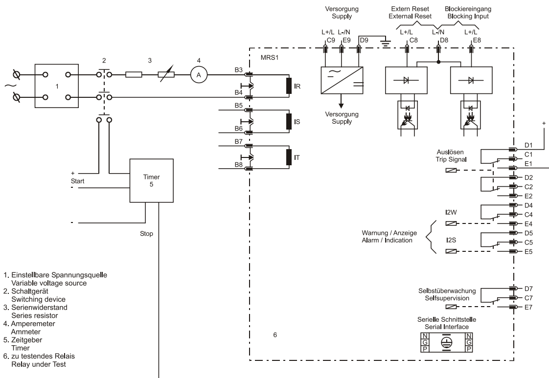
Abbildung 6.1: Testschaltung
