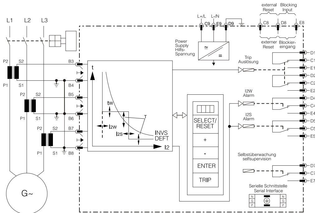
Abbildung 3.1: Anschlussbild
